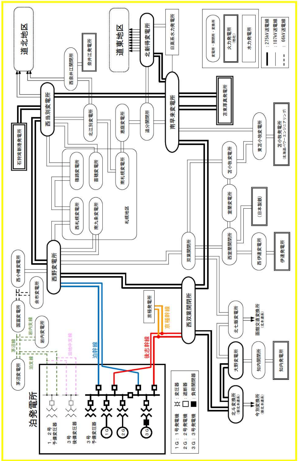
第 10.3.1 図 送電系統概要図
