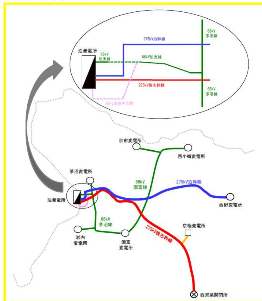
第 2.2.3.1 図 送電線ルート
