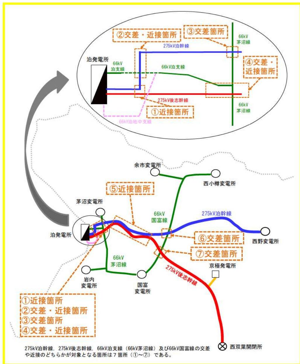
第 2.2.3.2 図 送電線の交差・近接箇所
