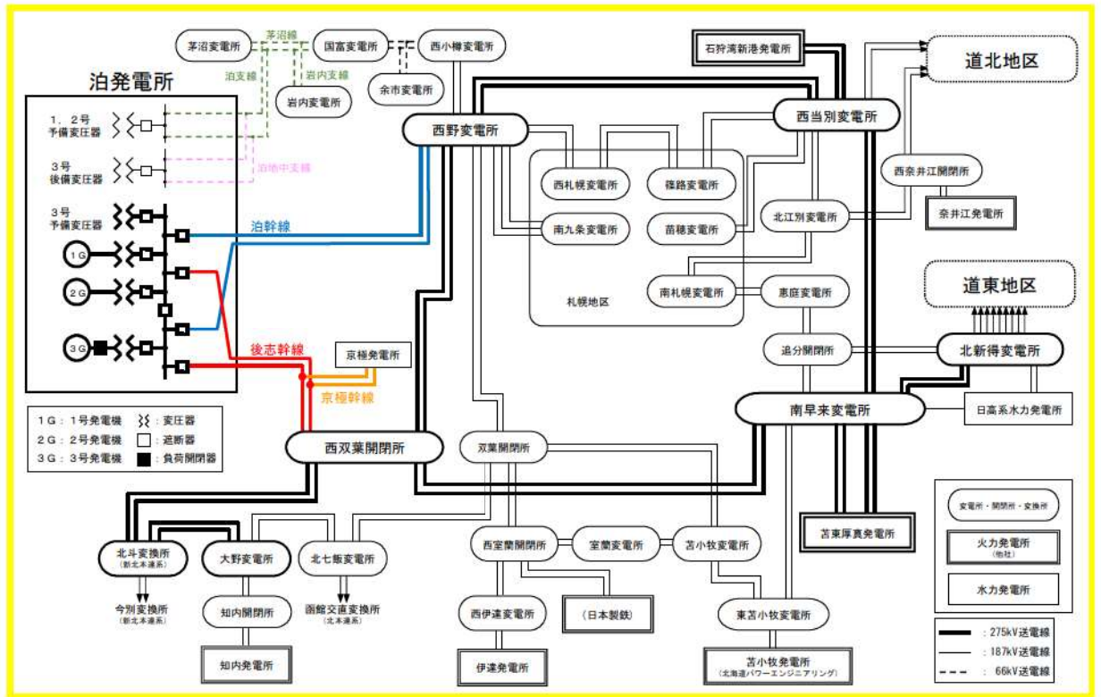
第 2.1.1.1 図 送電系統図
