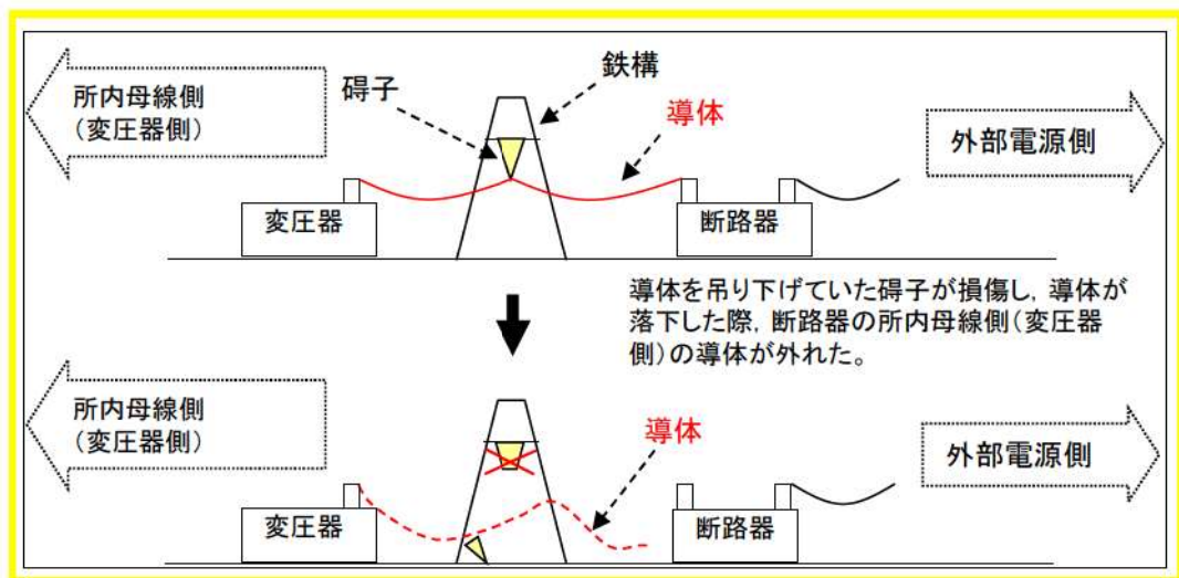
第2.2.1.8図 米国バイロン2号炉の1相開放故障の概要
