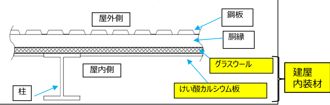
【使用済燃料貯蔵施設の上層部の壁断面概略図】
