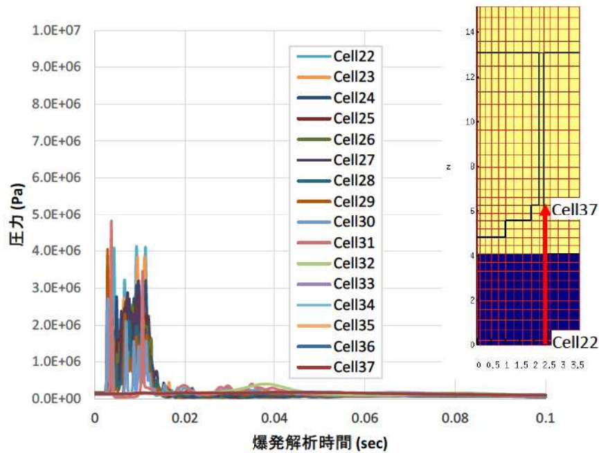
図2 原子炉下部キャビティ側面の圧力履歴
