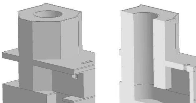
図2 LS-DYNA解析モデル図（原子炉下部キャビティ）
