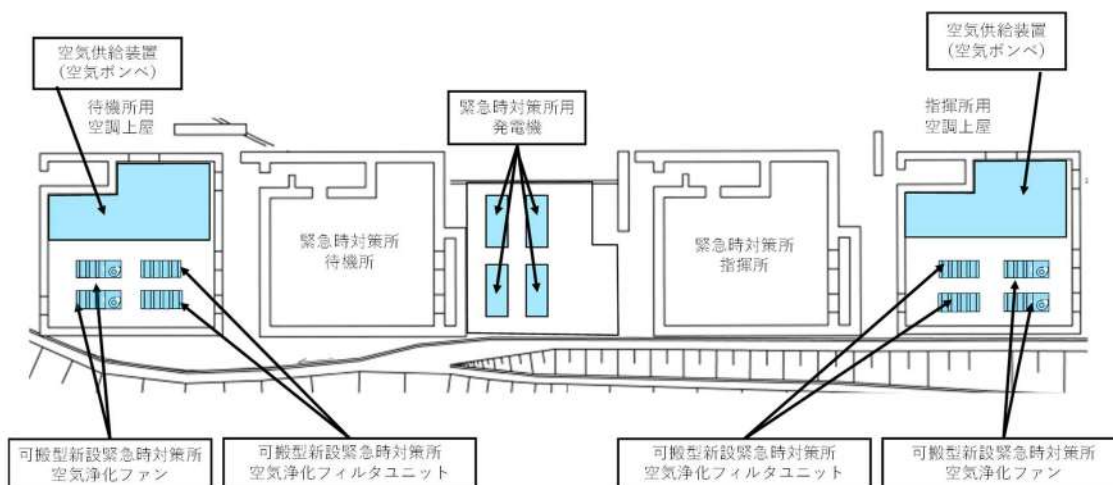
第1.18.5図 可搬型可搬型新設緊急時対策所空気浄化ファン，可搬型新設緊急 時対策所空気浄化フィルタユニット，空気供給装置（空気ボンベ）設置場所
