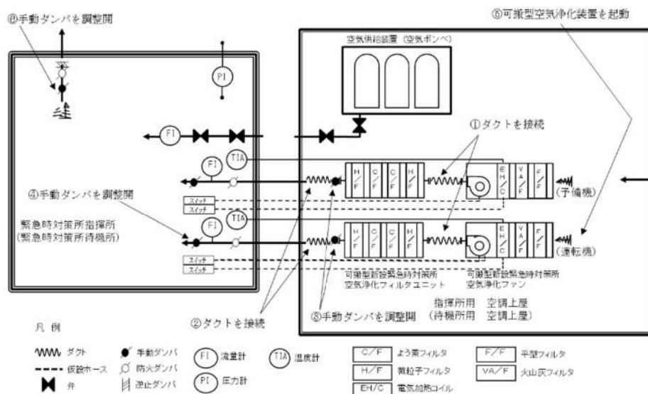
1.18.19 図 可搬型空気浄化装置運転概要図
