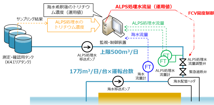
図 1.1.5-10 希釈率（ALPS 処理水流量）の評価式
