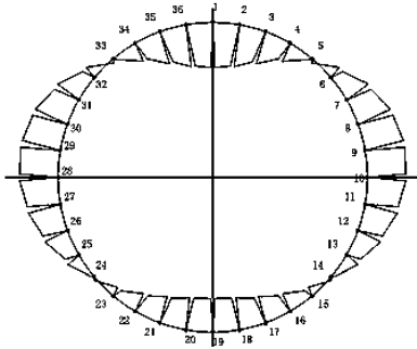
図 2.14.1.1-26 曲げモーメント図
