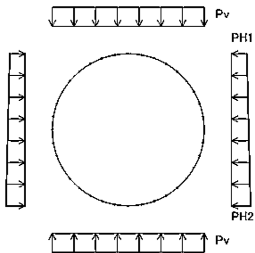
図 2.14.1.1-17 外荷重
