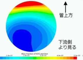
図-5 海水配管での混合希釈の評価結果
