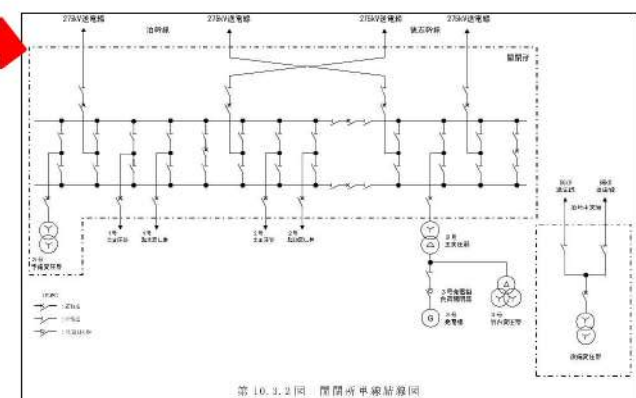
【系統概要図】開閉所単線結線図
