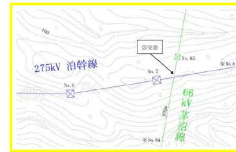
第2.2.3.5図 ③交差箇所の現地状況 (3/3)
