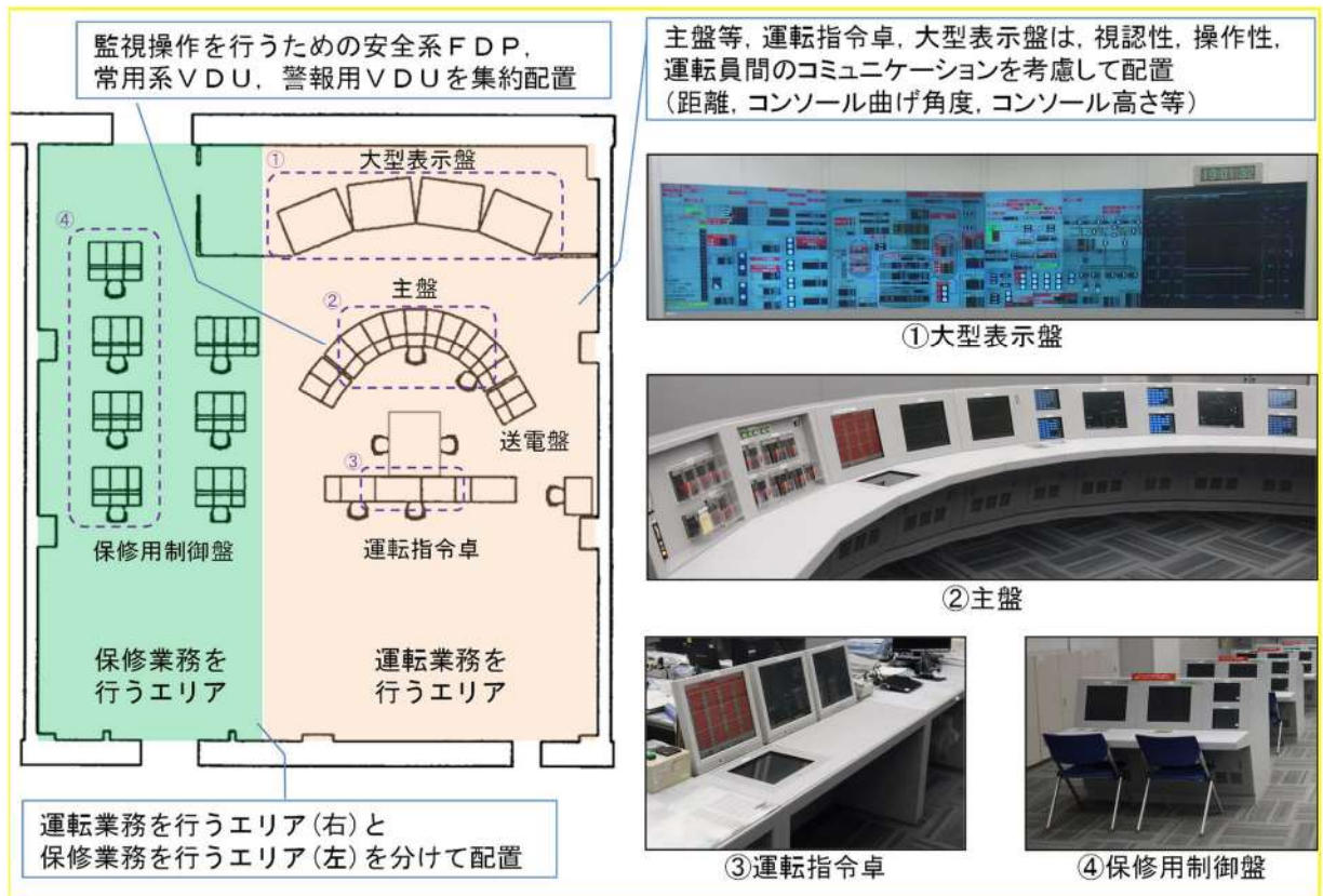
図 2.5.1.2 中央制御室内の盘面配置
