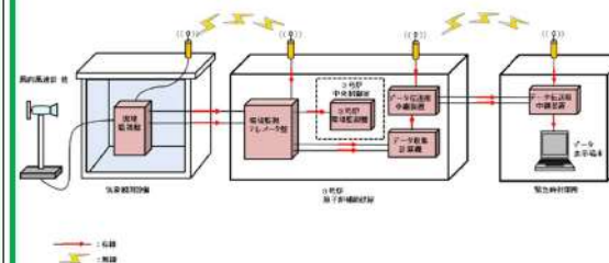
第2.1-2図 気象観測設備の伝送概略図
