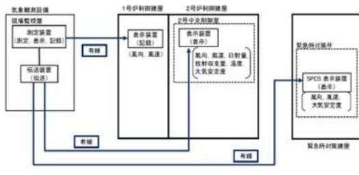
第2.1-2図 気象観測設備の伝送概略図
