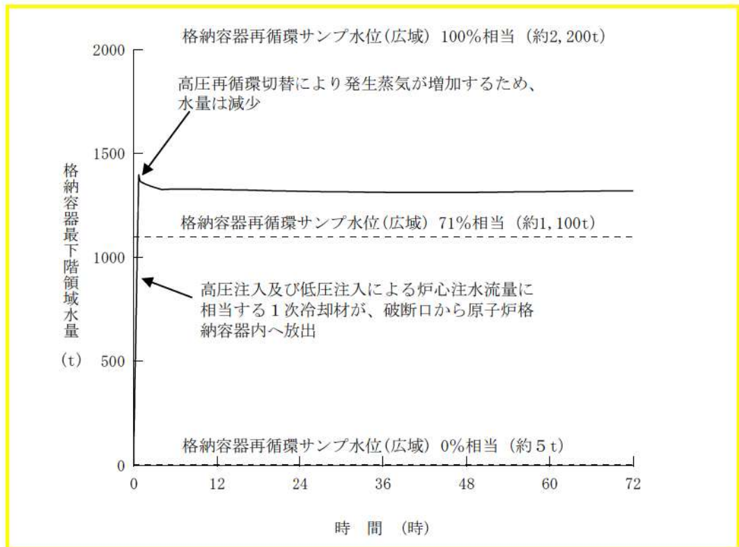
第 7.1.4.10 図 格納容器最下階領域水量の推移
