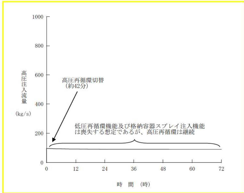
第 7. 1. 4. 6 図 高圧注入流量の推移
