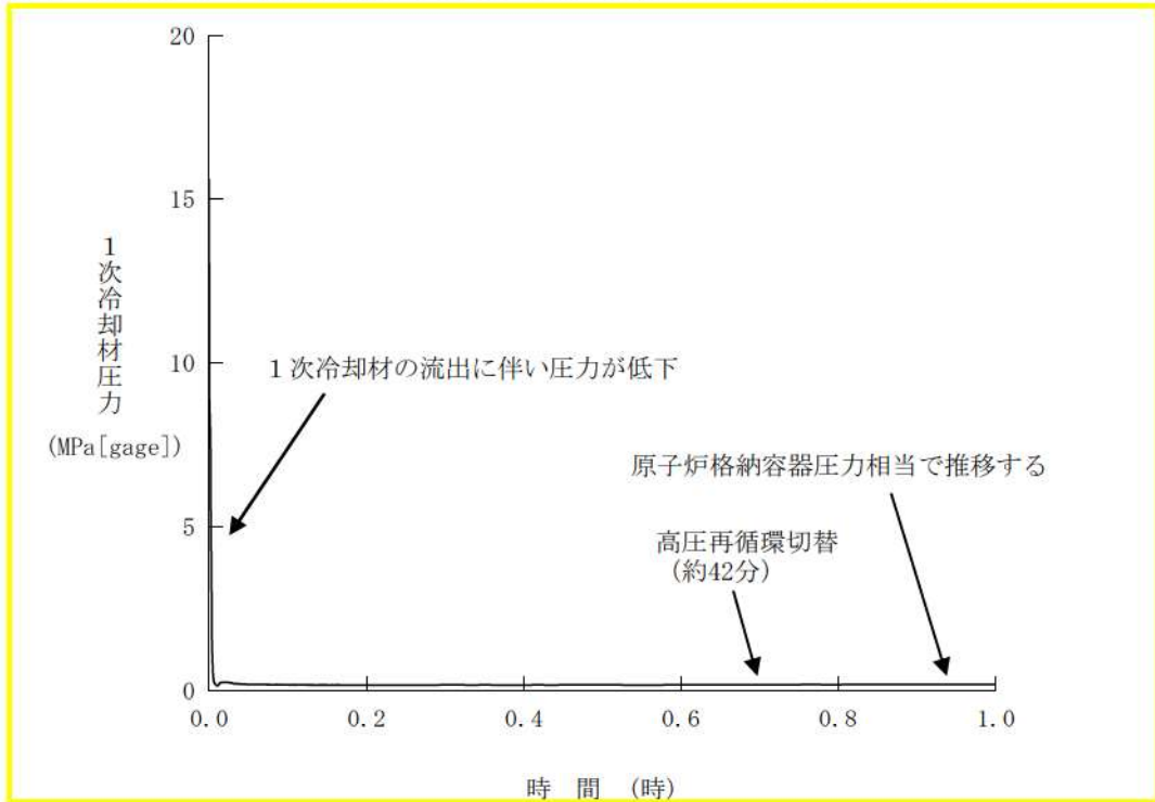
図1 1次冷却材圧力の推移 (本資料 第7.1.4.4図の拡大図)
