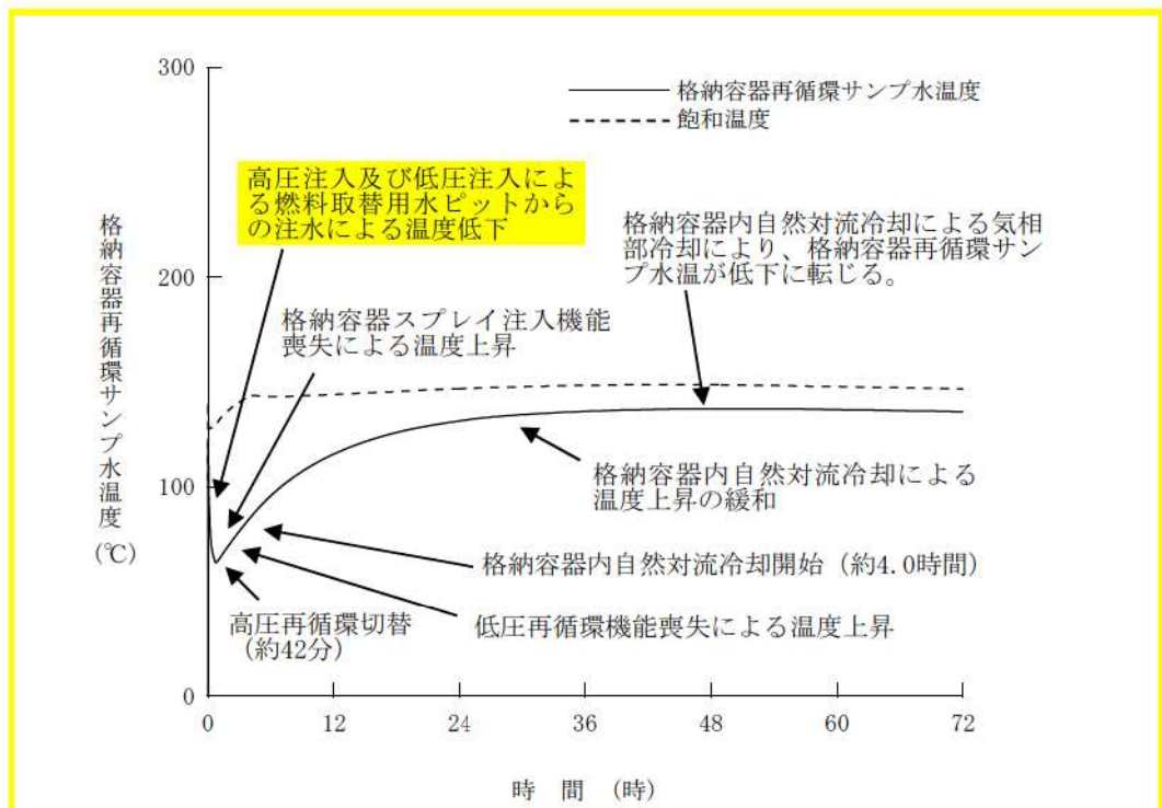
第 7.1.4.11 図 格納容器再循環サンプル水温度の推移
