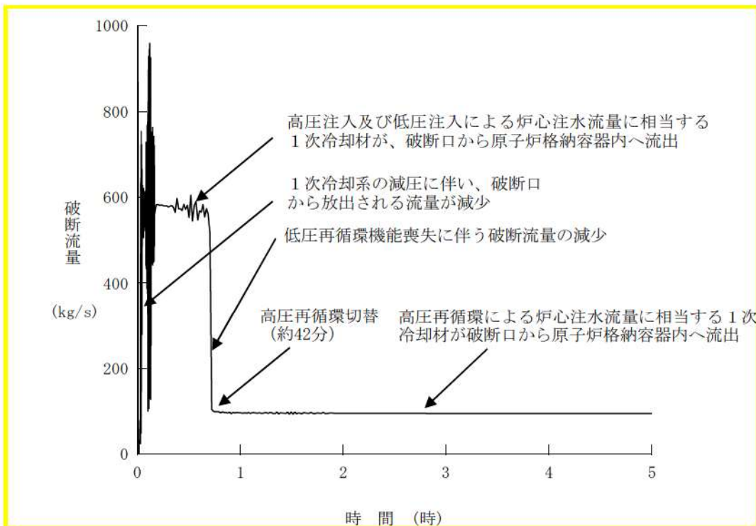
図2 破断流量の推移 (本資料 第7.1.4.5図の拡大図)
