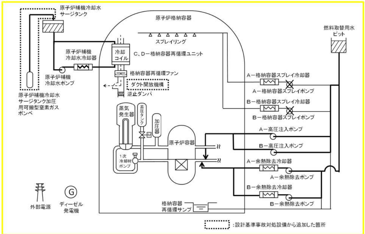
第 7.1.4.1 図 「原子炉格納容器の除熱機能喪失」の重大事故等対策の概略系統図 (1 / 2) (低圧注入, 高圧注入及び格納容器内自然対流冷却)
