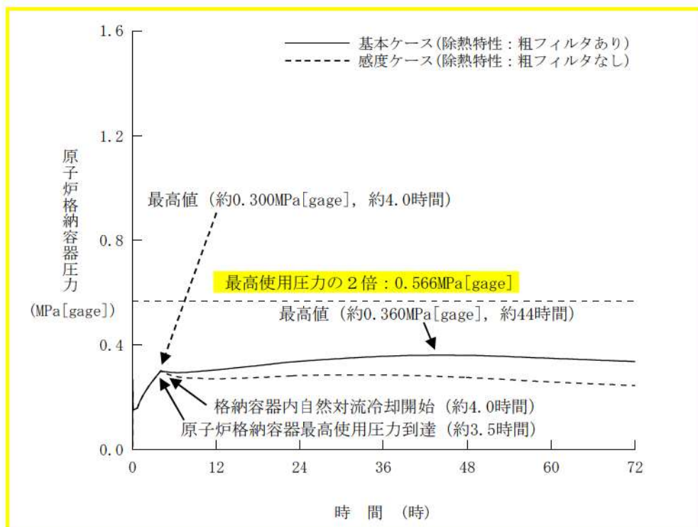
第7.1.4.15 図 原子炉格納容器圧力の推移 (格納容器再循環ユニット除熱特性の影響確認)
