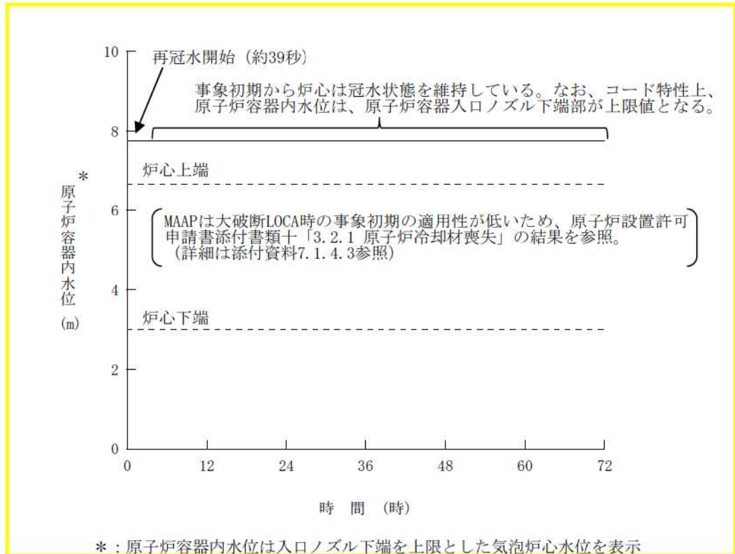
第 7.1.4.8 図 原子炉容器内水位の推移
