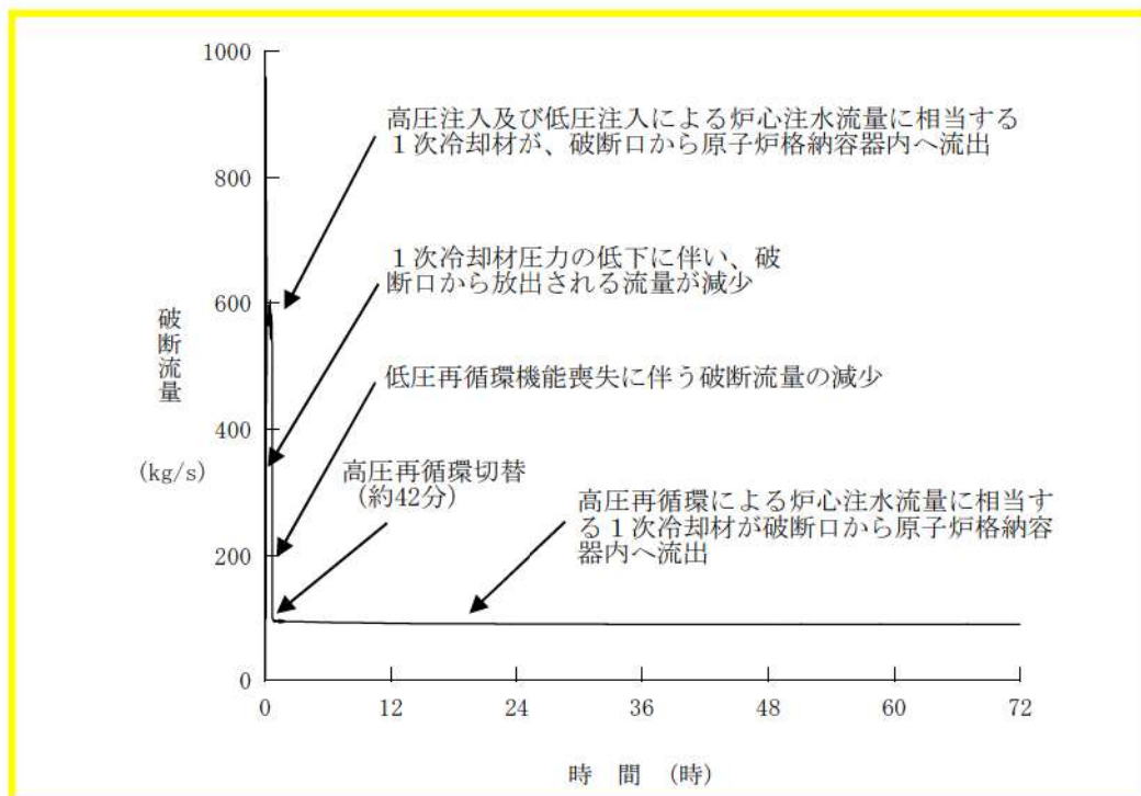
第 7.1.4.5 図 破断流量の推移※
