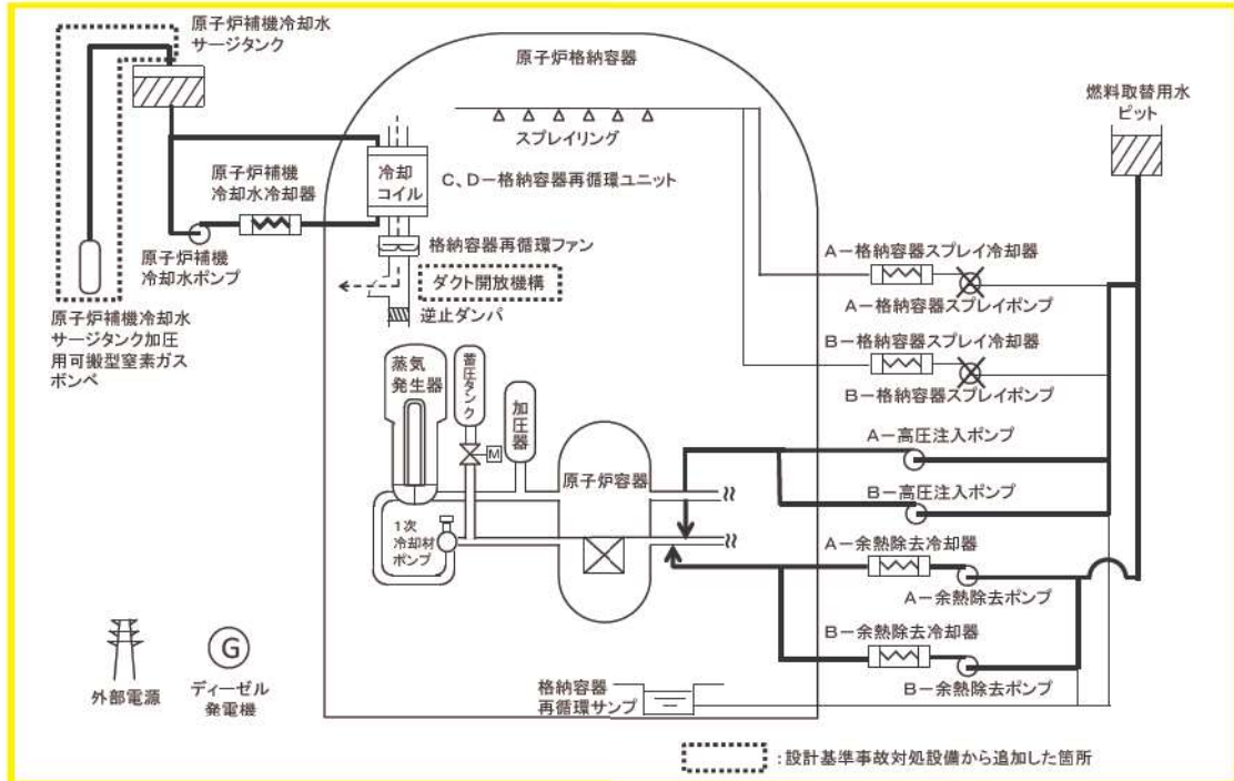
図1 「大破断 LOCA時に低圧再循環機能及び格納容器スプレイ注入機能が喪失する事故」の重大事故等対策の概略系統図（低圧注入，高圧注入及び格納容器内自然対流冷却）
