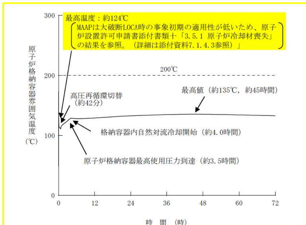
第 7.1.4.14 図 原子炉格納容器雰囲気温度の推移
