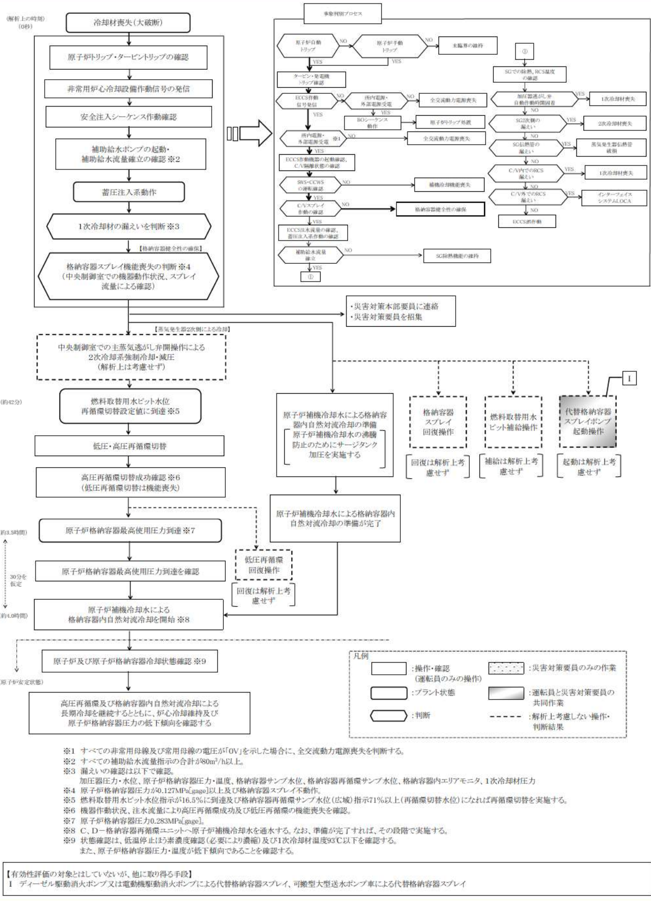
第 7.1.4.2 図 「原子炉格納容器の除熱機能喪失」の対応手順の概要 (「大破断 LOCA 時に低圧再循環機能及び格納容器スプレイ注入機能が喪失する事故」の事象進展)
