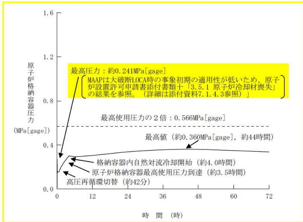
第 7.1.4.13 図 原子炉格納容器圧力の推移
