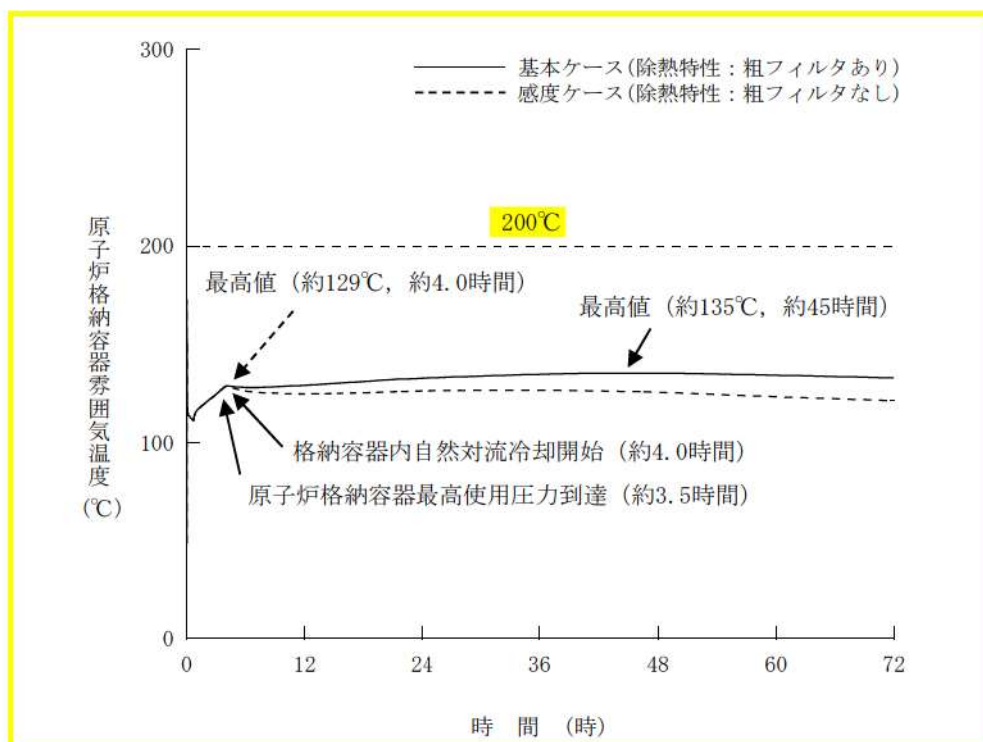
第7.1.4.16 図 原子炉格納容器雰囲気温度の推移 (格納容器再循環ユニット除熱特性の影響確認)
