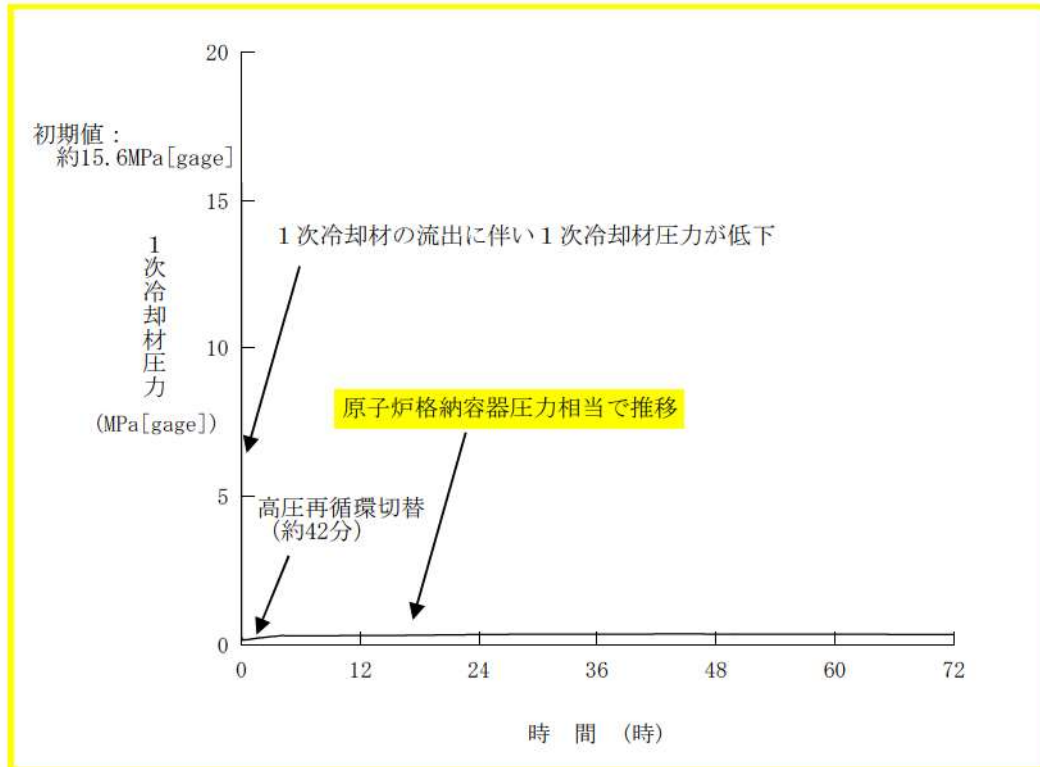
第 7.1.4.4 図 1次冷却材圧力の推移※
