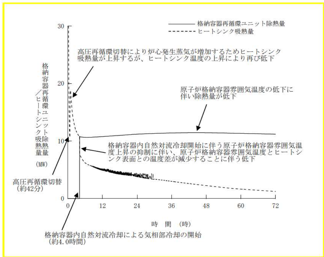
第 7. 1. 4. 12 図 原子炉格納容器からの除熱量の推移
