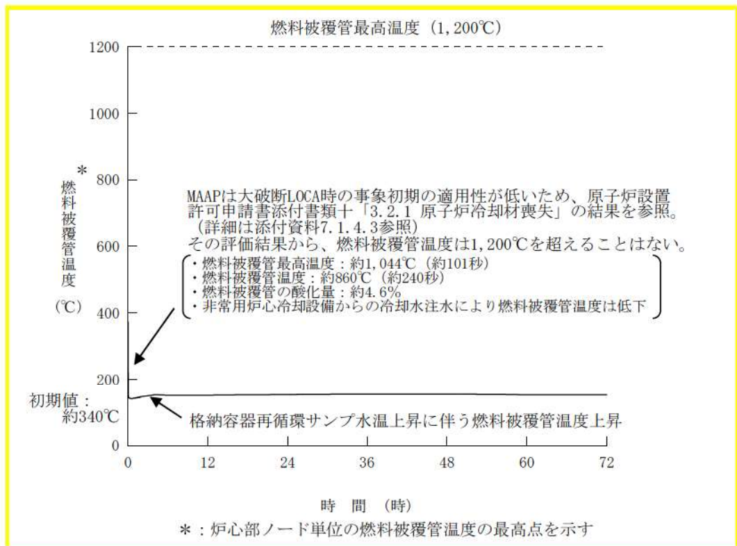
第 7.1.4.9 図 燃料被覆管温度の推移
