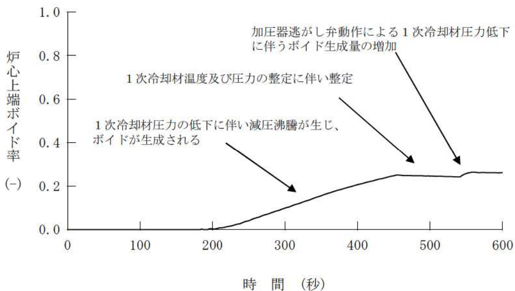
第 7.1.5.11 図 炉心上端ボイド率の推移 (主給水流量喪失)
