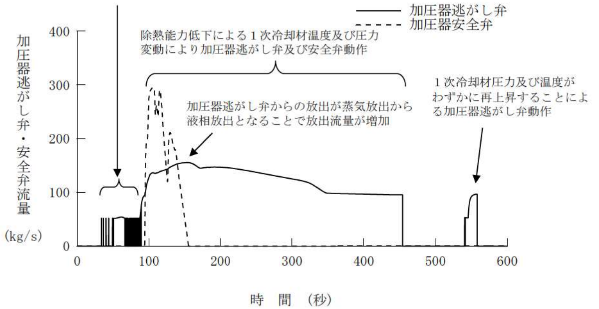
第 7.1.5.9 図 加圧器逃がし弁・安全弁流量の推移 (主給水流量喪失)
