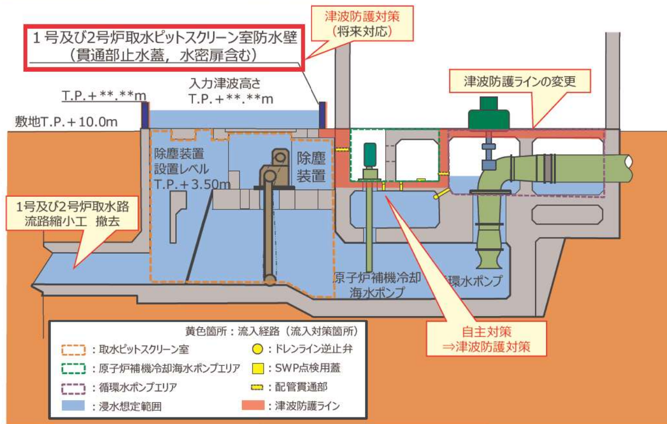
【1号及び2号炉取水系統断面図】 ※1号及び2号炉新規制基準適合性審査段階
