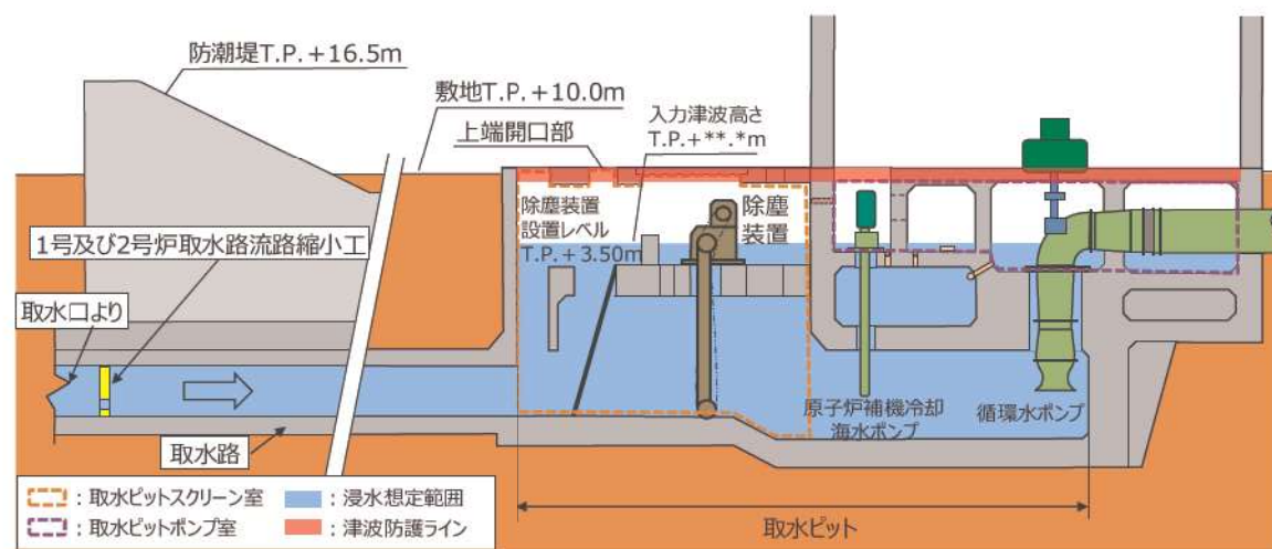
図10 1号及び2号炉取水路断面図
