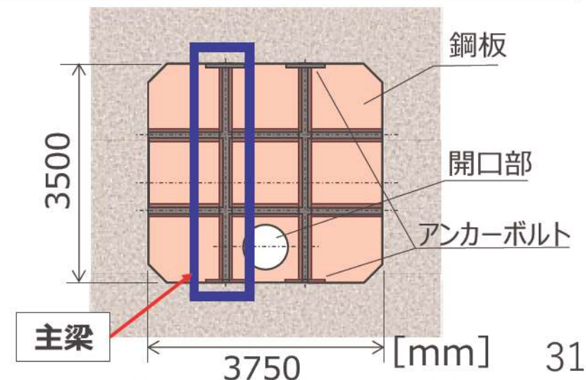
【1号及び2号炉取水路流路縮小工 概略図】
