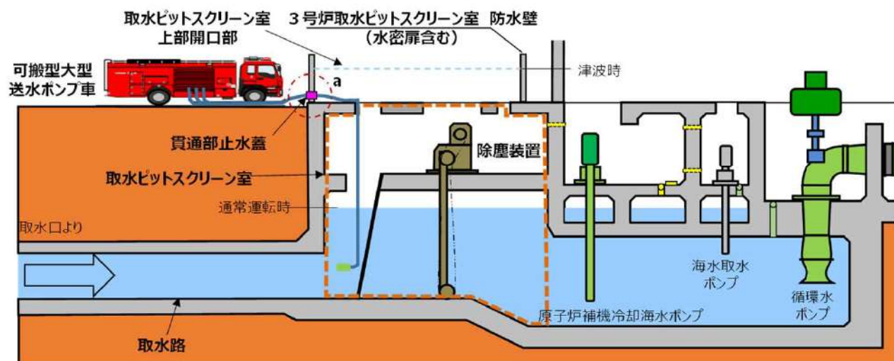
図8 3号炉取水路断面図
