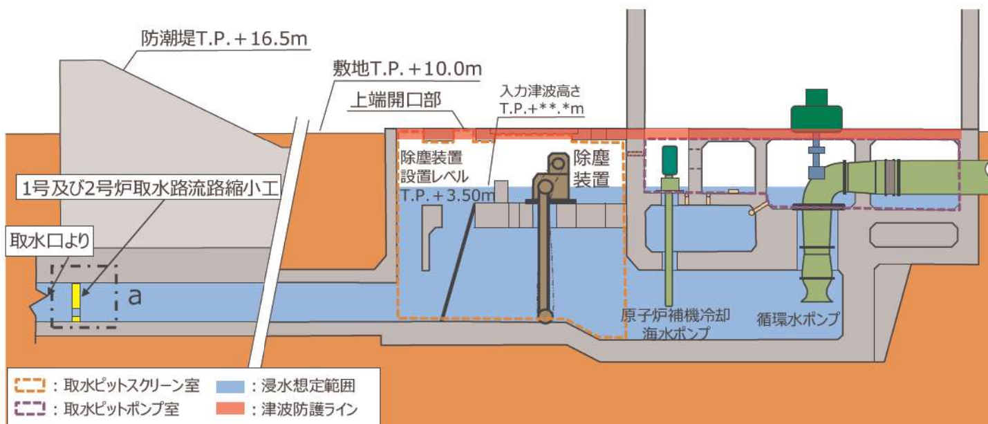
図3 1号及び2号炉取水路断面図
