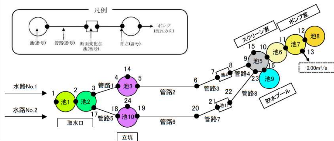
【3号炉取水路モデル図】
