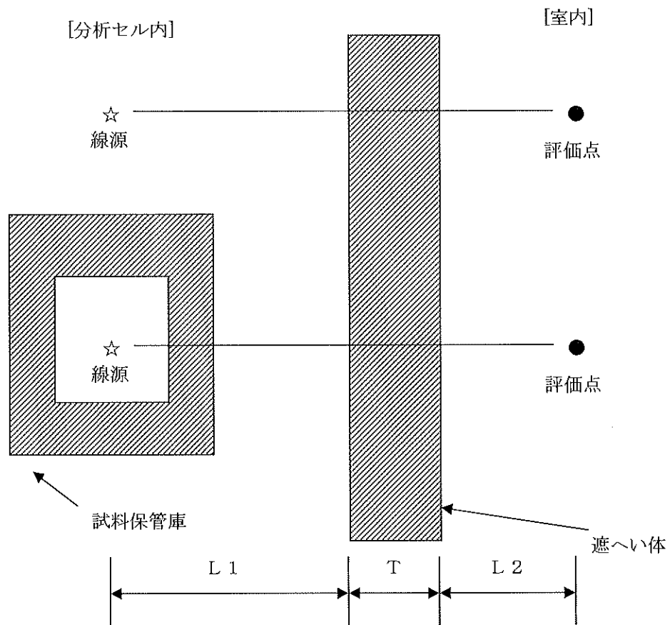
図-1 分析セル等の遮へい計算モデル
