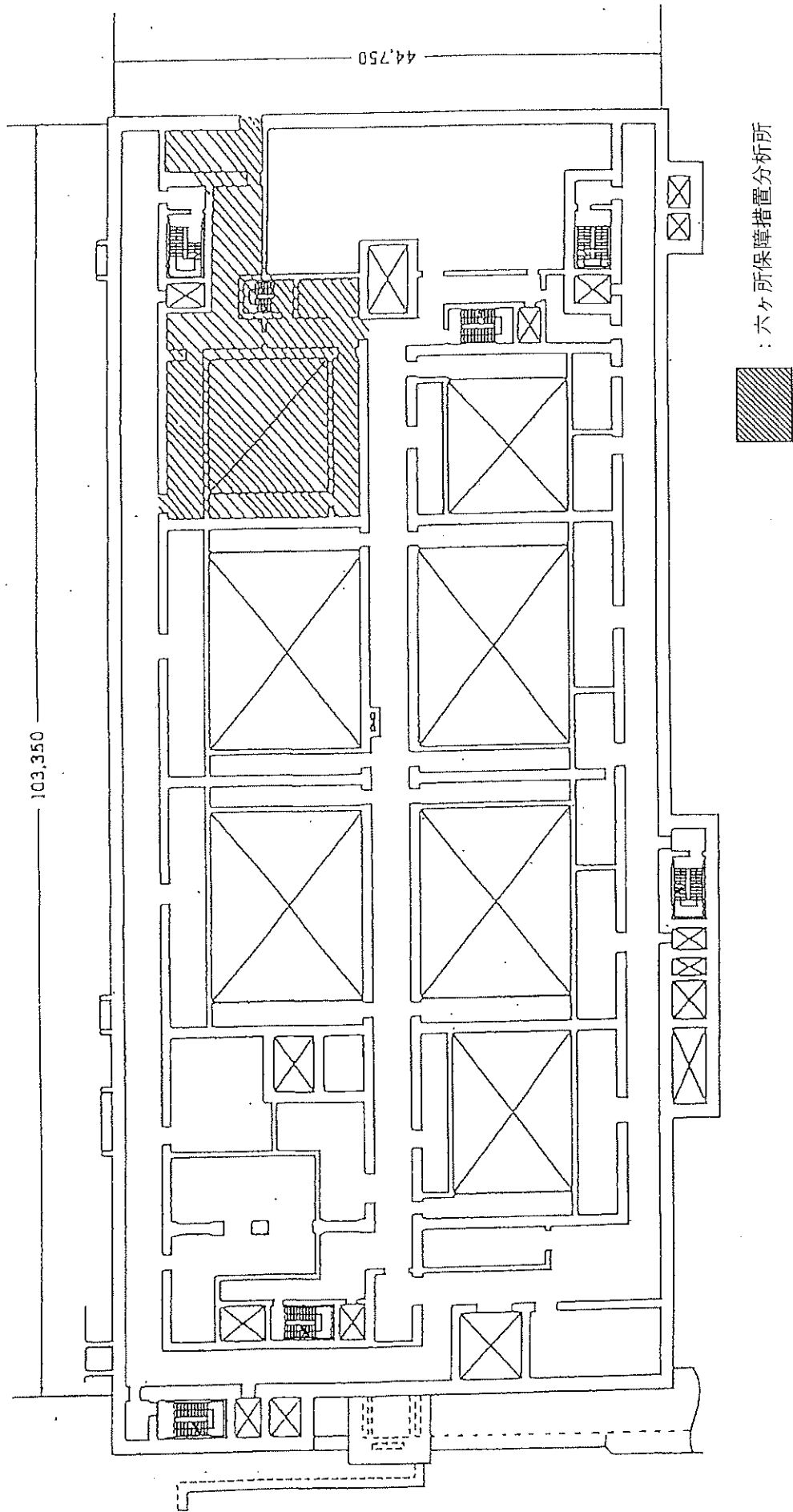
図7-2 分析建屋地下1階平面図
