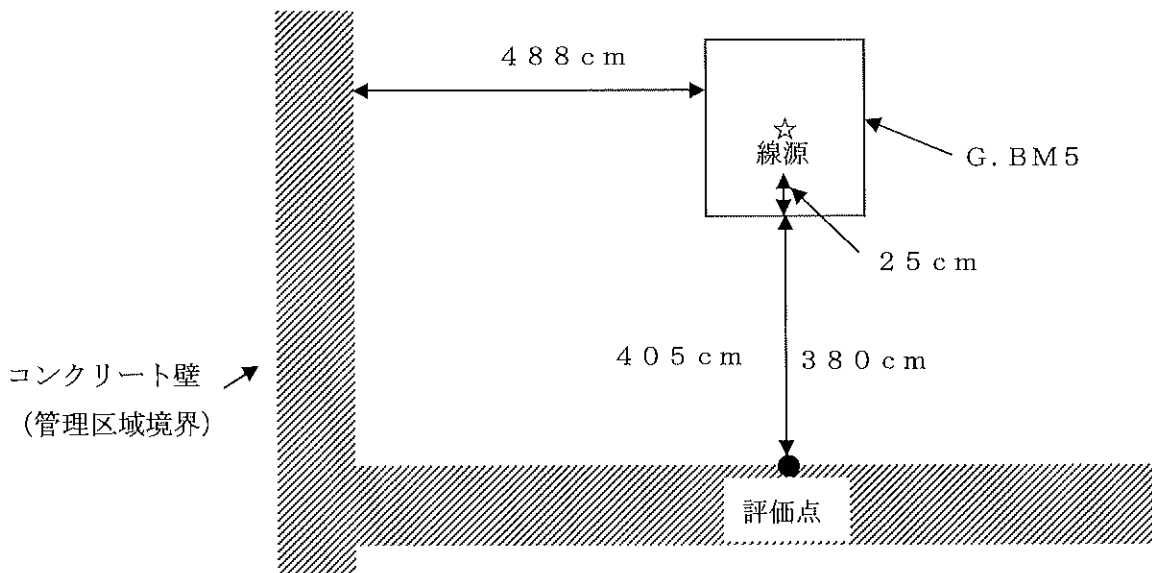
図-1 分析セル等の遮へい計算モデル
