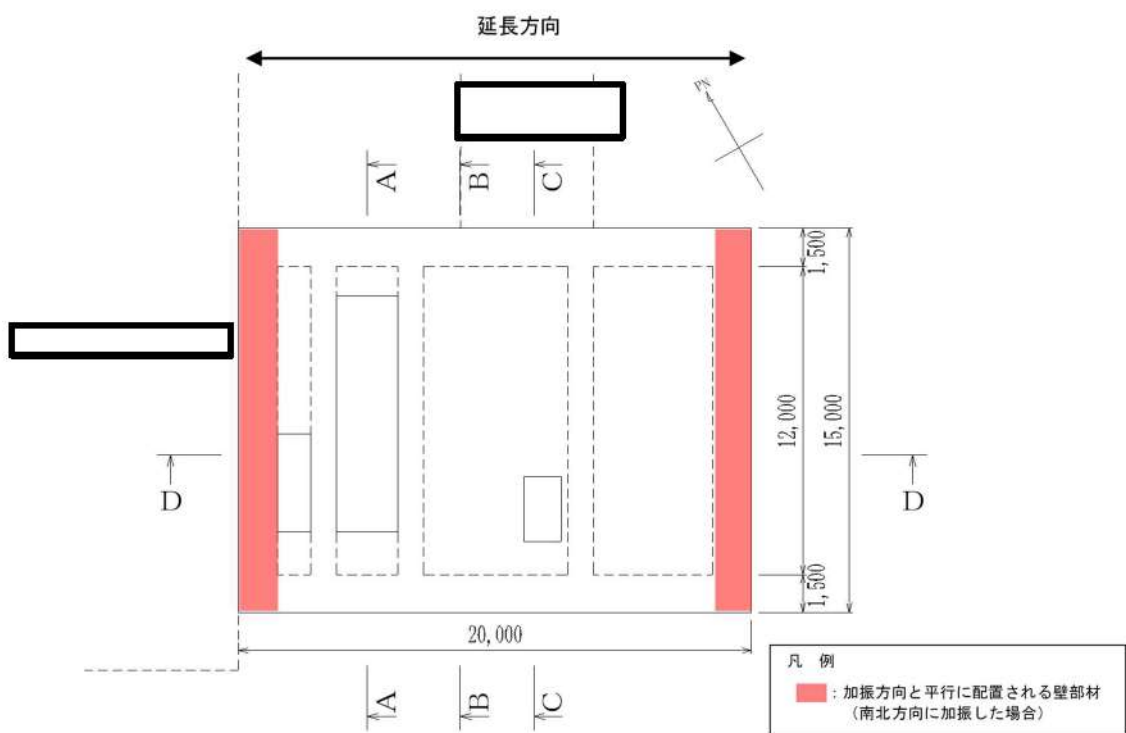
第 8-2-8-2 図 原子炉補機冷却海水ポンプ出口ストレーナ室 平面図
