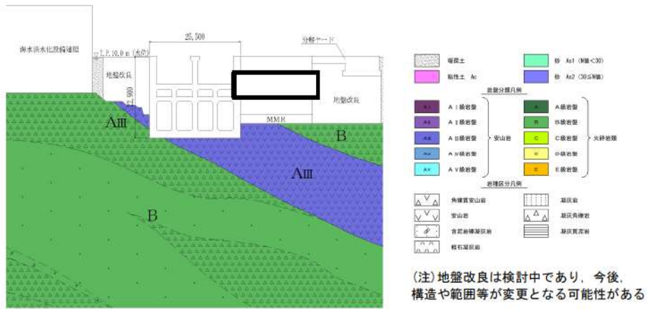
第 8-2-7-8 図 取水ピットポンプ室 地質断面図 (A-A 断面)
