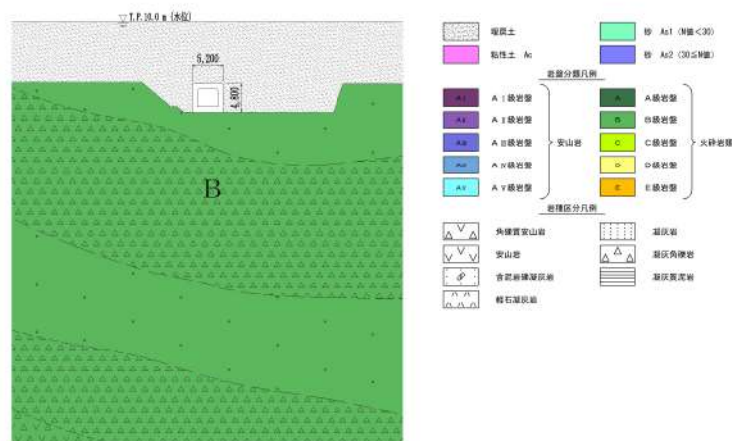
第6-31図 原子炉補機冷却海水管ダクト 地質断面図 (最深部：B-B断面)
