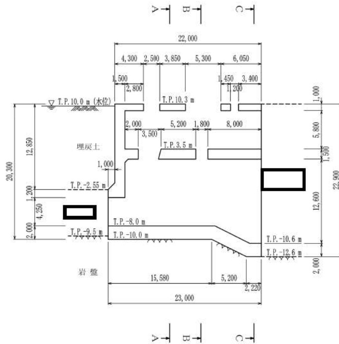
第6-48図 取水ピットスクリーン室 断面図 (D-D断面)
