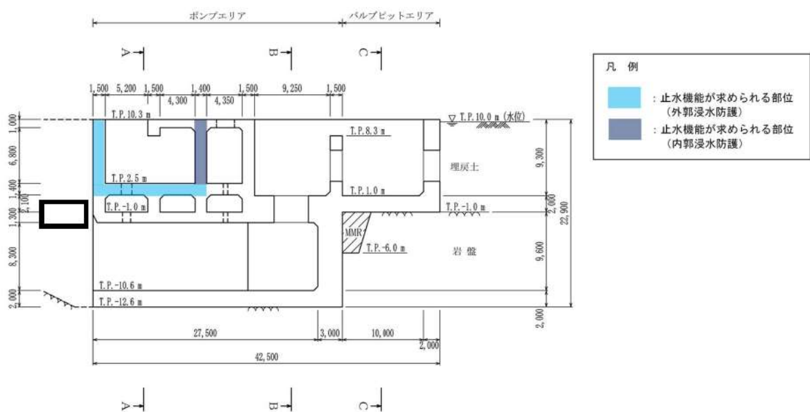
第6-54 図 取水ピットポンプ室 断面図 (D-D 断面)
