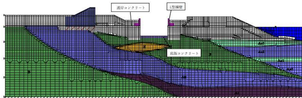
参考 1-3 図 取水口の解析モデル
