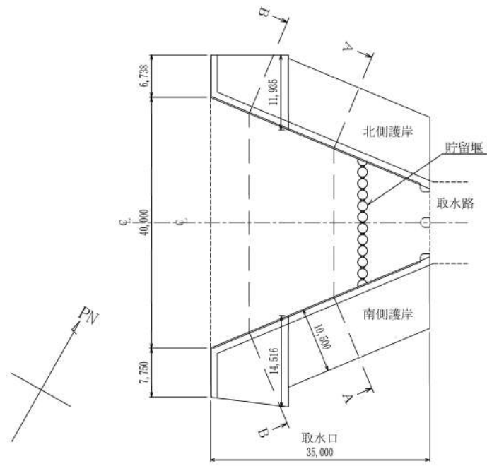
第 6-6 図 取水口 平面図
