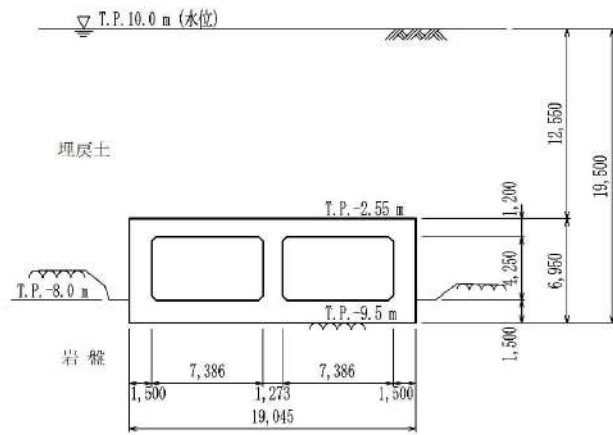
第 8-2-3-6 図 取水路 断面図 (D-D 断面)
