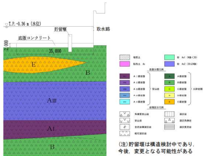
第 8-2-2-6 図 取水口 地質断面図 (縦断面)
