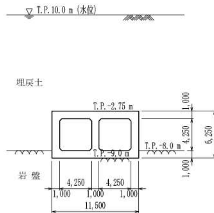
第 6-15 図 取水路 断面図 (C-C 断面)
