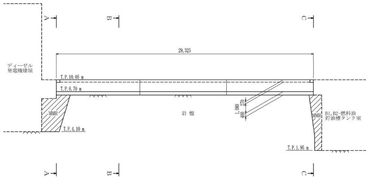
第 6-40 図 B1, B2-ディーゼル発電機燃料油貯油槽トレンチ 断面図 (縦断)
