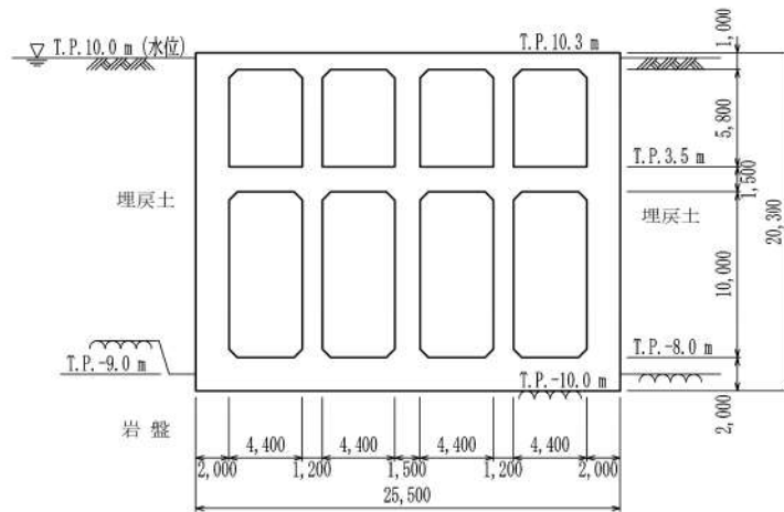
第6-45図 取水ピットスクリーン室 断面図 (A-A 断面)
