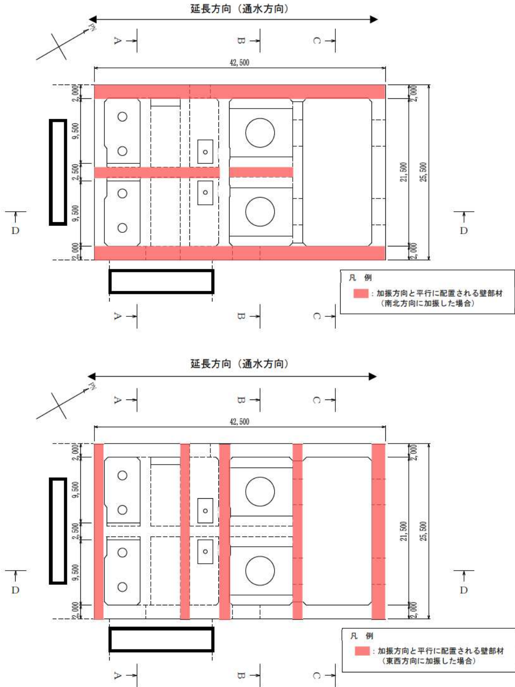
第 6-52 図 取水ピットポンプ室 平面図
