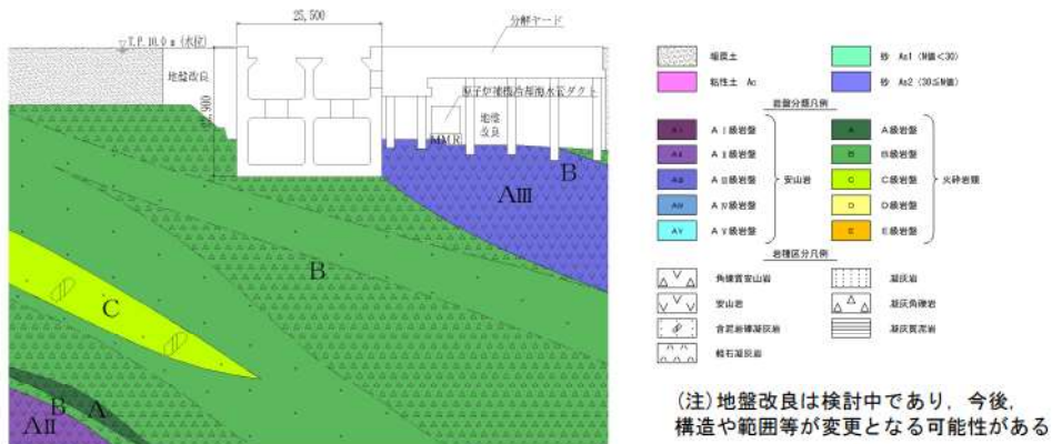
第 6-59 図 取水ピットポンプ室 地質断面図 (B-B 断面)
