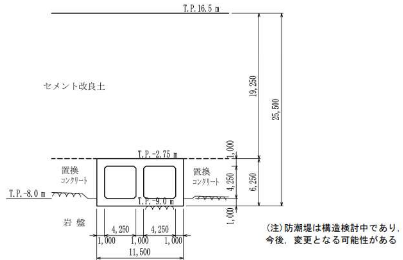
第 6-14 図 取水路 断面図 (B-B 断面)
