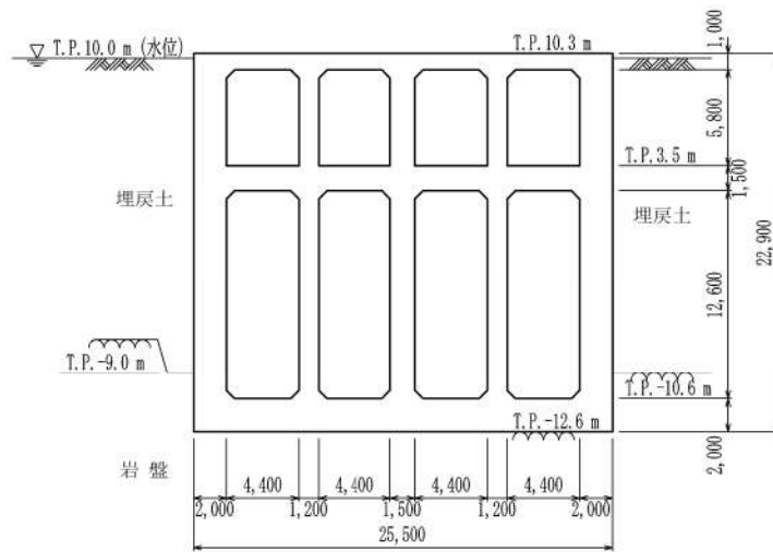
第6-47図 取水ピットスクリーン室 断面図 (C-C断面)
