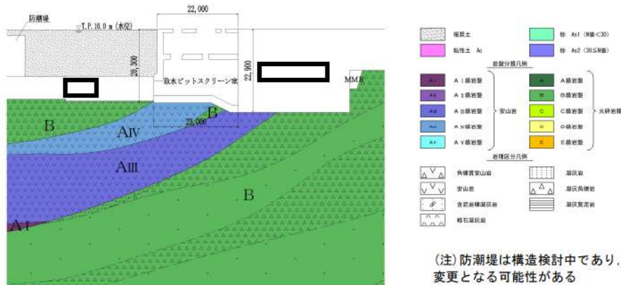
第6-50図 取水ピットスクリーン室 地質断面図 (D-D断面)
