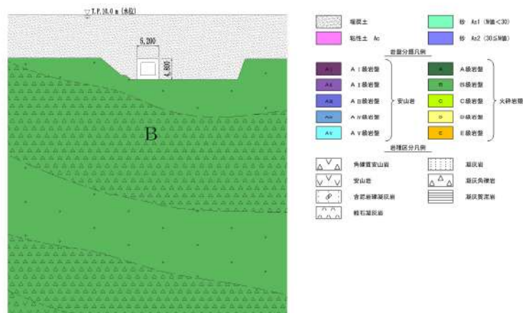
第 8-2-4-9 図 原子炉補機冷却海水管ダクト 地質断面図 (B-B 断面)
