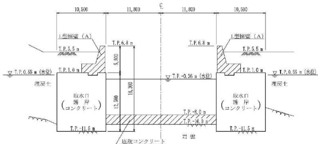
参考 1-2 図 取水口 断面図 (A-A断面)
