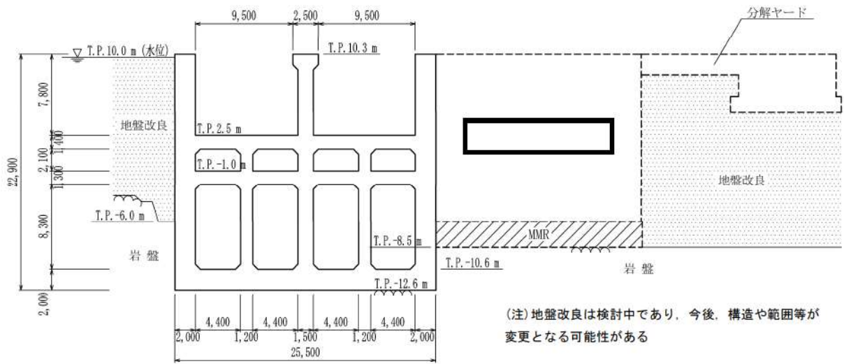
第6-55図 取水ピットポンプ室 断面図 (A-A 断面)
