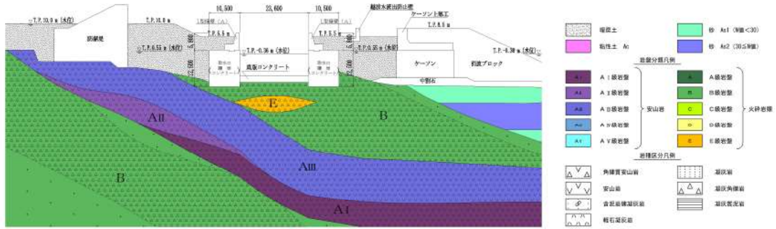
第6-9図 取水口 地質断面図 (A-A断面)
