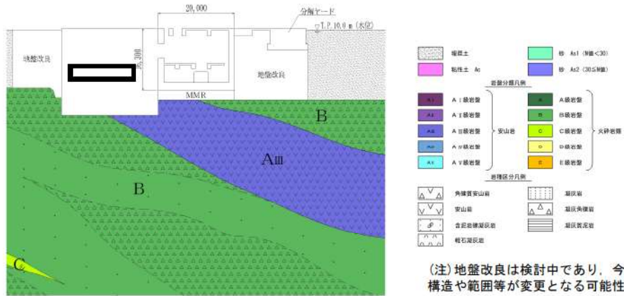
第 6-69 図 原子炉補機冷却海水ポンプ出口ストレーナ室 地質断面図 (D-D 断面)
