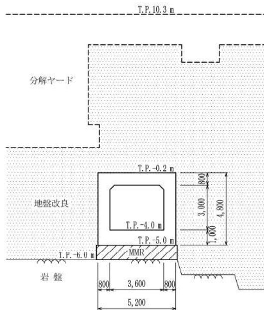
第 6-25 図 原子炉補機冷却海水管ダクト 断面図 (A-A 断面)
