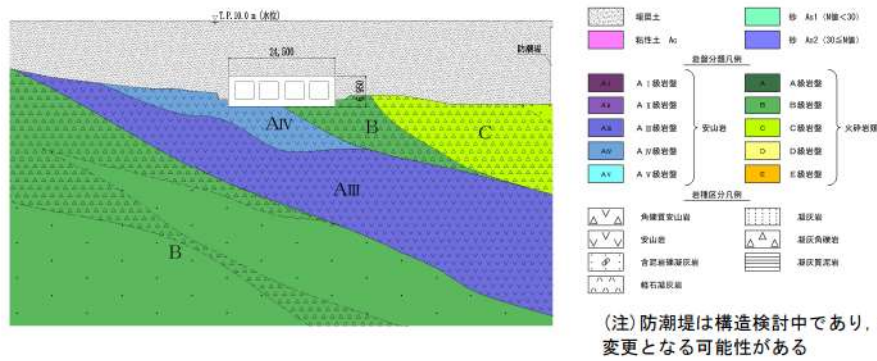
第 6-21 図 取水路 地質断面図 (E-E 断面)
