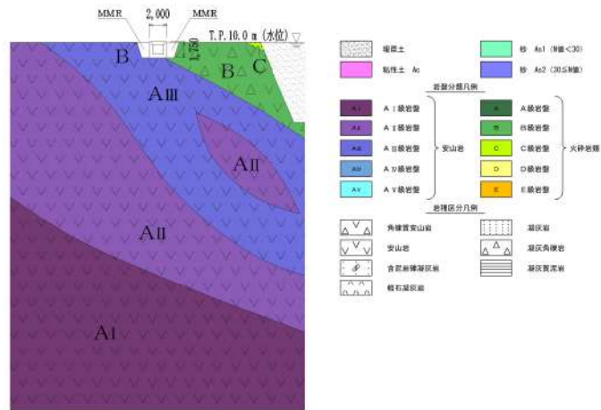
第 6-41 図 B1, B2-ディーゼル発電機燃料油貯油槽トレンチ 地質断面図 (B-B 断面)
