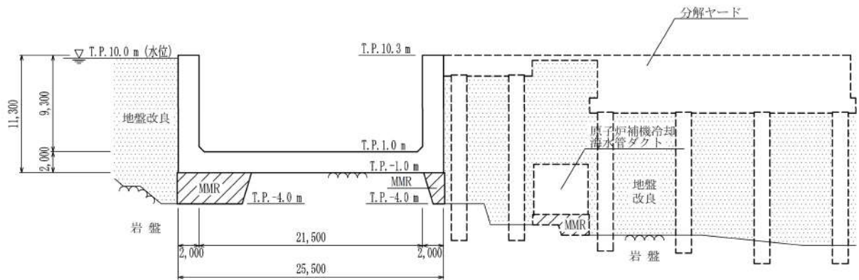
第6-57図 取水ピットポンプ室 断面図 (C-C 断面)
