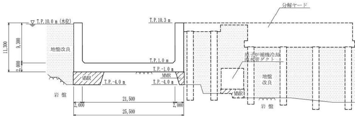
第8-2-7-6図 取水ピットポンプ室 断面図 (B-B断面)
