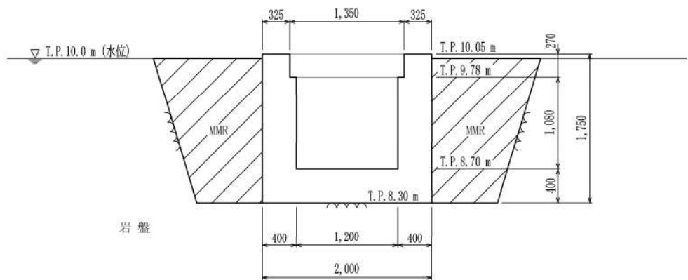
第 6-38 図 B1, B2-ディーゼル発電機燃料油貯油槽トレンチ 断面図 (B-B 断面)
