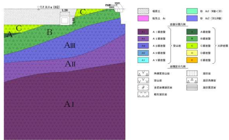
第 6-33 図 原子炉補機冷却海水管ダクト 地質断面図 (最浅部：E-E 断面)
