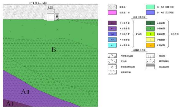
第 6-32 図 原子炉補機冷却海水管ダクト 地質断面図 (中間部：C-C 断面)
