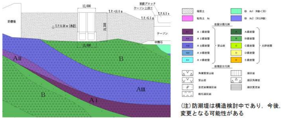
第 8-2-3-9 図 取水路 地質断面図 (A-A 断面)
