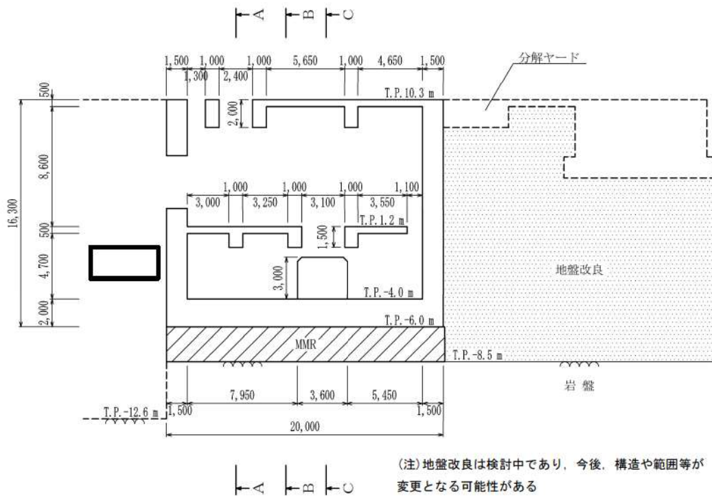
第 8-2-8-6 図 原子炉補機冷却海水ポンプ出口ストレーナ室 断面図 (D-D 断面)
