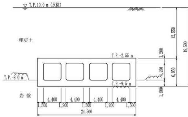
第 6-17 図 取水路 断面図 (E-E 断面)
