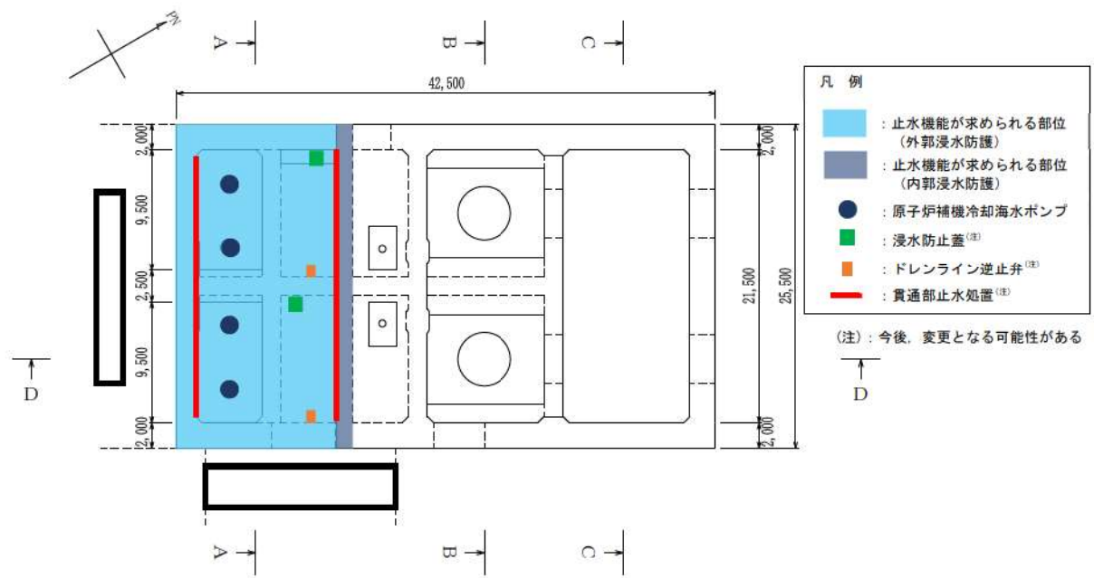
第6-53 図 取水ピットポンプ室 設置される設備の配置図 (平面図)
