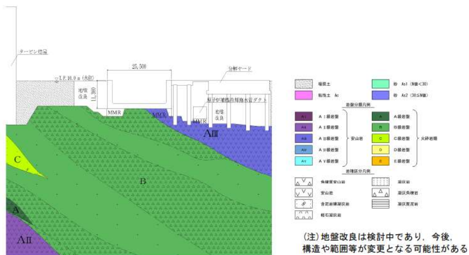
第 6-60 図 取水ピットポンプ室 地質断面図 (C-C 断面)
