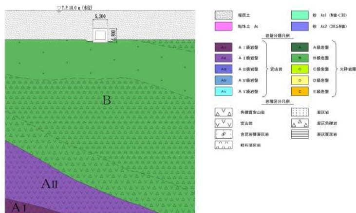
第 8-2-4-10 図 原子炉補機冷却海水管ダクト 地質断面図 (C-C断面)
