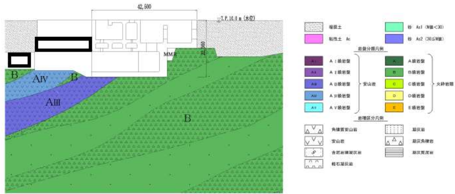
第 6-61 図 取水ピットポンプ室 地質断面図 (D-D 断面)
