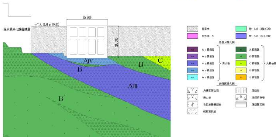
第6-49図 取水ピットスクリーン室 地質断面図 (A-A断面)
