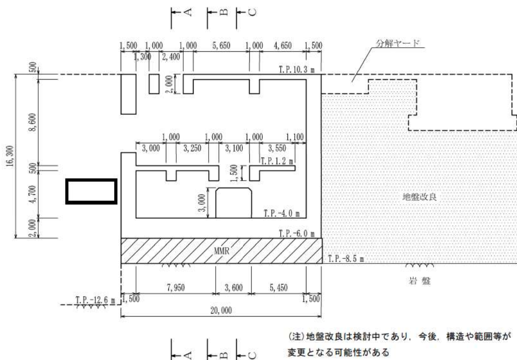
第 6-67 図 原子炉補機冷却海水ポンプ出口ストレーナ室 断面図 (D-D 断面)
