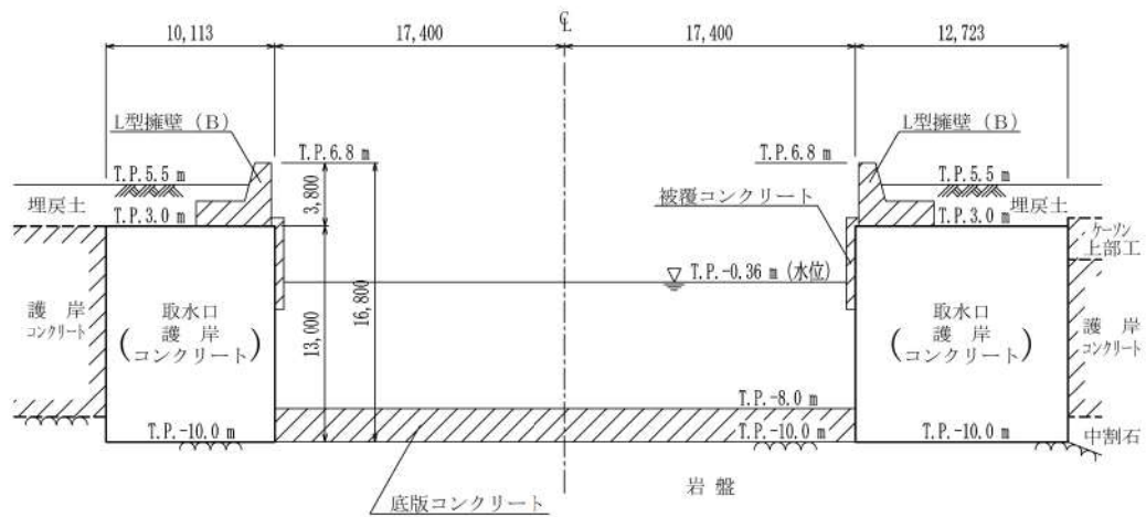
第6-8図 取水口 断面図 (B-B断面)
