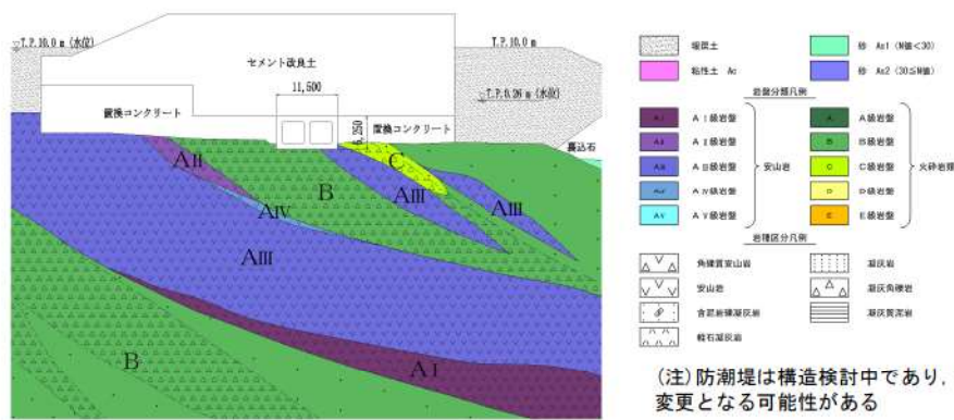
第 6-20 図 取水路 地質断面図 (B-B 断面)
