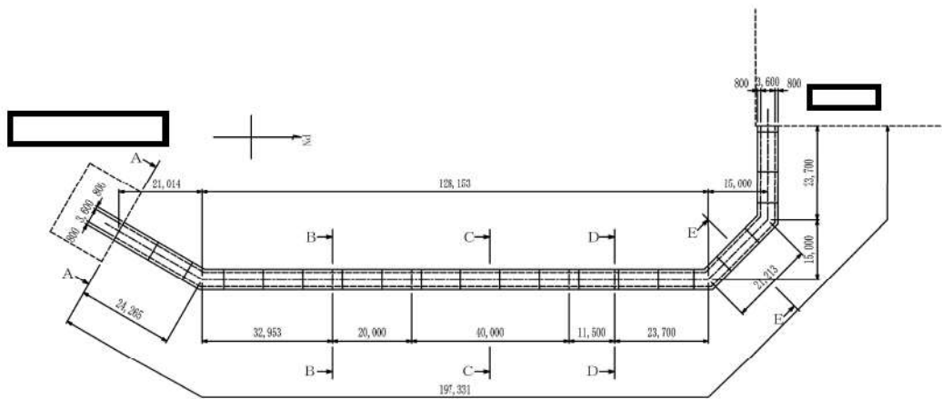
第 6-24 図 原子炉補機冷却海水管ダクト 平面図
