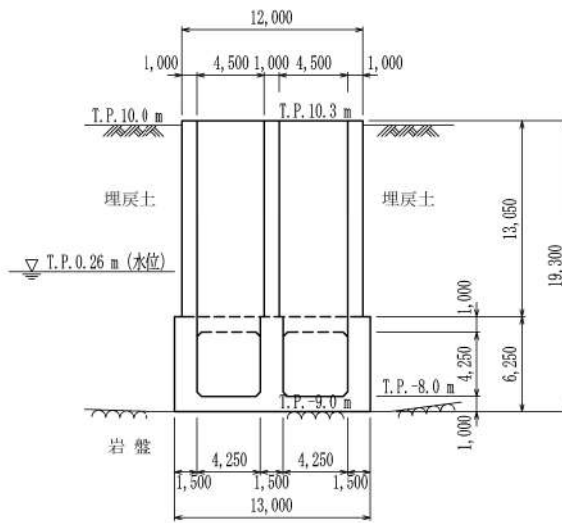
第 6-13 図 取水路 断面図 (A-A 断面)
