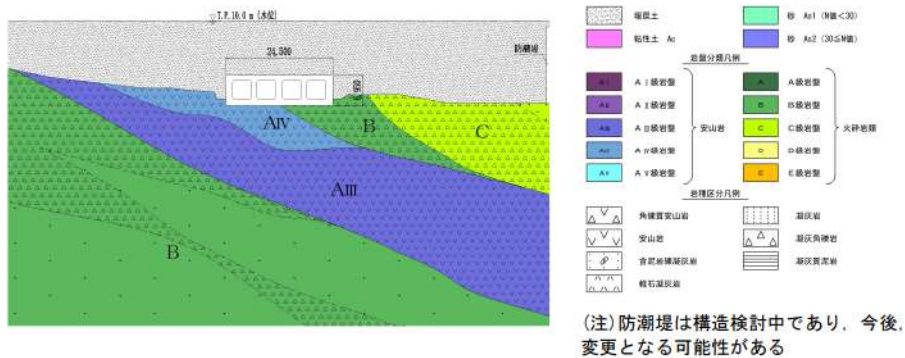
第 8-2-3-11 図 取水路 地質断面図 (E-E 断面)
