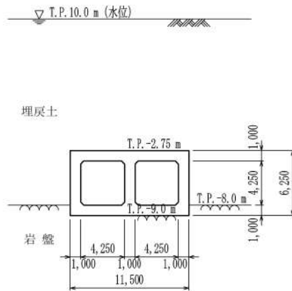
第 8-2-3-5 図 取水路 断面図 (C-C 断面)
