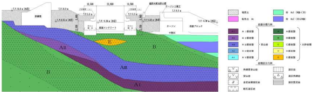
第 8-2-2-5 図 取水口 地質断面図 (A-A 断面)
