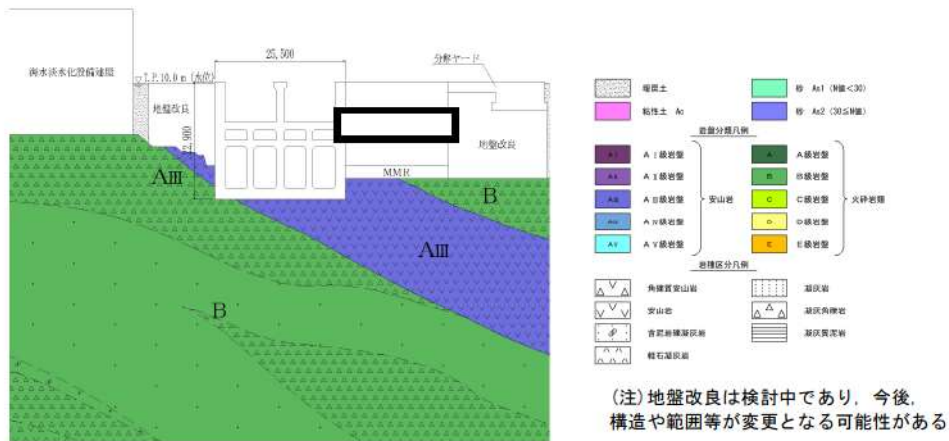
第 6-58 図 取水ピットポンプ室 地質断面図 (A-A 断面)
