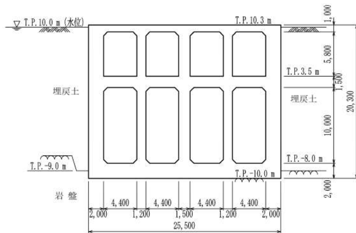
第 8-2-6-3 図 取水ピットスクリーン室 断面図 (A-A 断面)
