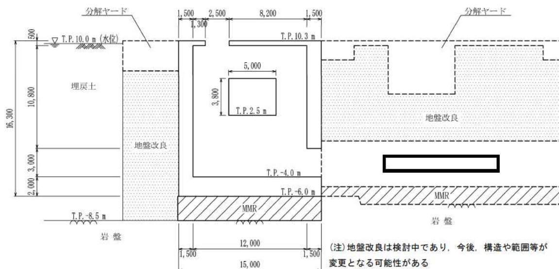
第 6-66 図 原子炉補機冷却海水ポンプ出口ストレーナ室 断面図 (C-C 断面)
