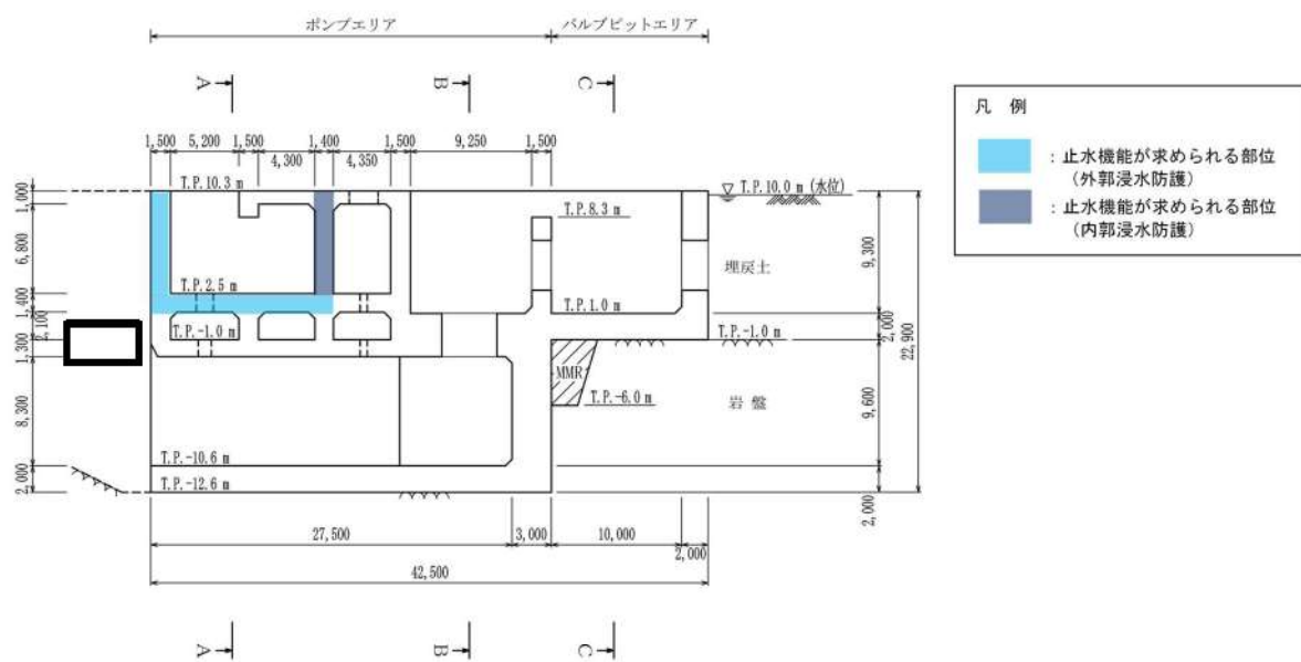
第8-2-7-4図 取水ピットポンプ室 断面図 (D-D断面)
