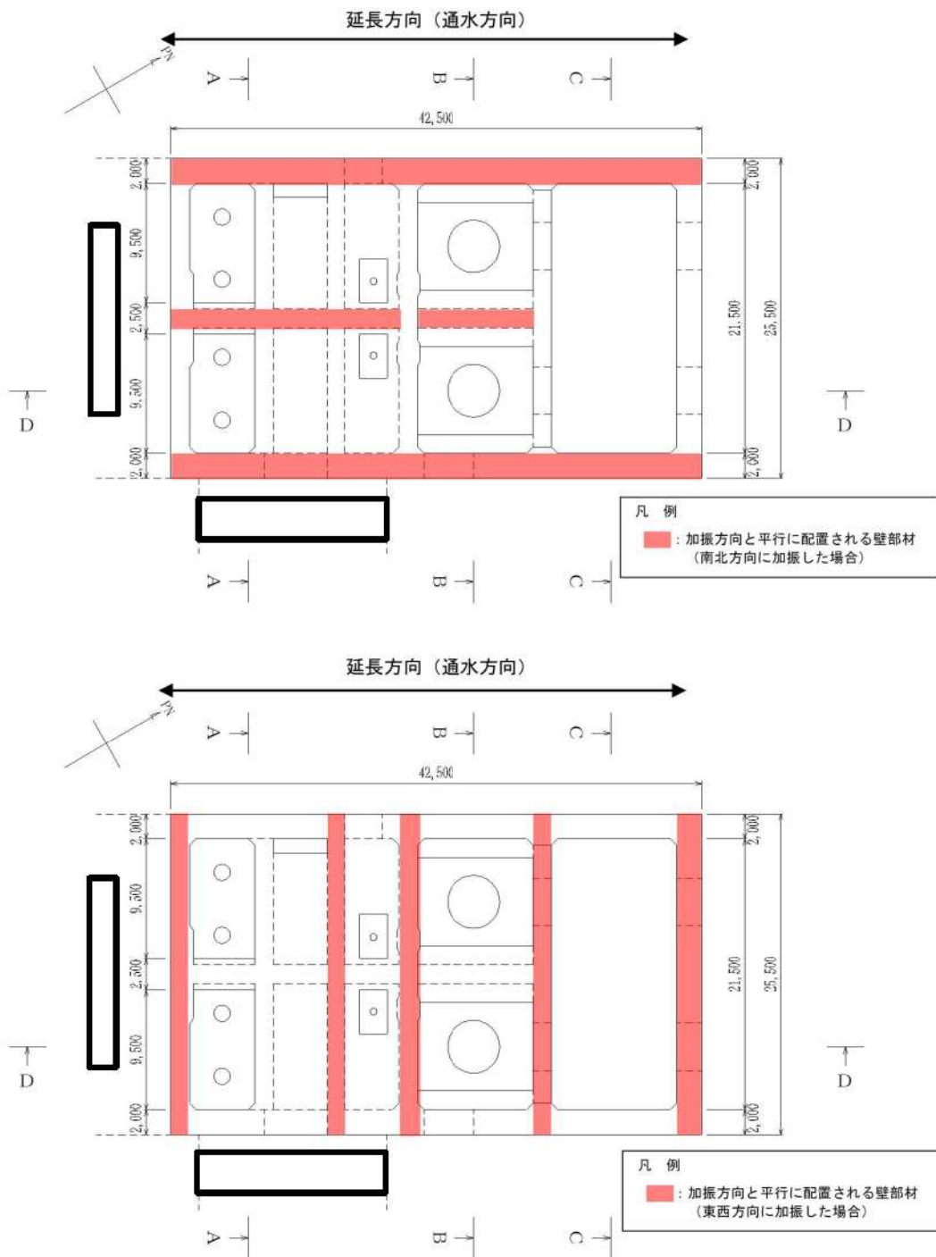
第8-2-7-2図 取水ピットポンプ室 平面図
