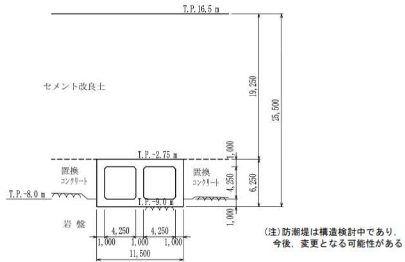
第 8-2-3-4 図 取水路 断面図 (B-B 断面)
