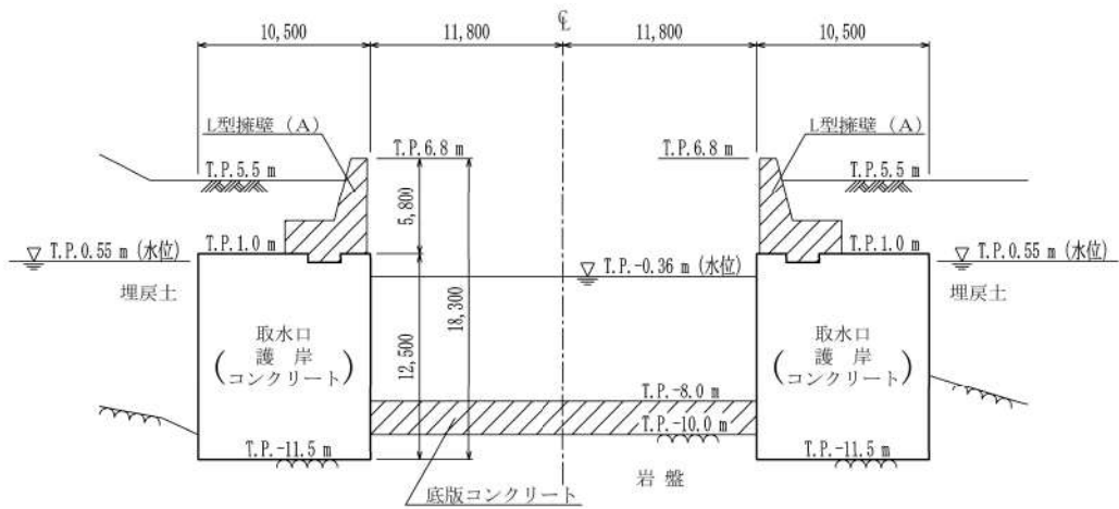
第8-2-2-3図 取水口 断面図 (A-A断面)
