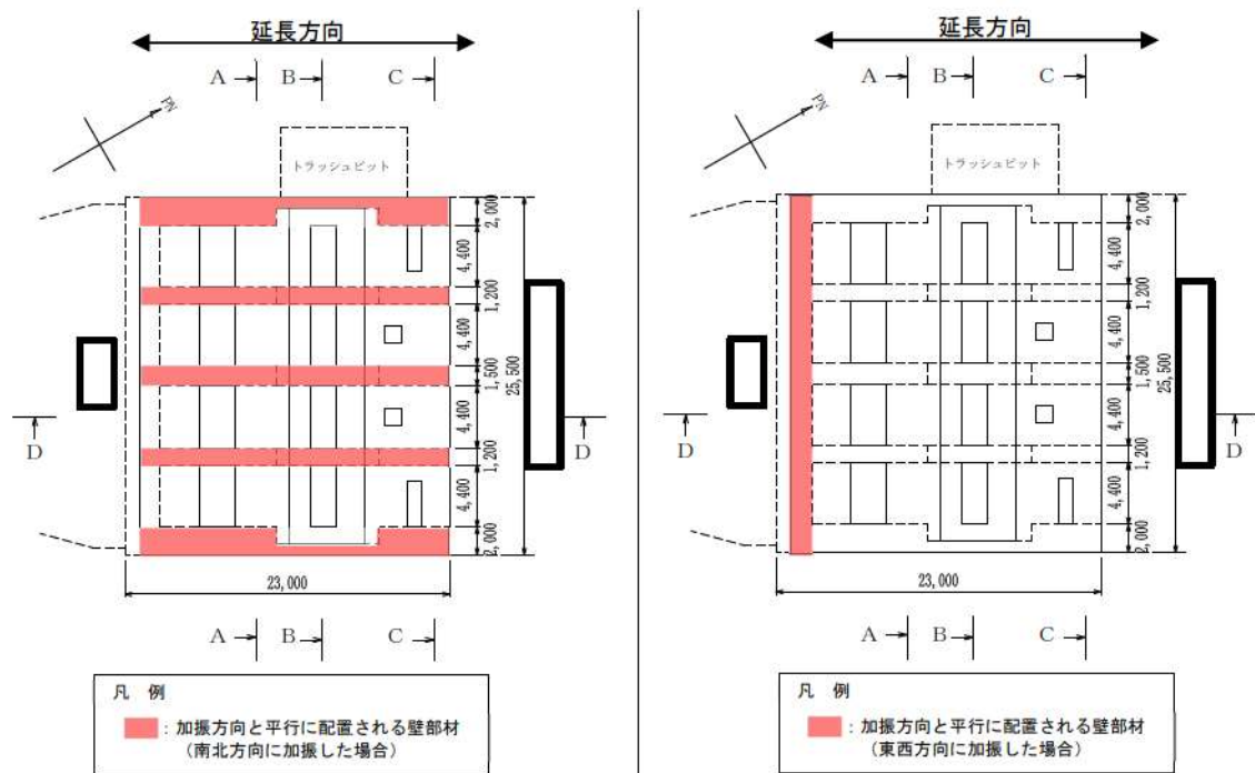
第 8-2-6-2 図 取水ピットスクリーン室 平面図
