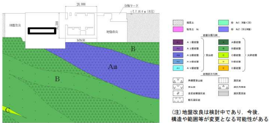
第 8-2-8-8 図 原子炉補機冷却海水ポンプ出口ストレーナ室 地質断面図 (D-D 断面)
