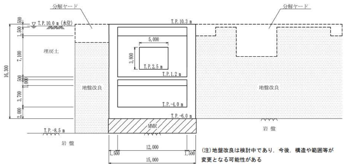
第 6-65 図 原子炉補機冷却海水ポンプ出口ストレーナ室 断面図 (B-B 断面)
