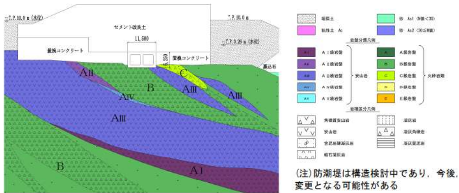
第 8-2-3-10 図 取水路 地質断面図 (B-B 断面)
