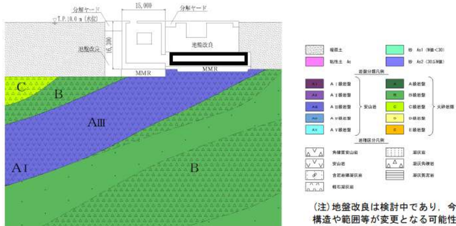
第 6-68 図 原子炉補機冷却海水ポンプ出口ストレーナ室 地質断面図 (C-C 断面)
