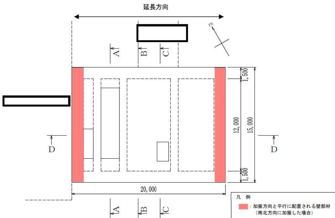
第 6-63 図 原子炉補機冷却海水ポンプ出口ストレーナ室 平面図
