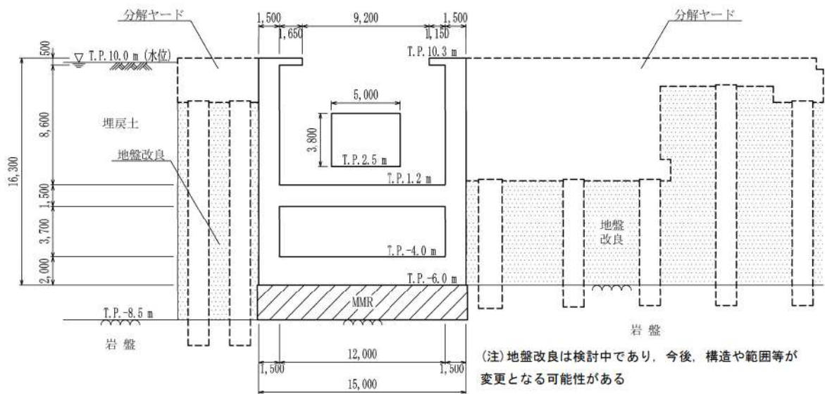
第 6-64 図 原子炉補機冷却海水ポンプ出口ストレーナ室 断面図 (A-A 断面)
