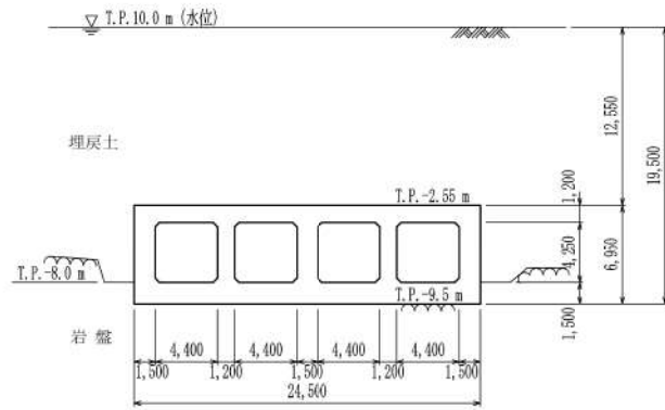
第 8-2-3-7 図 取水路 断面図 (E-E 断面)
