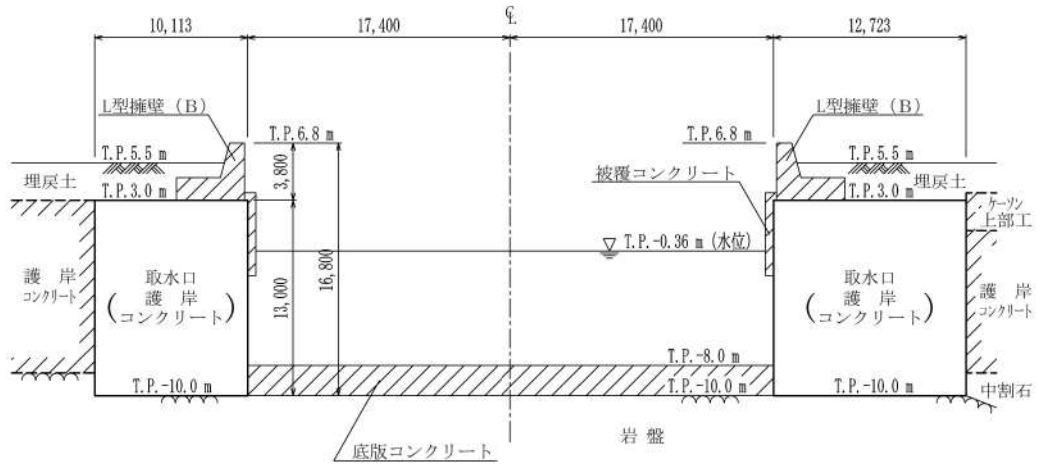
第 8-2-2-4 図 取水口 断面図 (B-B 断面)
