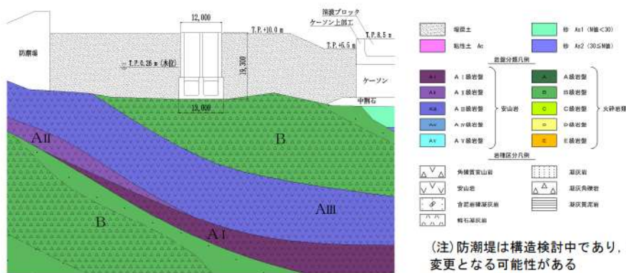
第 6-19 図 取水路 地質断面図 (A-A 断面)
