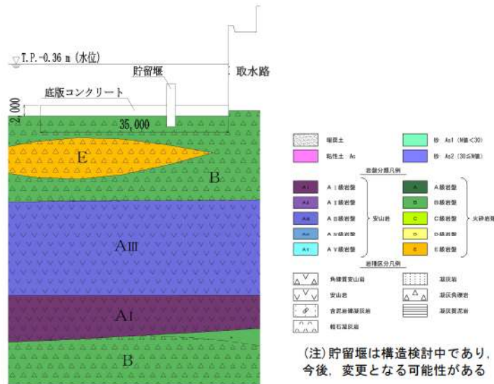
第6-10図 取水口 地質断面図 (縦断)
