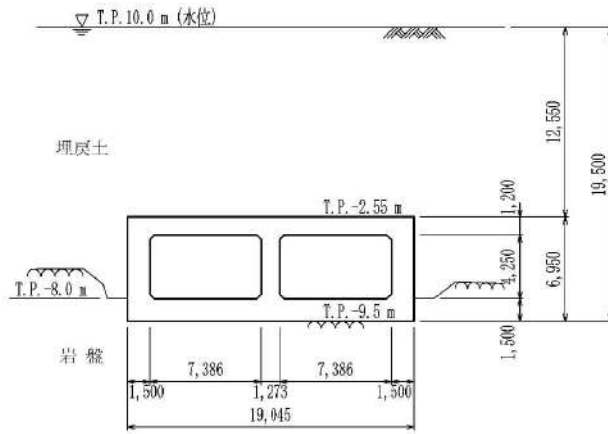
第 6-16 図 取水路 断面図 (D-D 断面)
