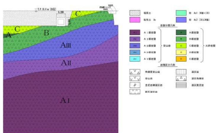
第 8-2-4-11 図 原子炉補機冷却海水管ダクト 地質断面図 (E-E断面)
