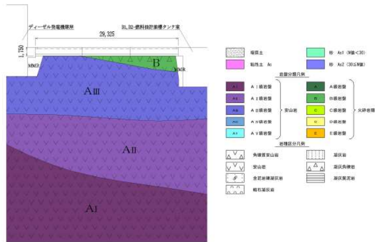
第 6-42 図 B1, B2-ディーゼル発電機燃料油貯油槽トレンチ 地質断面図 (縦断)
