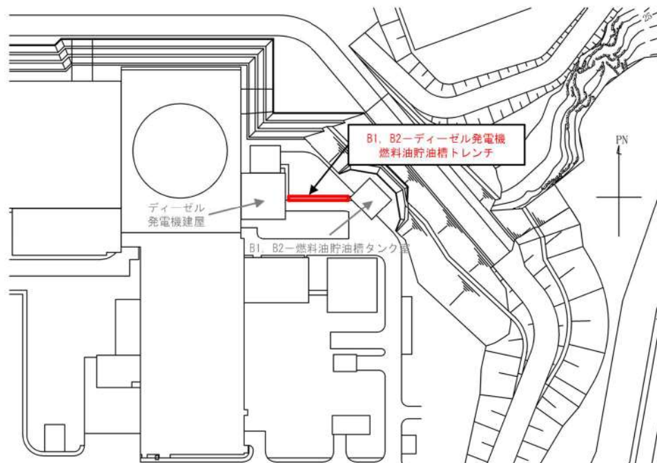
第6-35図 B1, B2-ディーゼル発電機燃料油貯油槽トレンチ 配置図
