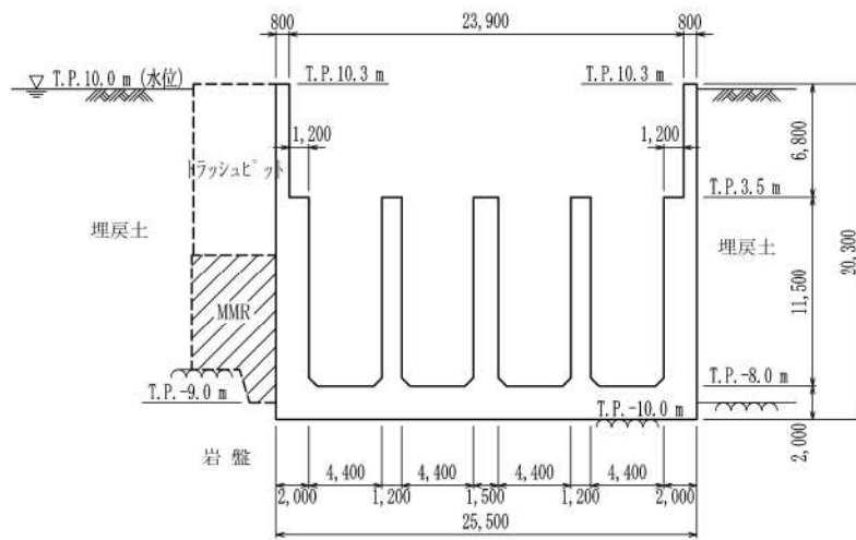
第 8-2-6-4 図 取水ピットスクリーン室 断面図 (B-B 断面)
