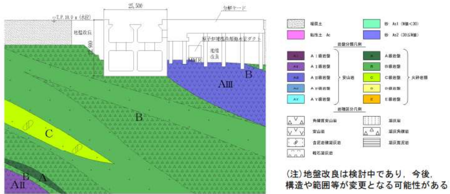
第 8-2-7-9 図 取水ピットポンプ室 地質断面図 (B-B 断面)
