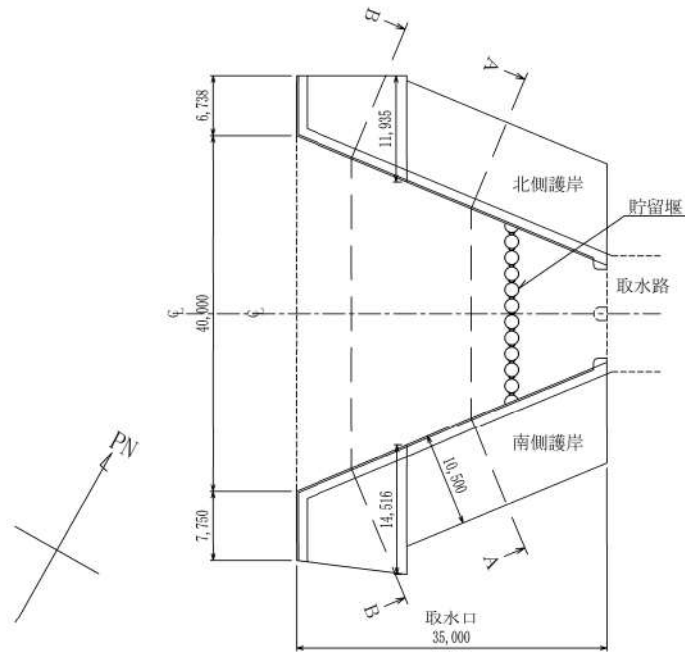
参考 1-1 図 取水口 平面図
