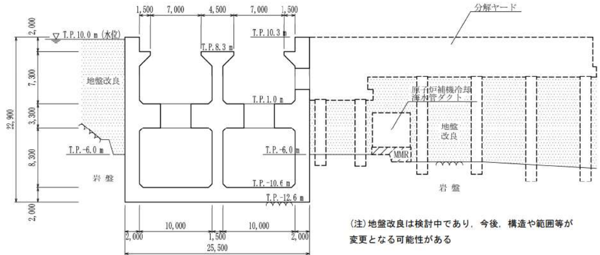
第6-56図 取水ピットポンプ室 断面図 (B-B 断面)
