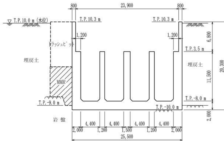
第6-46図 取水ピットスクリーン室 断面図 (B-B断面)
