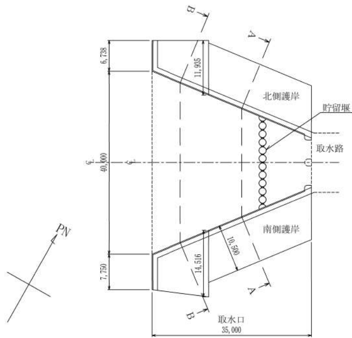
第8-2-2-2図 取水口 平面図
