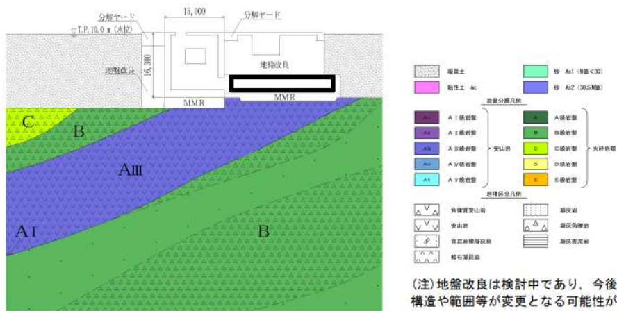
第 8-2-8-7 図 原子炉補機冷却海水ポンプ出口ストレーナ室 地質断面図 (C-C 断面)
