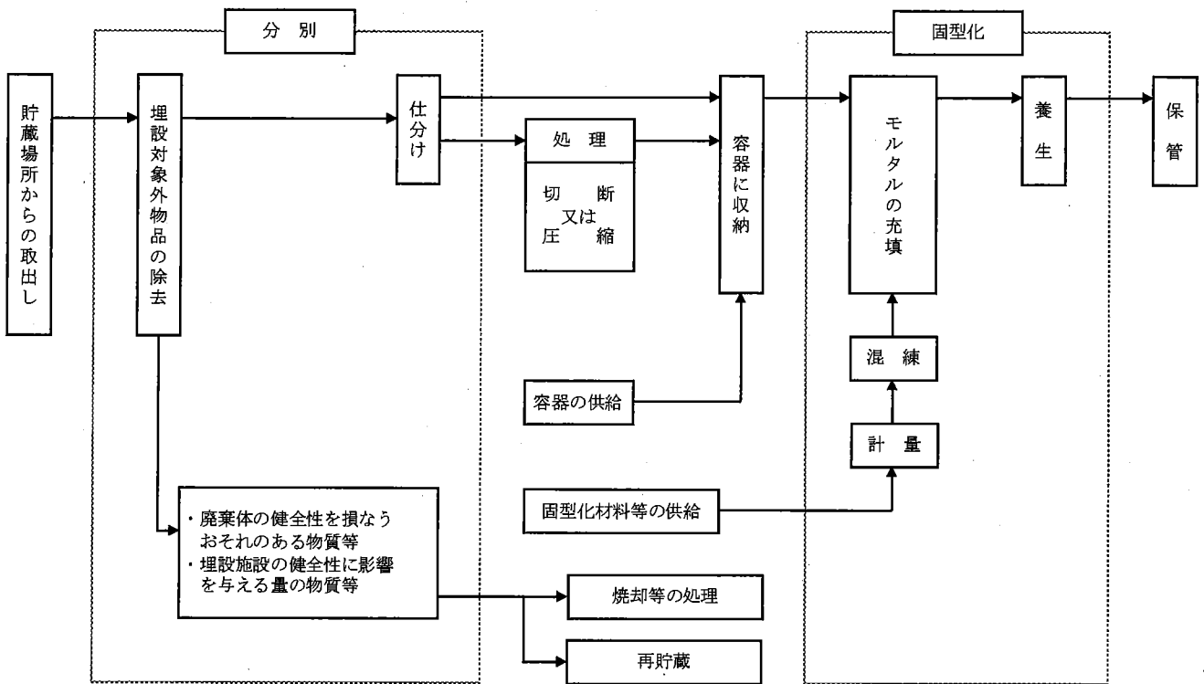
図-1 廃棄体製作の基本フロー
