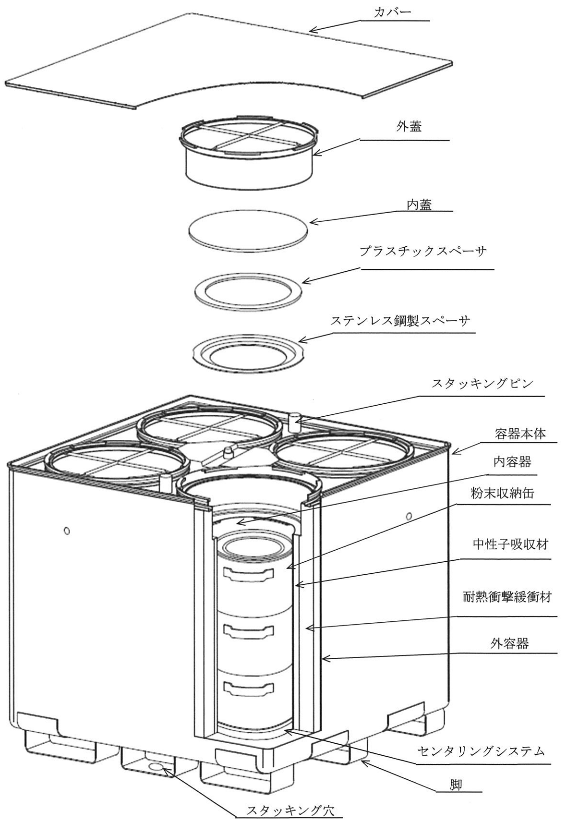
図1 TNF·XI型輸送物外観図
