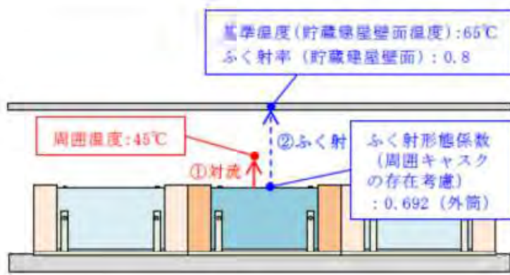
型式指定(貯蔵建屋内貯蔵)
