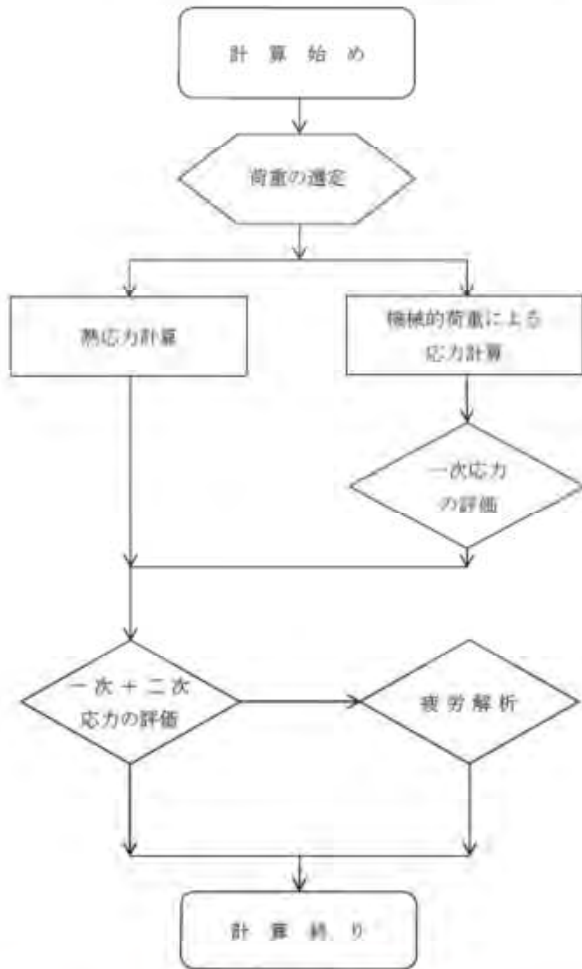
トラニオンの評価フロー
