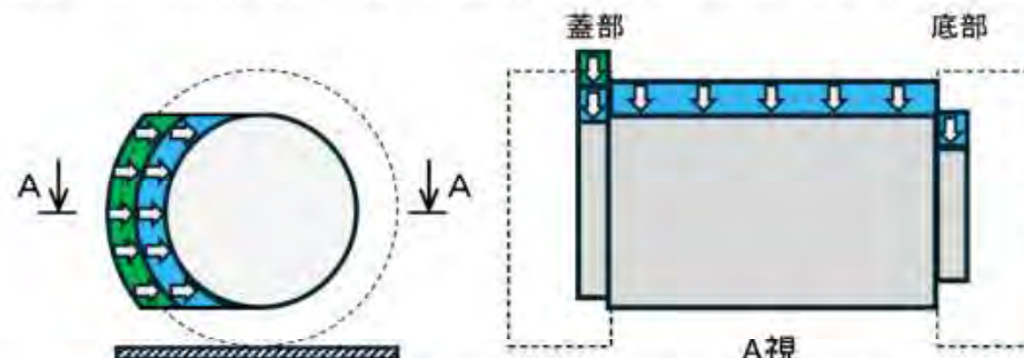
(2) MSF-24P(S)型の径方向衝突時
