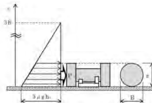
(1) MSF-24P(S)型の軸方向衝突時
