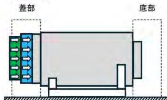
(1) MSF-24P(S)型の軸方向衝突時
