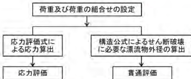
外筒の評価フロー
