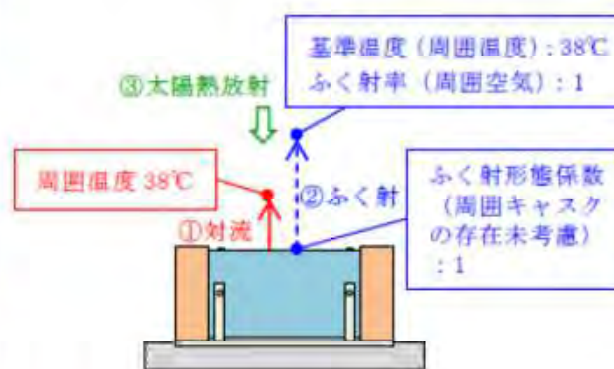
型式証明(屋外貯蔵[評価代表例])
