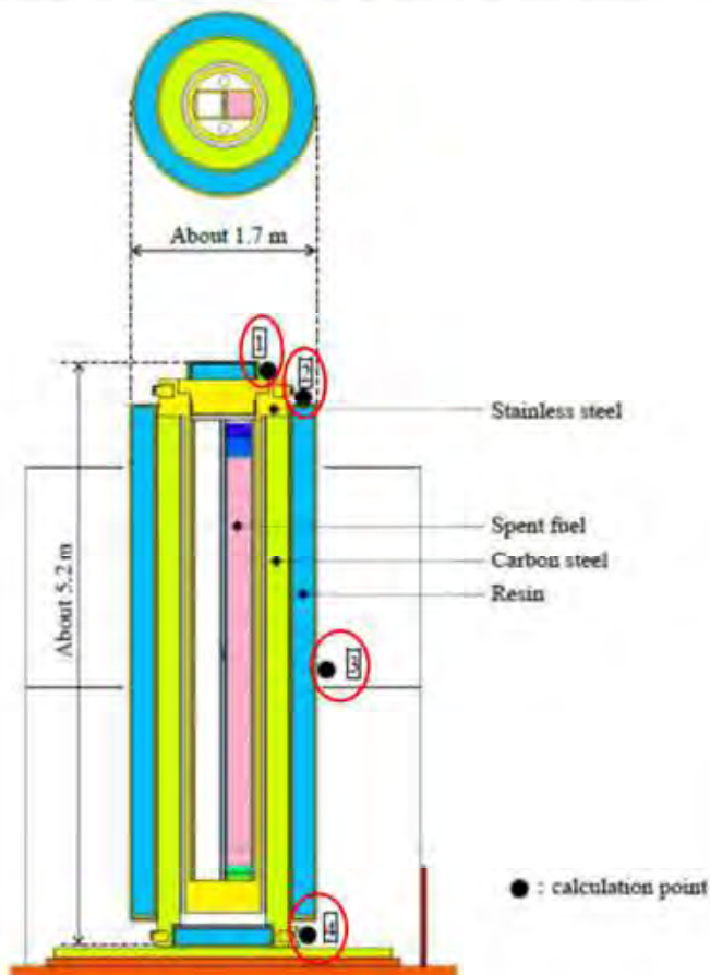
(解析モデル)
