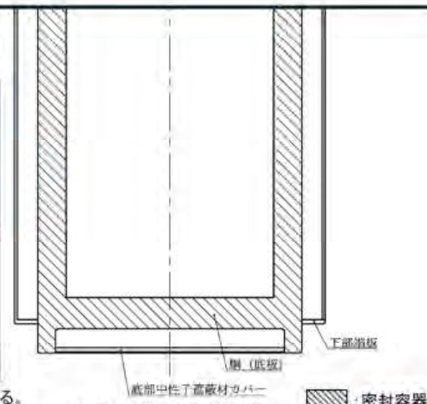
密封容器の評価箇所
