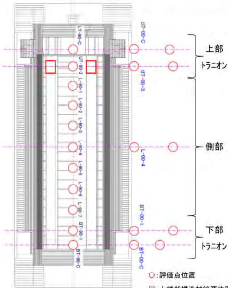
(解析モデル)
