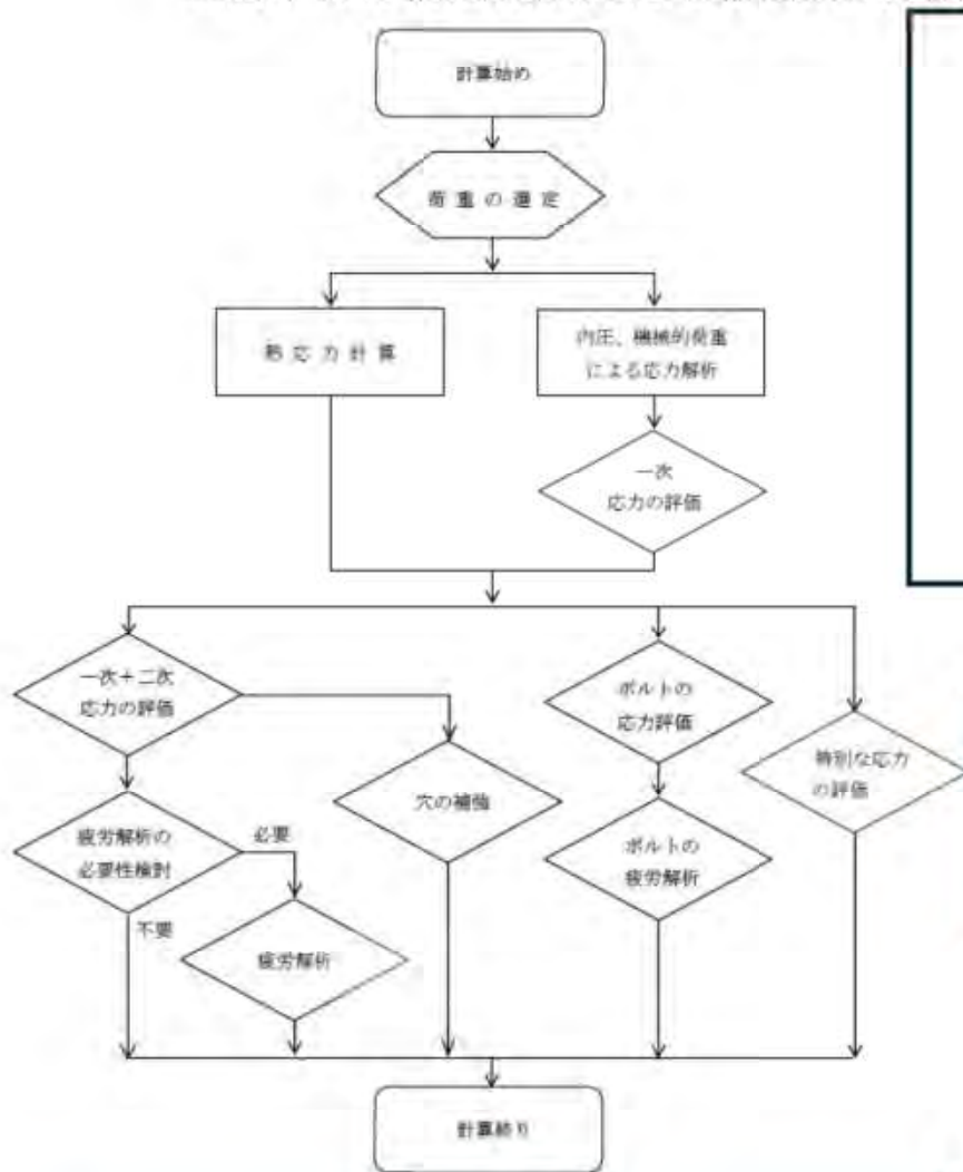
密封容器の評価フロー
