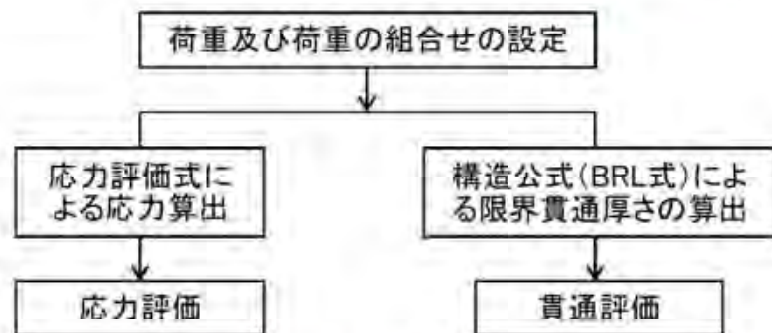
外筒の評価フロー
