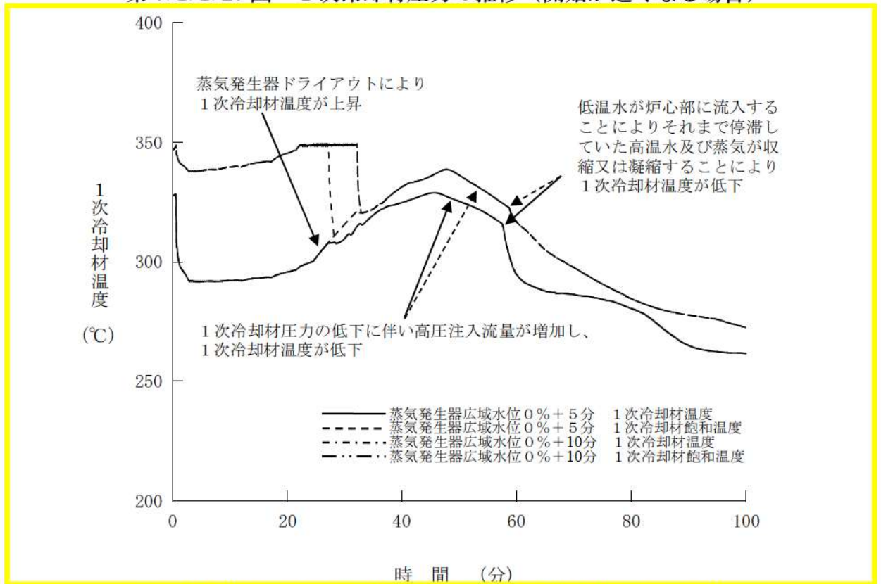
第 7.1.1.28 図 1次冷却材温度の推移 (開始が遅くなる場合)
