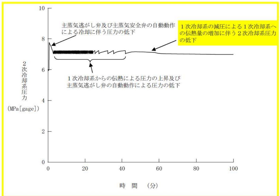
第 7. 1. 1. 15 図 2次冷却系圧力の推移
