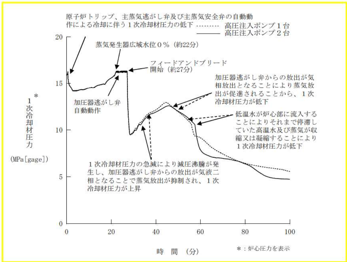
図2 1次冷却材圧力の推移
