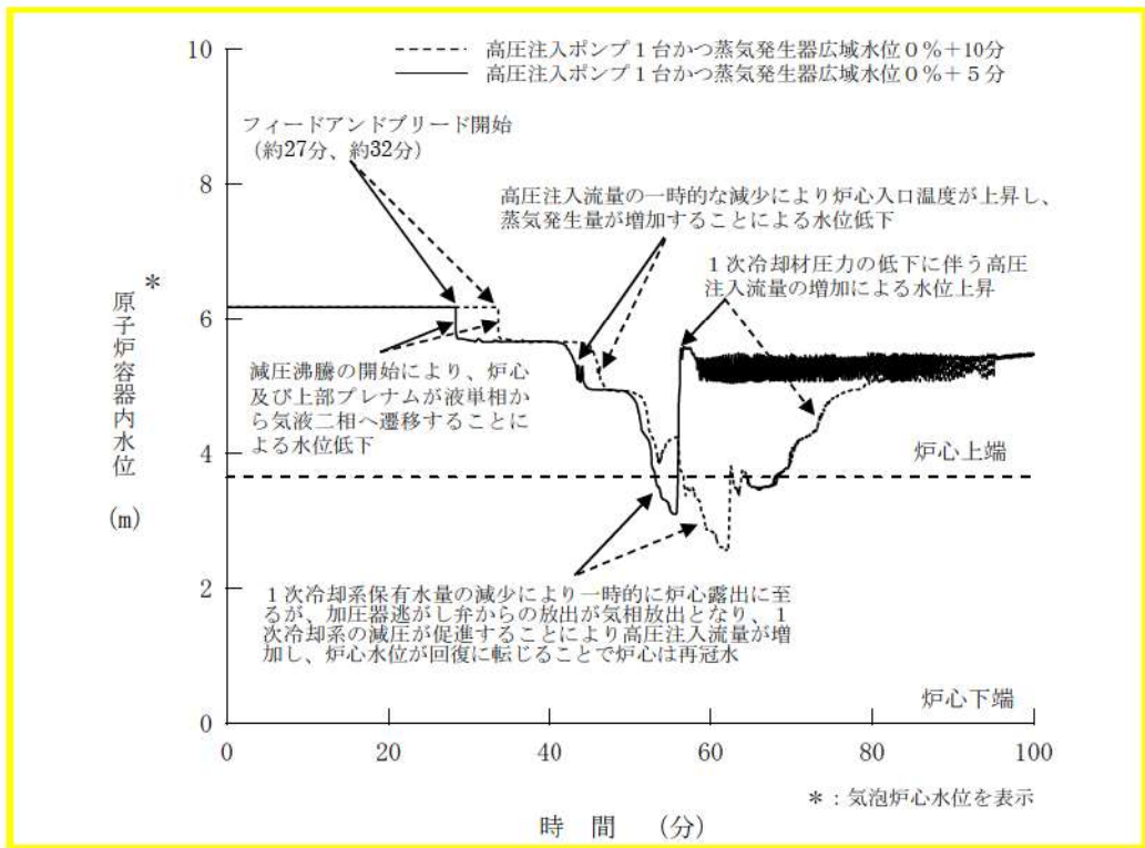
参考図5 原子炉容器内水位の推移 (感度ケース2)
