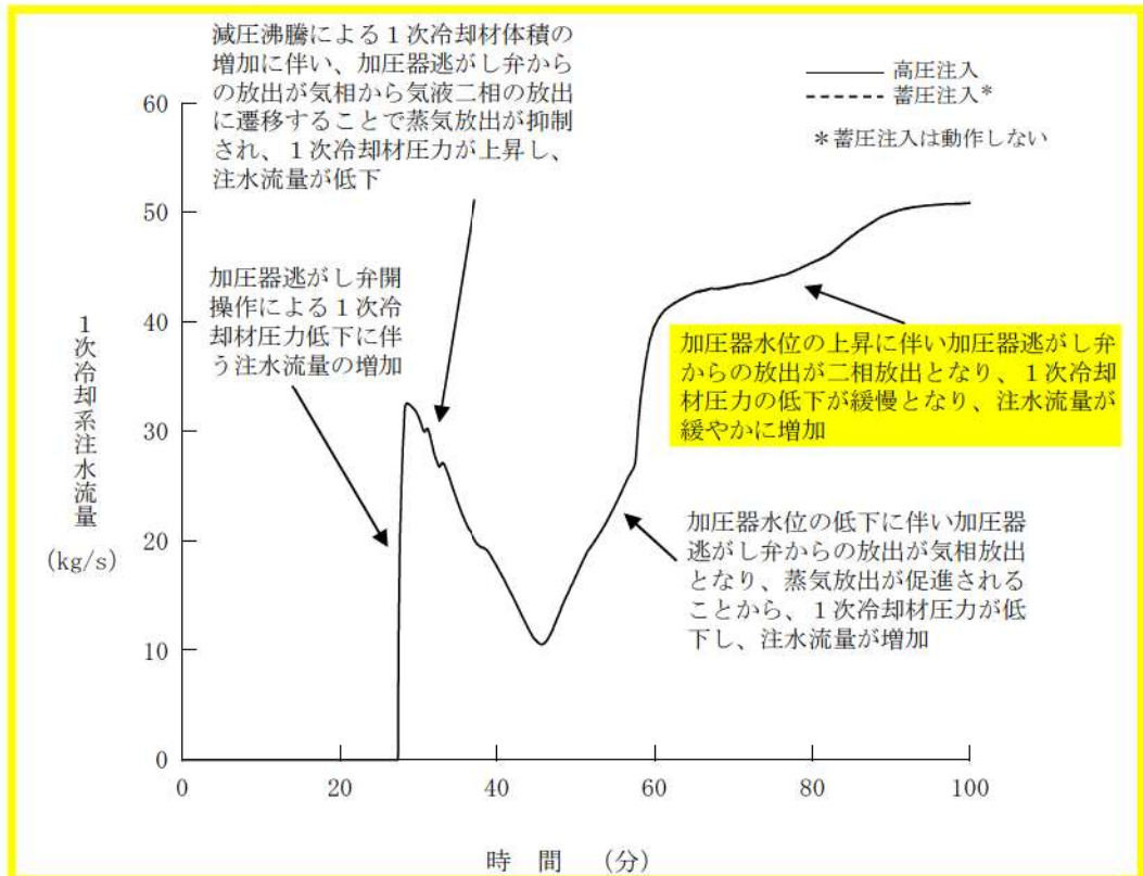
第 7.1.1.10 図 1次冷却系注水流量の推移
