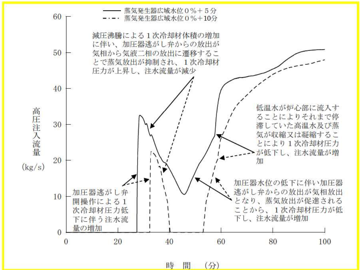
第 7.1.1.29 図 高圧注入流量の推移（開始が遅くなる場合）
