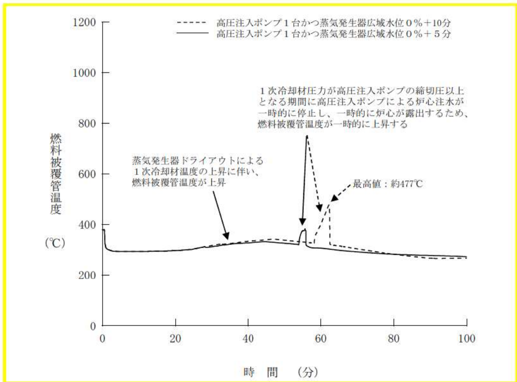
参考図6 燃料被覆管温度の推移 (感度ケース2)
