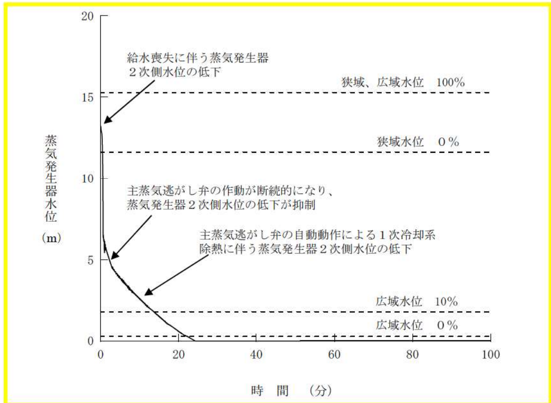
第 7. 1. 1. 14 図 蒸気発生器水位の推移
