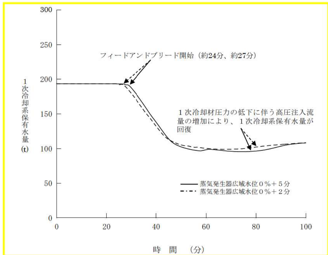
第 7.1.1.24 図 1次冷却系保有水量の推移（開始が早くなる場合）
