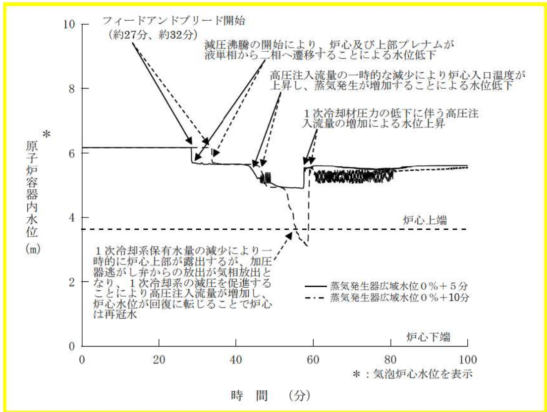
第 7.1.1.31 図 原子炉容器内水位の推移（開始が遅くなる場合）
