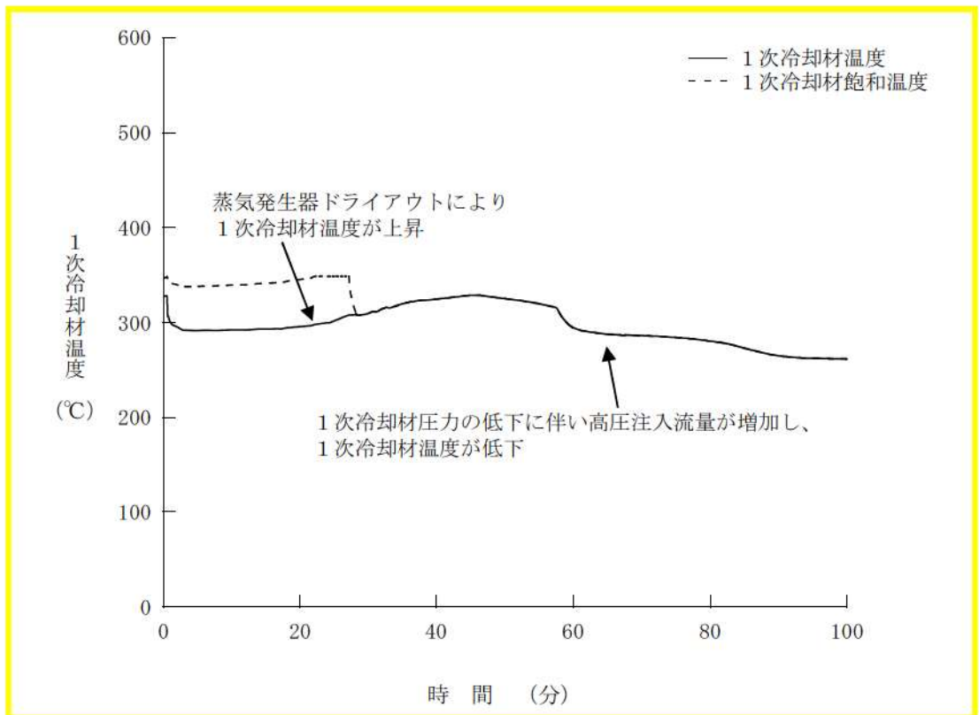
第 7. 1. 1. 13 図 1次冷却材温度の推移
