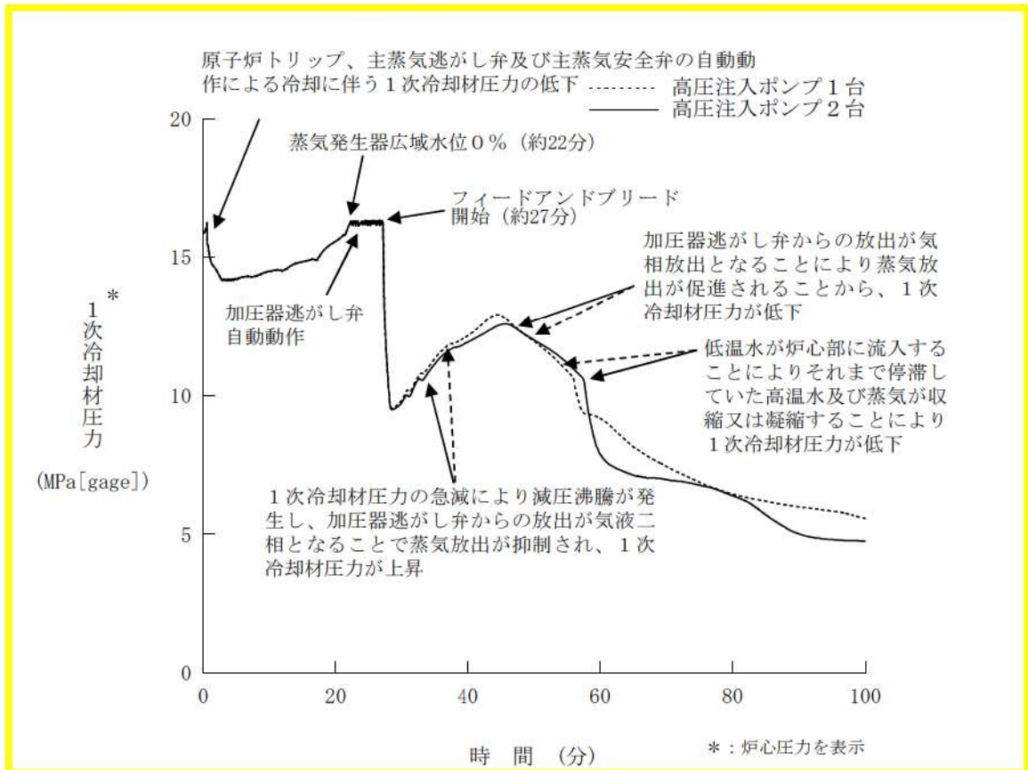
第 7.1.1.16 図 1次冷却材圧力の推移 (高圧注入ポンプ1台の場合)
