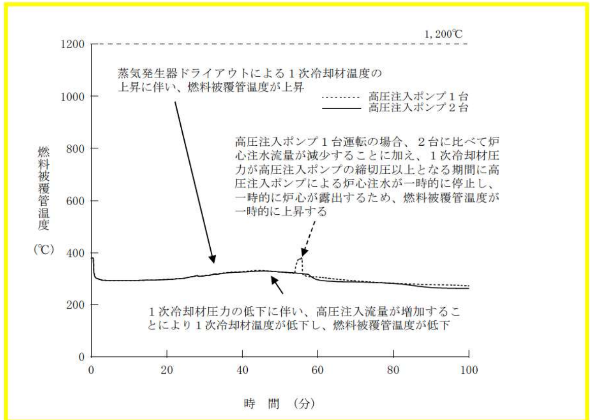
第 7.1.1.20 図 燃料被覆管温度の推移（高圧注入ポンプ1台の場合）
