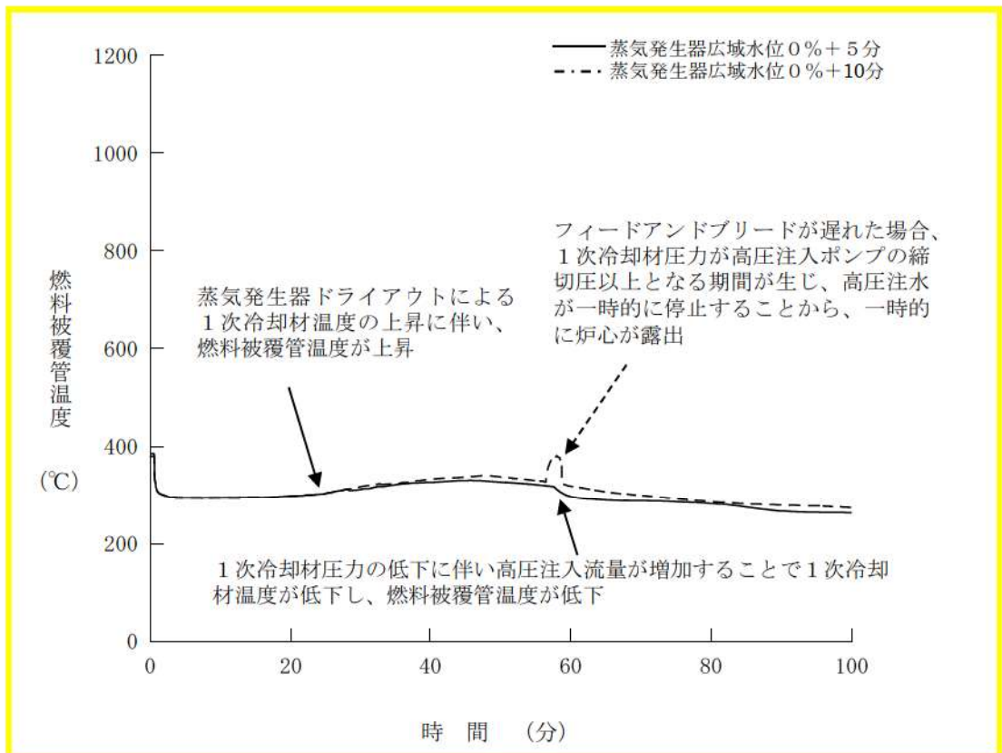
第 7.1.1.32 図 燃料被覆管温度の推移（開始が遅くなる場合）
