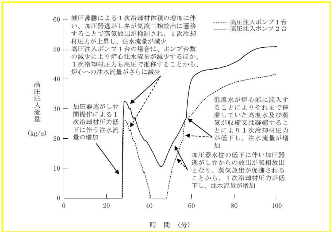
図3 高圧注入流量の推移
