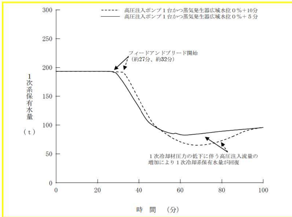
参考図3 1次系保有水量の推移 (感度ケース2)
