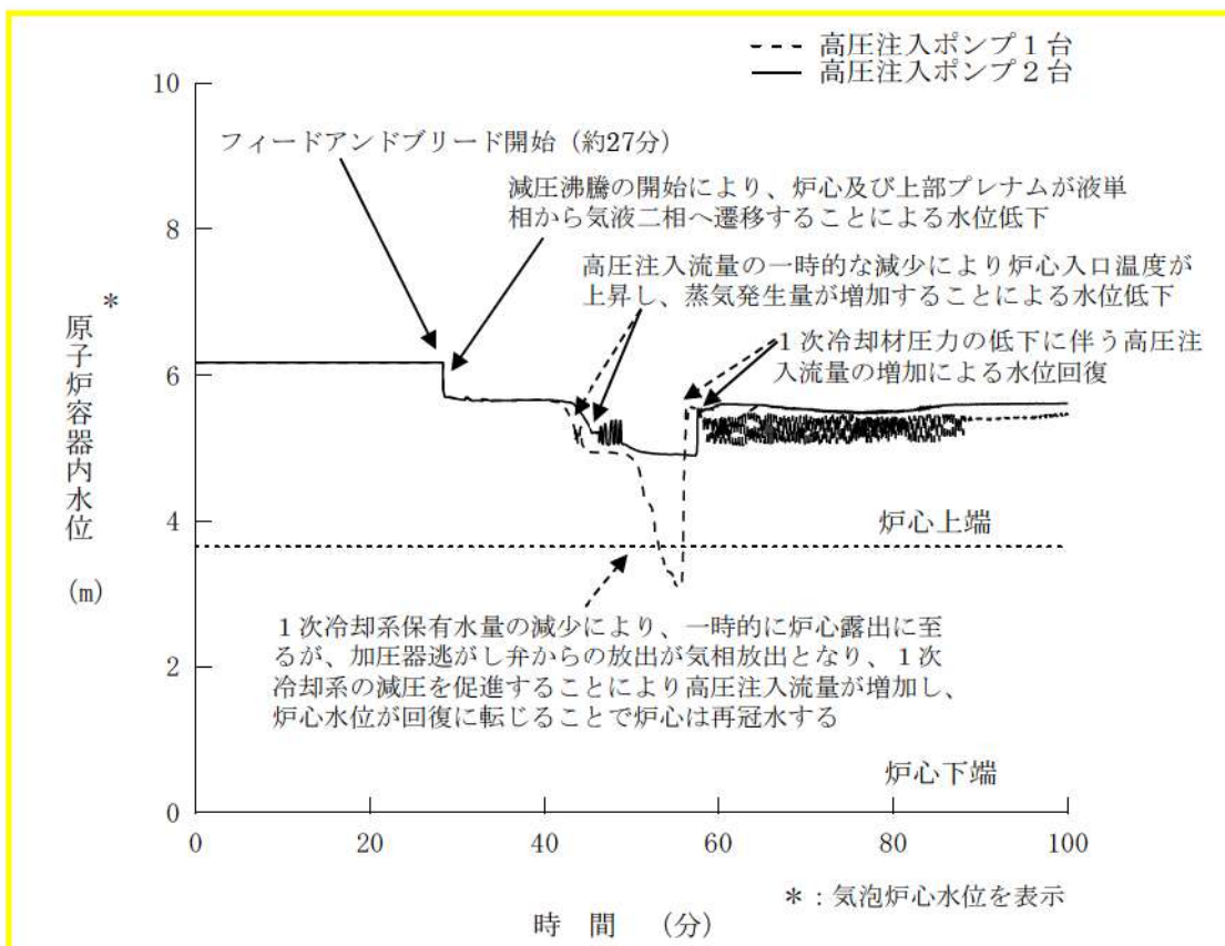
図7 原子炉容器内水位の推移
