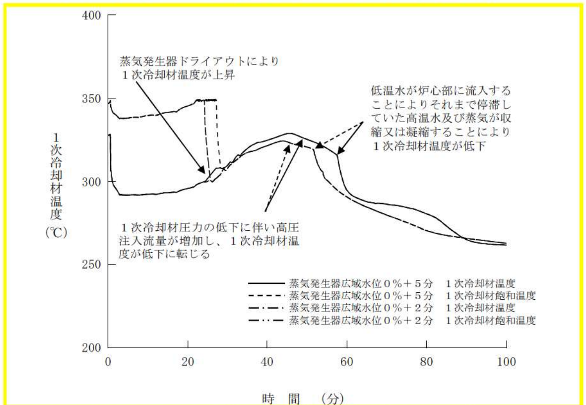
第7.1.1.22図 1次冷却材温度の推移 (開始が早くなる場合)
