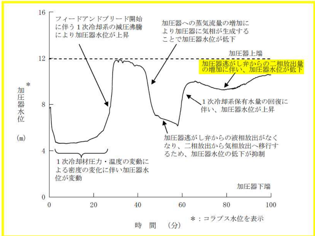
第 7.1.1.6 図 加圧器水位の推移
