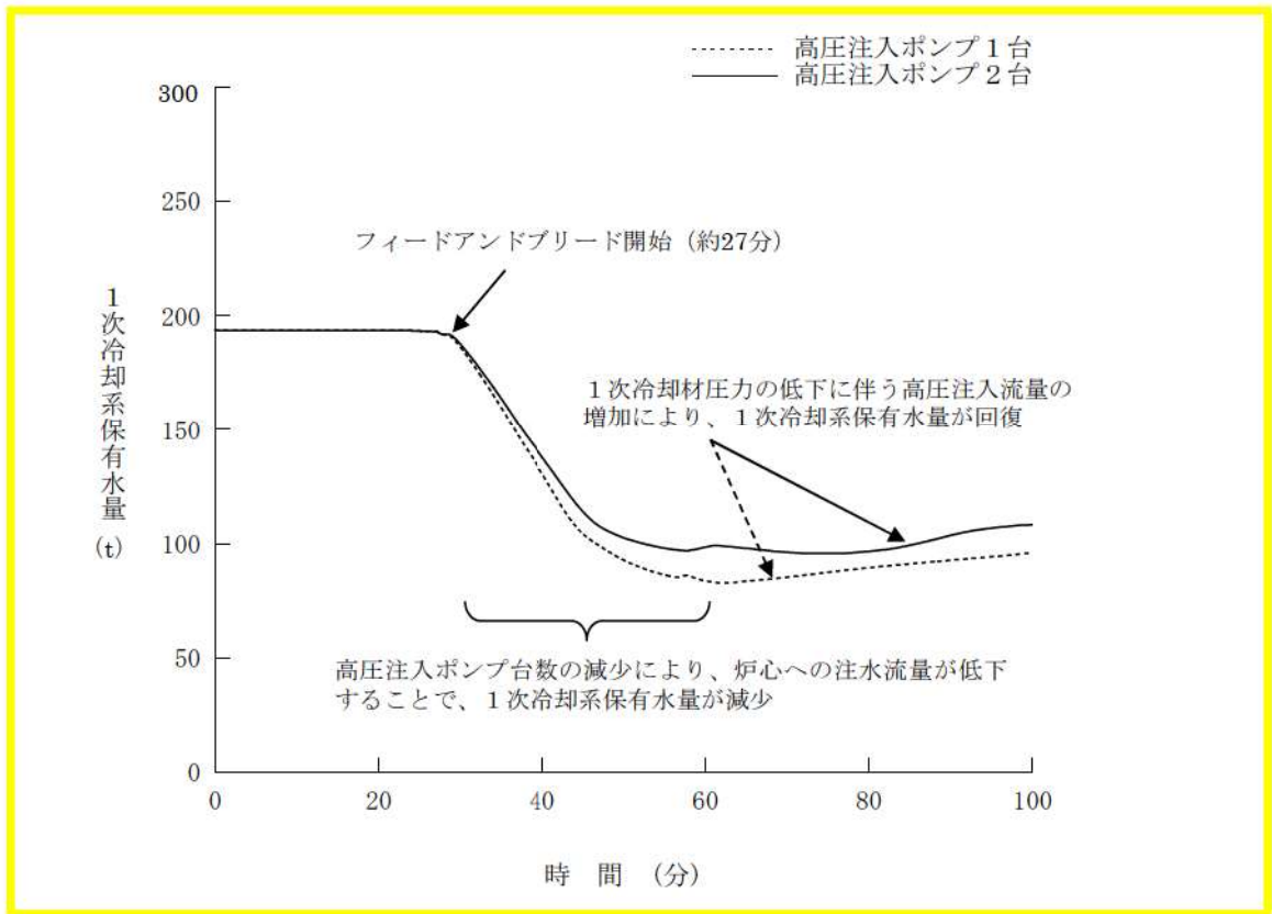
第 7. 1. 1. 18 図 1 次冷却系保有水量の推移 (高圧注入ポンプ 1 台の場合)
