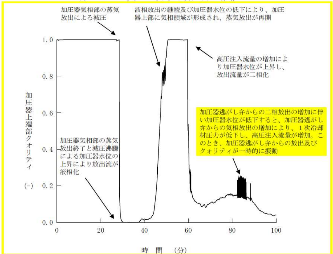
第 7.1.1.5 図 加圧器上端部クオリティの推移
