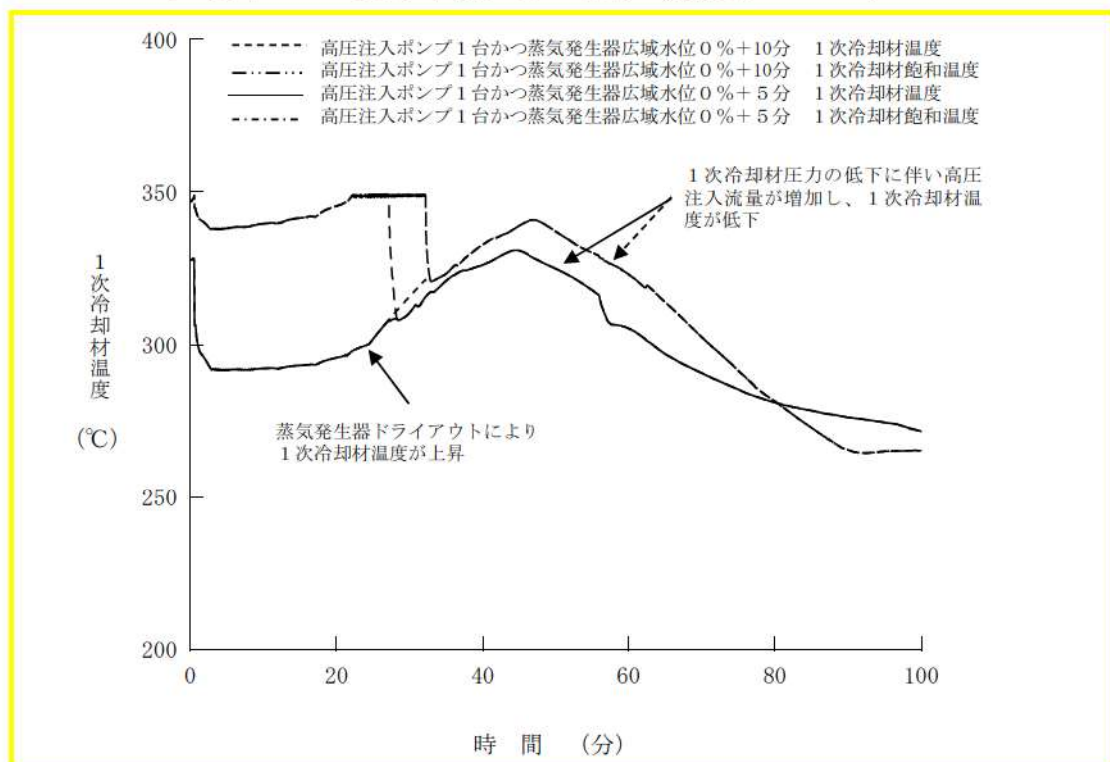
参考図2 1次冷却材温度の推移 (感度ケース2)
