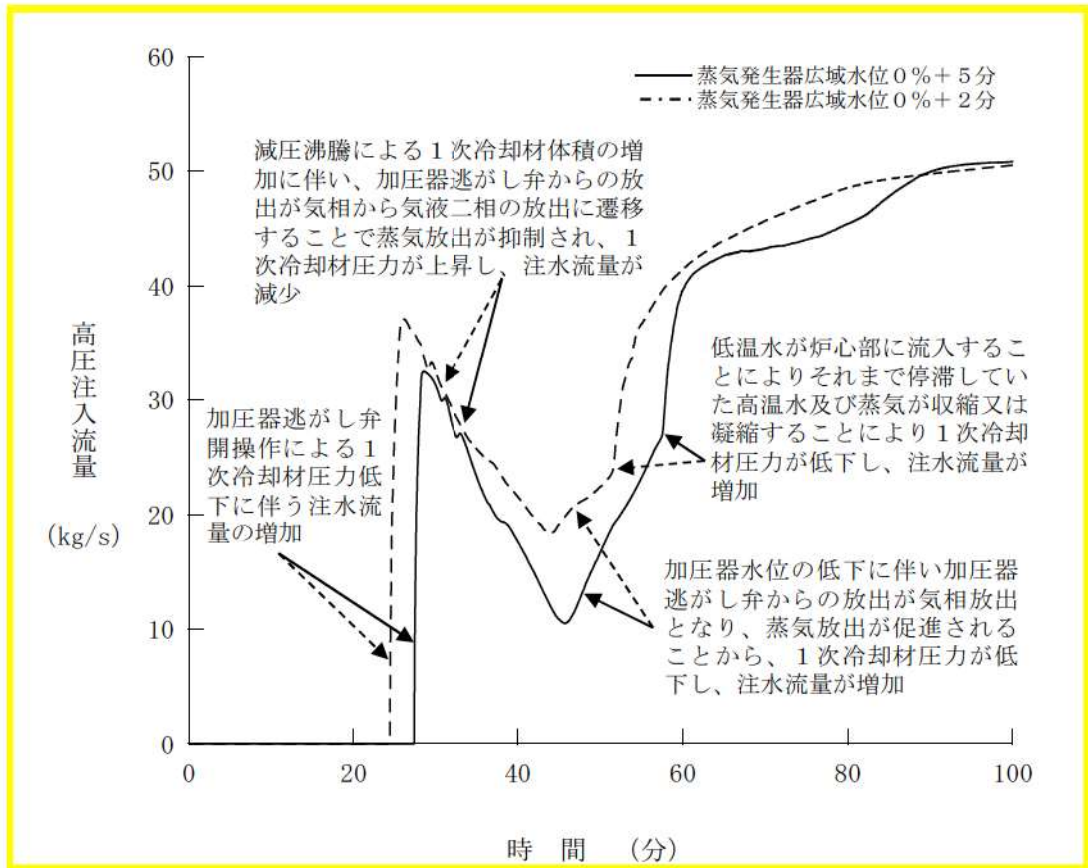
第 7.1.1.23 図 高圧注入流量の推移（開始が早くなる場合）
