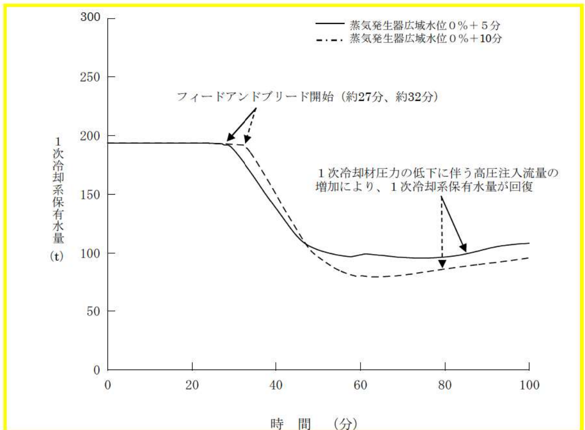
第 7.1.1.30 図 1次冷却系保有水量の推移（開始が遅くなる場合）
