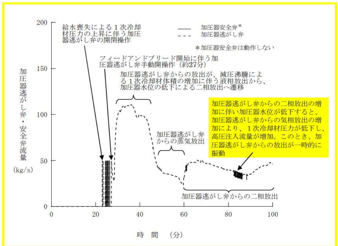
第 7.1.1.11 図 加圧器逃がし弁・安全弁流量の推移
