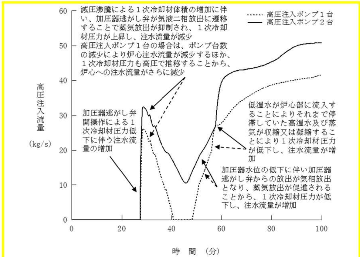
第 7.1.1.17 図 高圧注入流量の推移 (高圧注入ポンプ1台の場合)
