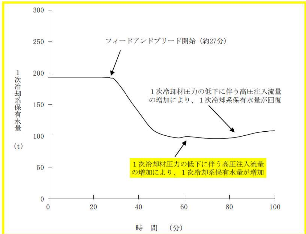
第 7.1.1.8 図 1次冷却系保有水量の推移
