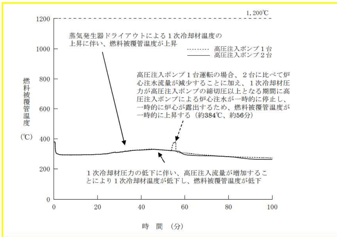
図6 燃料被覆管温度の推移
