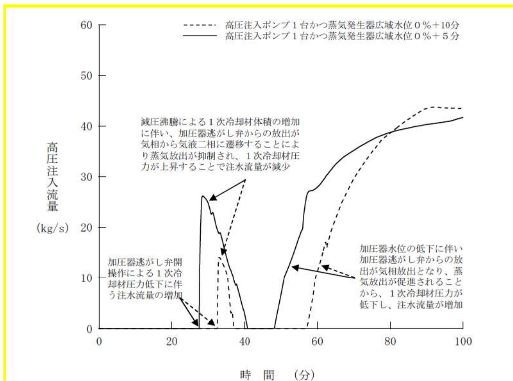
参考図4 高圧注入流量の推移 (感度ケース2)
