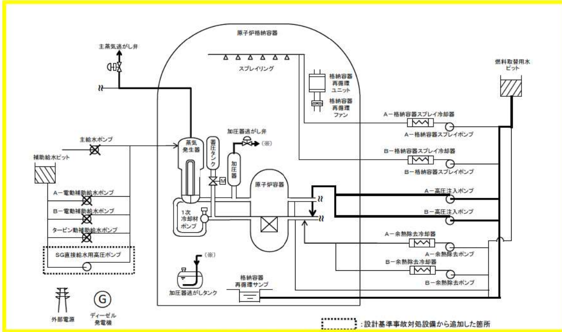
図1 「主給水流量喪失時に補助給水機能が喪失する事故」の重大事故等対策の概略系統図 (フィードアンドブリード及び高压再循環)
