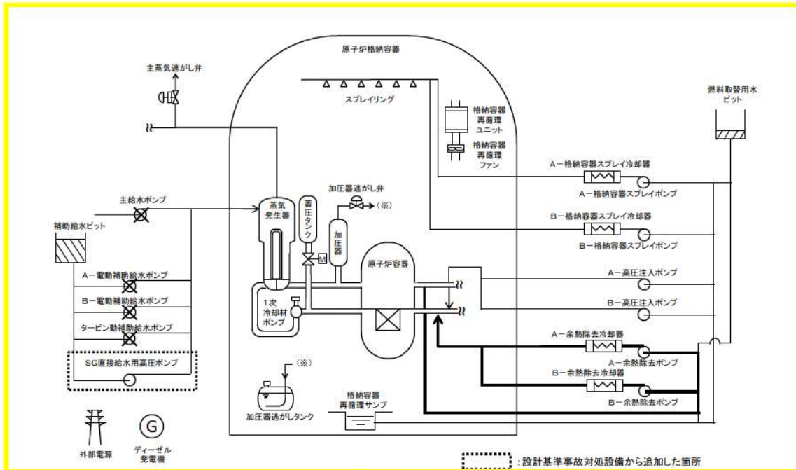
図2 「主給水流量喪失時に補助給水機能が喪失する事故」の重大事故等対策の概略系統図 (余熱除去系による炉心冷却)
