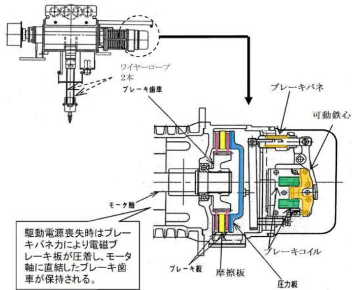
電磁ブレーキ構造図
