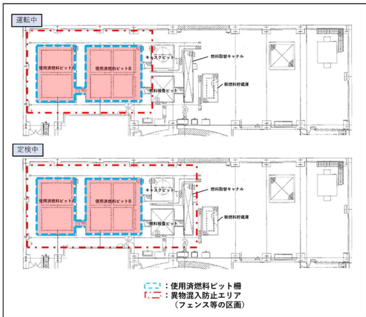
図 1 燃料取扱棟 異物混入防止エリア設定概要 (運転中・点検中)
