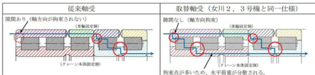
図 2 女川原子力発電所 1号炉 従来軸受と取替軸受の比較 (平成 25 年 11 月 21 日 東北電力株式会社プレス資料から抜粋)
