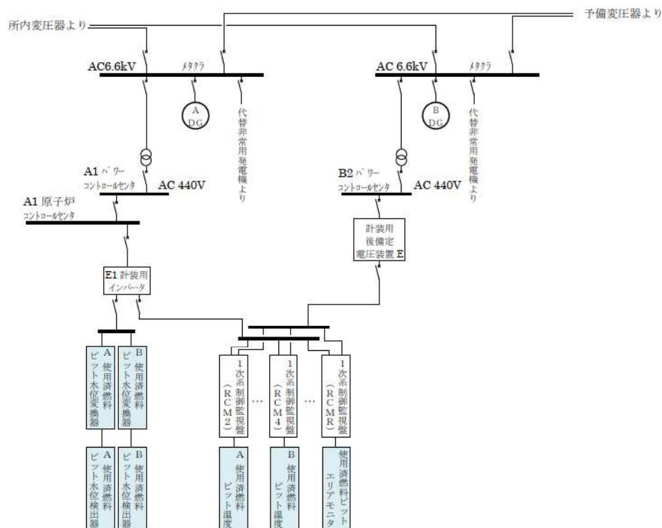
図 1.4.1 使用済燃料ピット監視設備（設計基準対象施設）の電源構成
