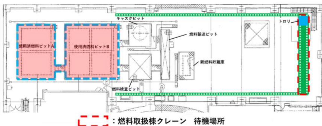
図2 燃料取扱棟クレーン 待機場所
