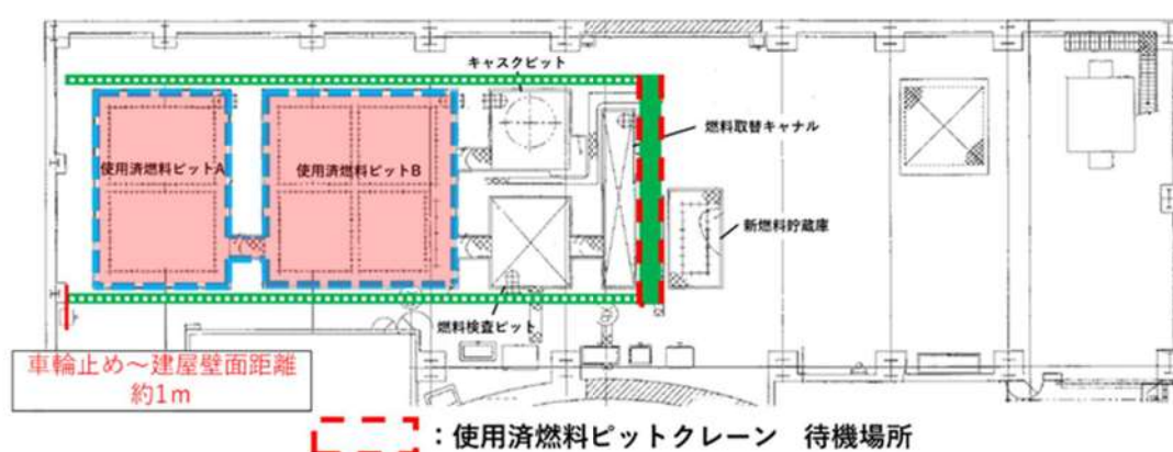
図 1 使用済燃料ピットクレーン走行レールと壁面距離
