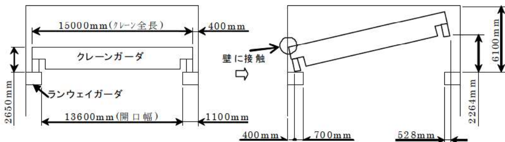
鉛直移動した場合の寸法図
