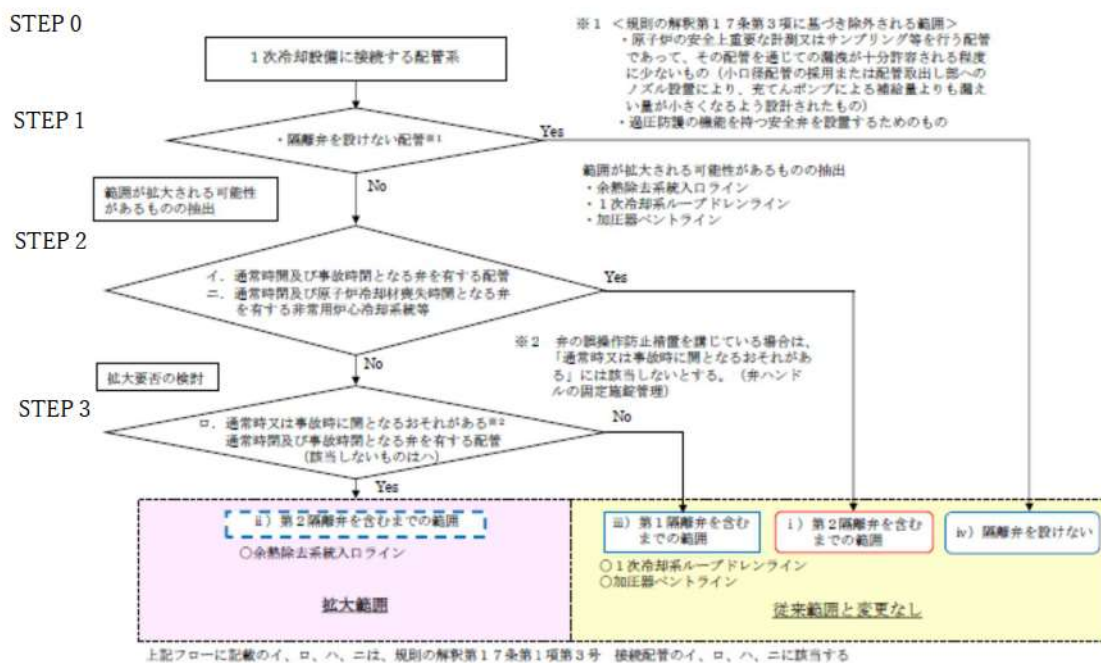
原子炉冷却材圧力バウンダリ抽出フロー
