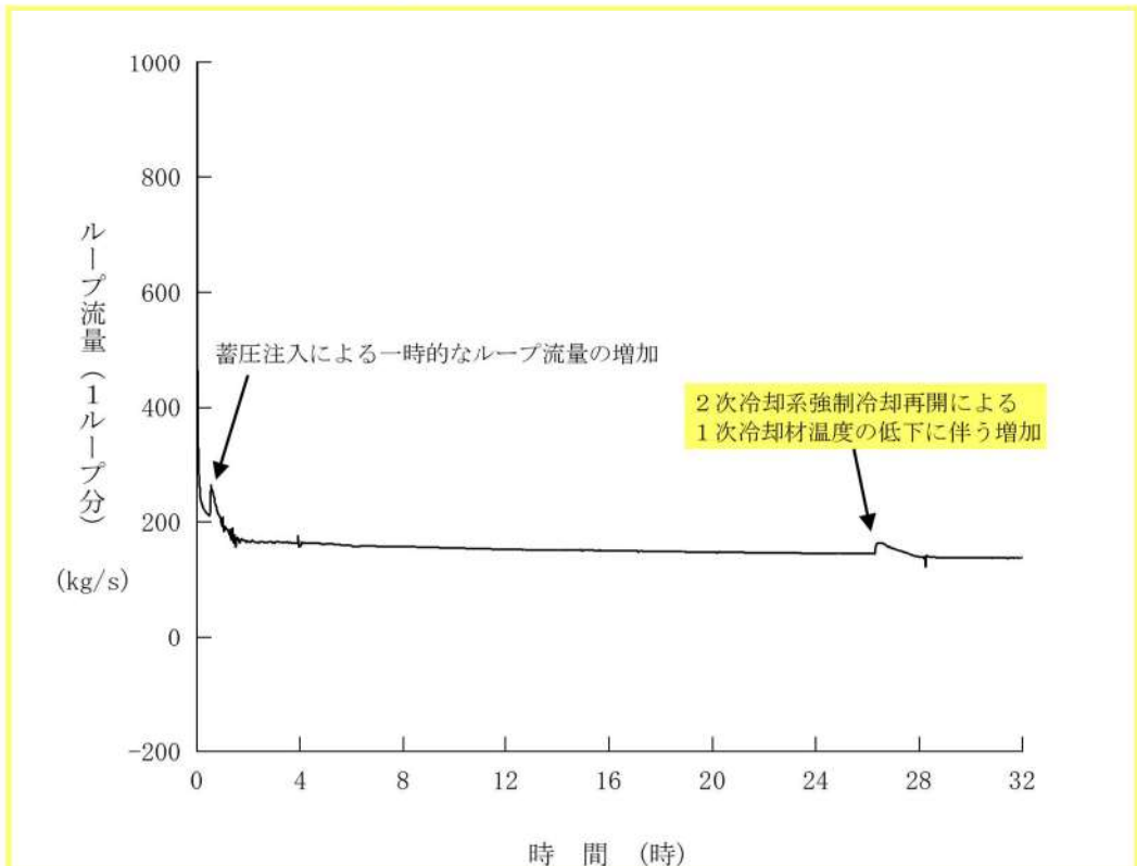
第 7.1.2.32 図 1 次冷却材流量の推移 (RCP シール LOCA が発生しない場合)
