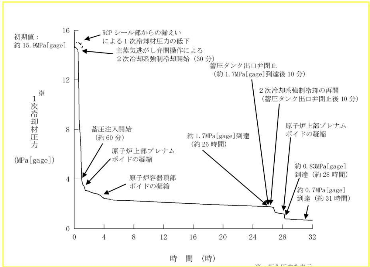
第 7.1.2.27 図 1次冷却材圧力の推移 (RCP シール LOCA が発生しない場合)
