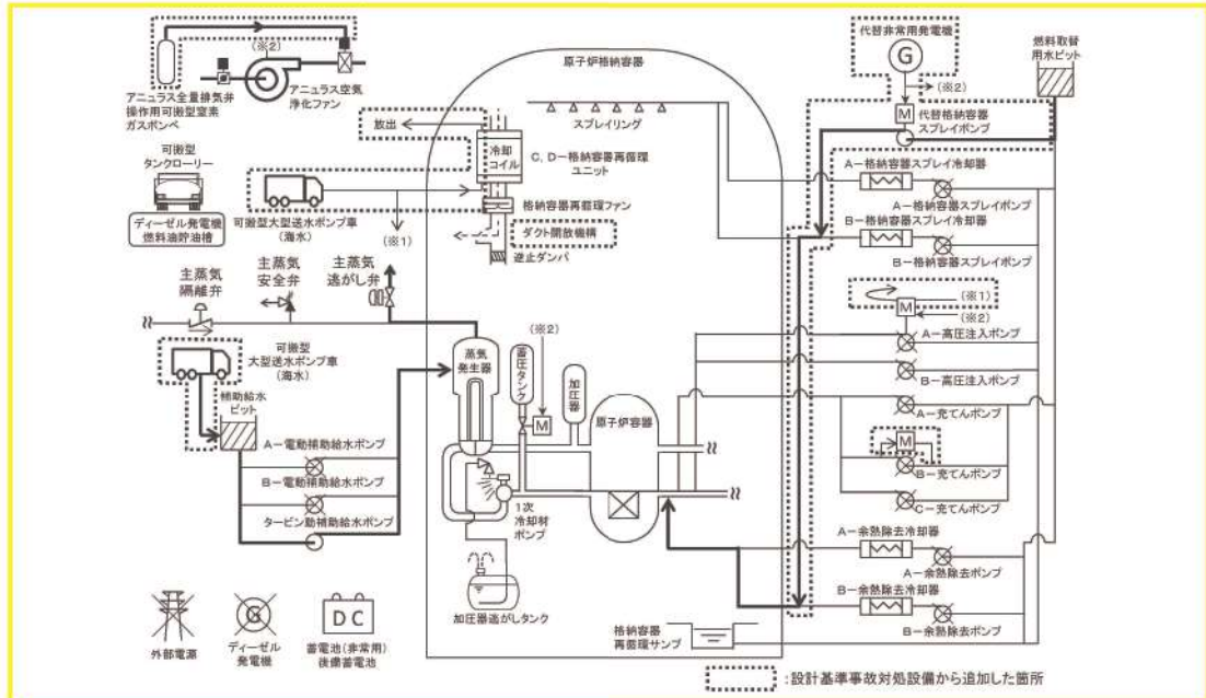
図 1 「外部電源喪失時に非常用所内交流電源が喪失し、原子炉補機冷却機能の喪失及びRCPシールLOCAが発生する事故」の重大事故等対策の概略系統図 (2次系強制冷却及び代替炉心注水)
