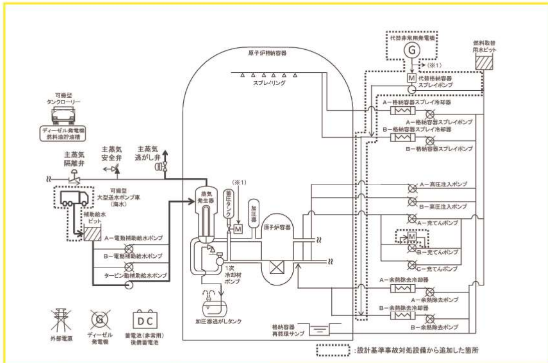
図 3 「外部電源喪失時に非常用所内交流電源が喪失し、原子炉補機冷却機能の喪失する事故」の重大事故等対策の概略系統図 (2次系強制冷却)
