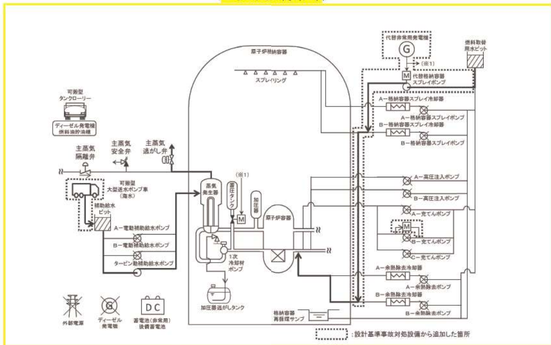
図 4 「外部電源喪失時に非常用所内交流電源が喪失し、原子炉補機冷却機能の喪失する事故」の重大事故等対策の概略系統図 (2次系強制冷却及び代替炉心注水)
