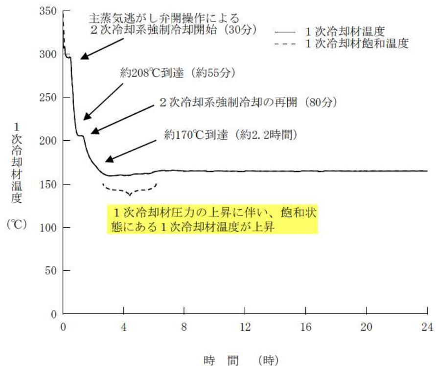
第 7. 1. 2. 7 図 1次冷却材温度の推移 (RCP シール LOCA が発生する場合)
