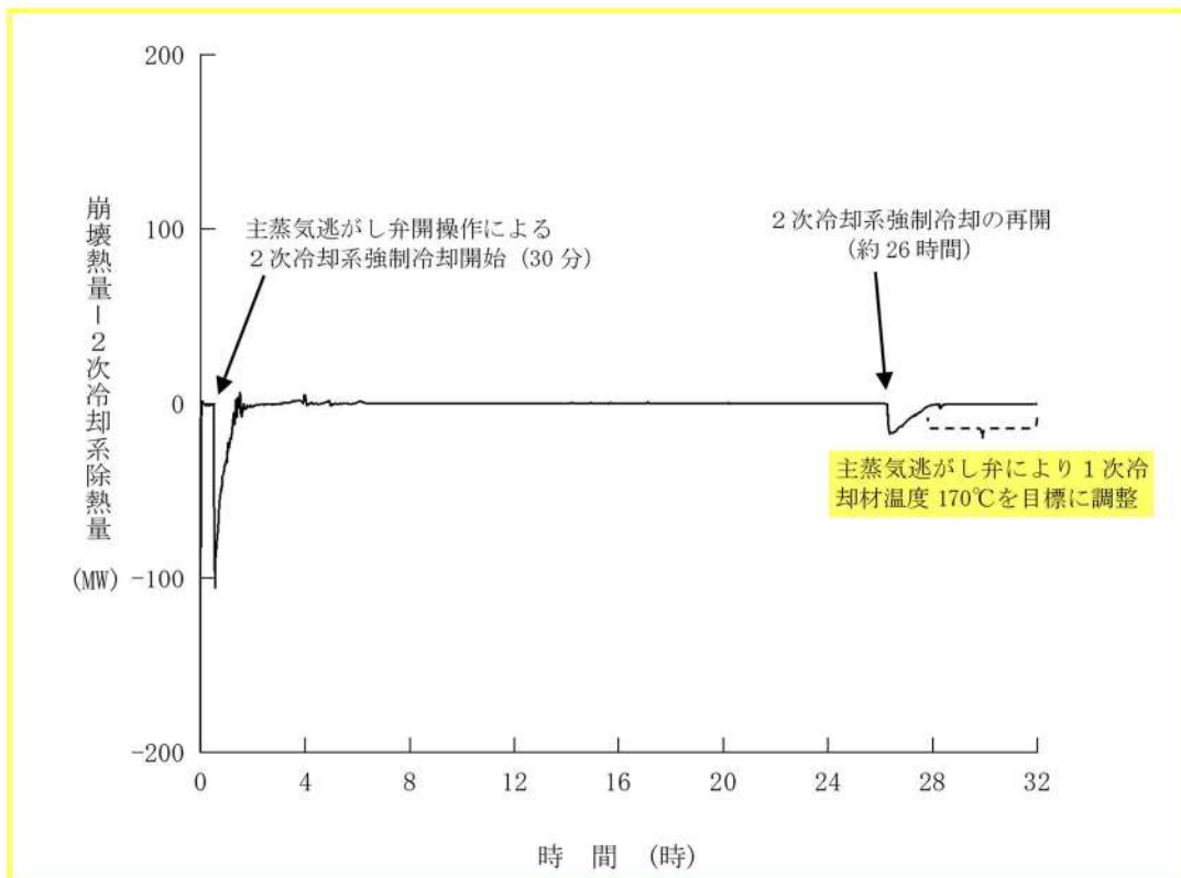
第7.1.2.41図 崩壊熱量と2次冷却系除熱量の推移 (RCP シール LOCA が発生しない場合)
