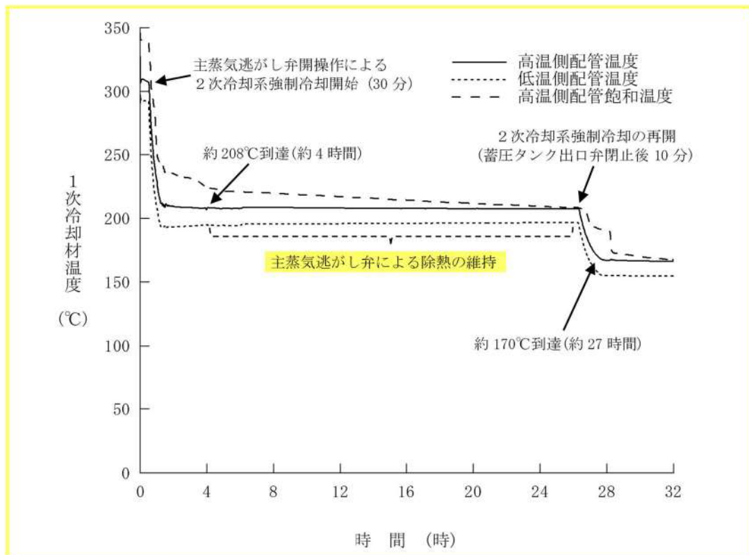
第 7.1.2.28 図 1次冷却材温度の推移 (RCP シール LOCA が発生しない場合)
