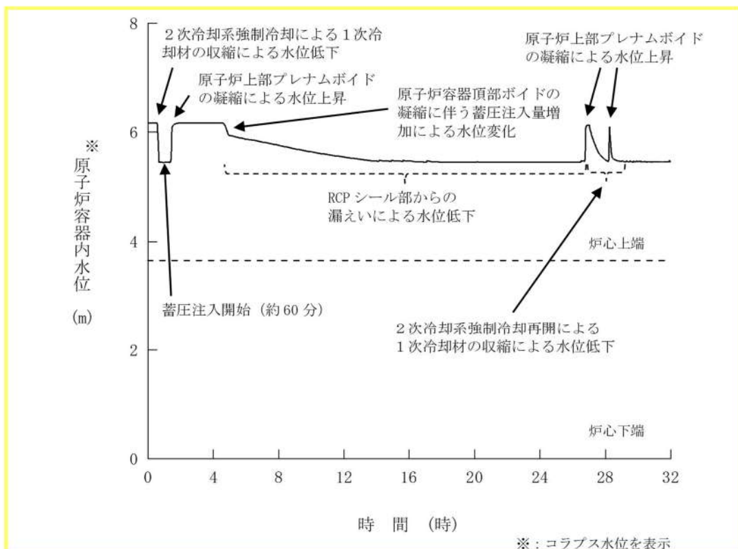
第 7.1.2.34 図 原子炉容器内水位の推移 (RCP シール LOCA が発生しない場合)
