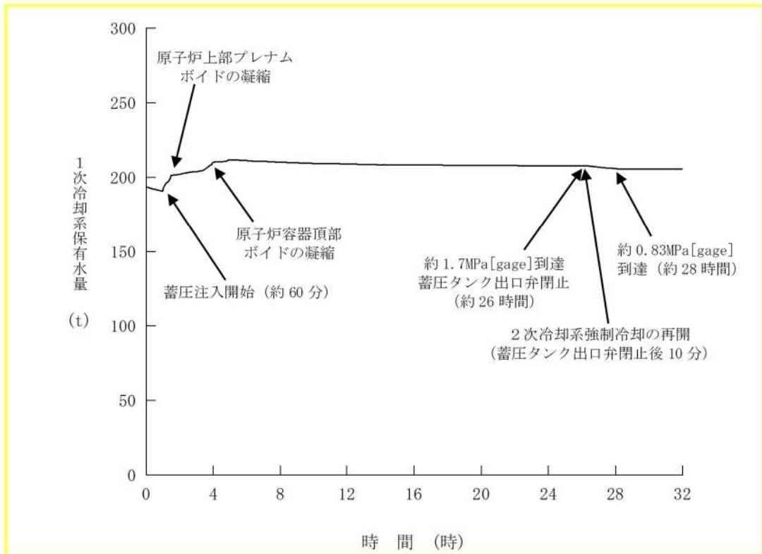
第 7. 1. 2. 29 図 1 次冷却系保有水量の推移 (RCP シール LOCA が発生しない場合)
