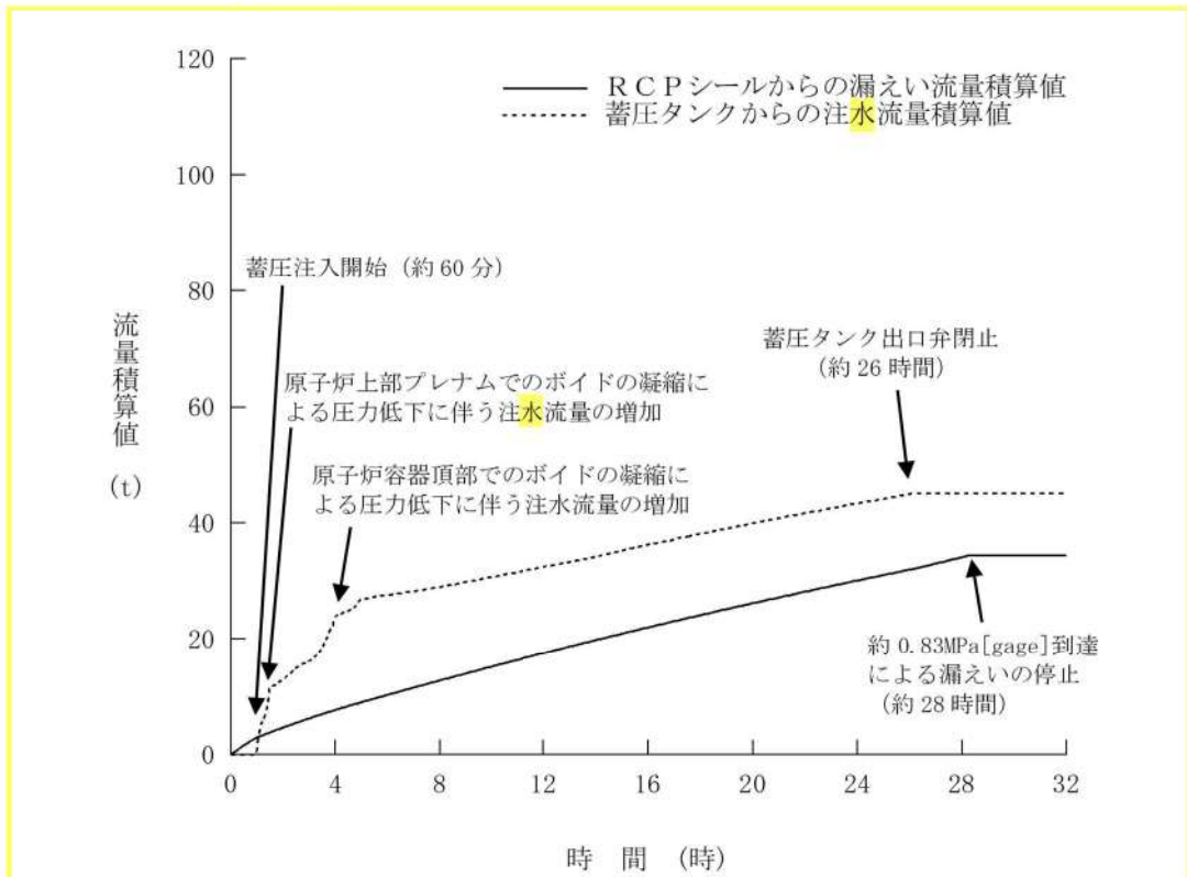
第 7. 1. 2. 30 図 漏えい流量と注水流量の積算値の推移 (RCP シール LOCA が発生しない場合)
