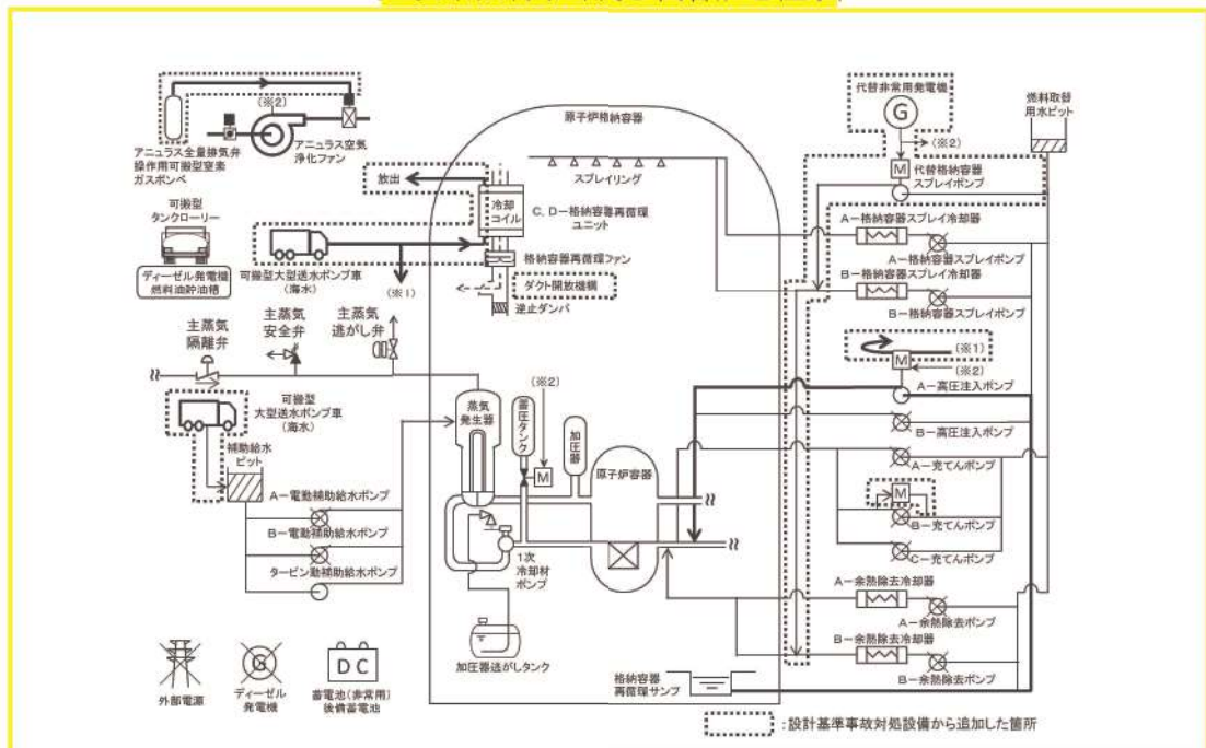
図 2 「外部電源喪失時に非常用所内交流電源が喪失し、原子炉補機冷却機能の喪失及びRCPシールLOCAが発生する事故」の重大事故等対策の概略系統図 (格納容器内自然対流冷却及び高圧代替再循環)
