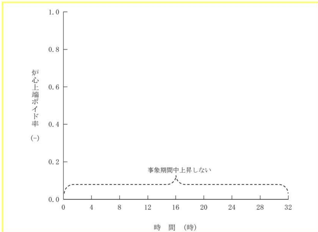
第 7.1.2.33 図 炉心上端ボイド率の推移 (RCP シール LOCA が発生しない場合)
