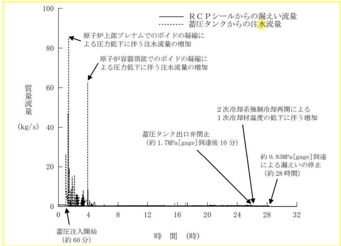
第 7.1.2.31 図 漏えい流量と注水流量の推移 (RCP シール LOCA が発生しない場合)
