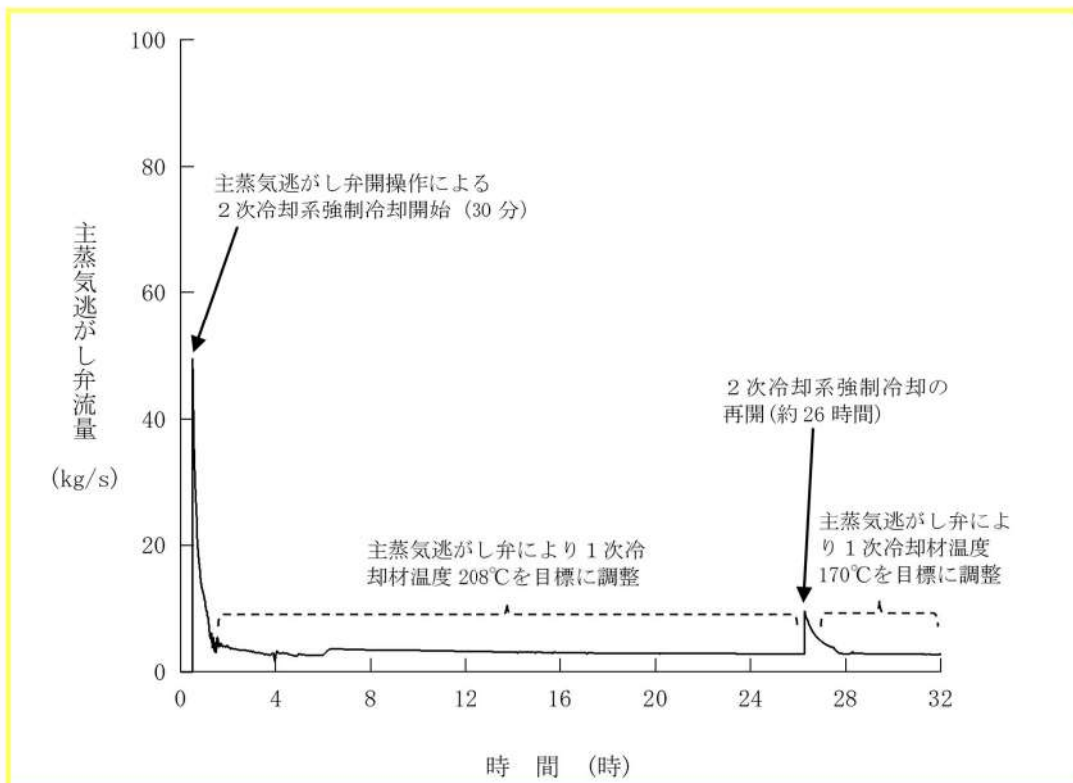
第 7. 1. 2. 37 図 主蒸気逃がし弁流量の推移 (RCP シール LOCA が発生しない場合)
