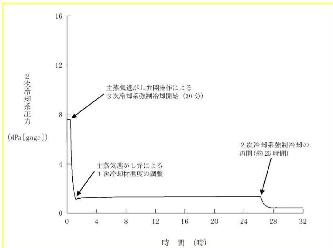
第 7. 1. 2. 36 図 2次冷却系圧力の推移 (RCP シール LOCA が発生しない場合)
