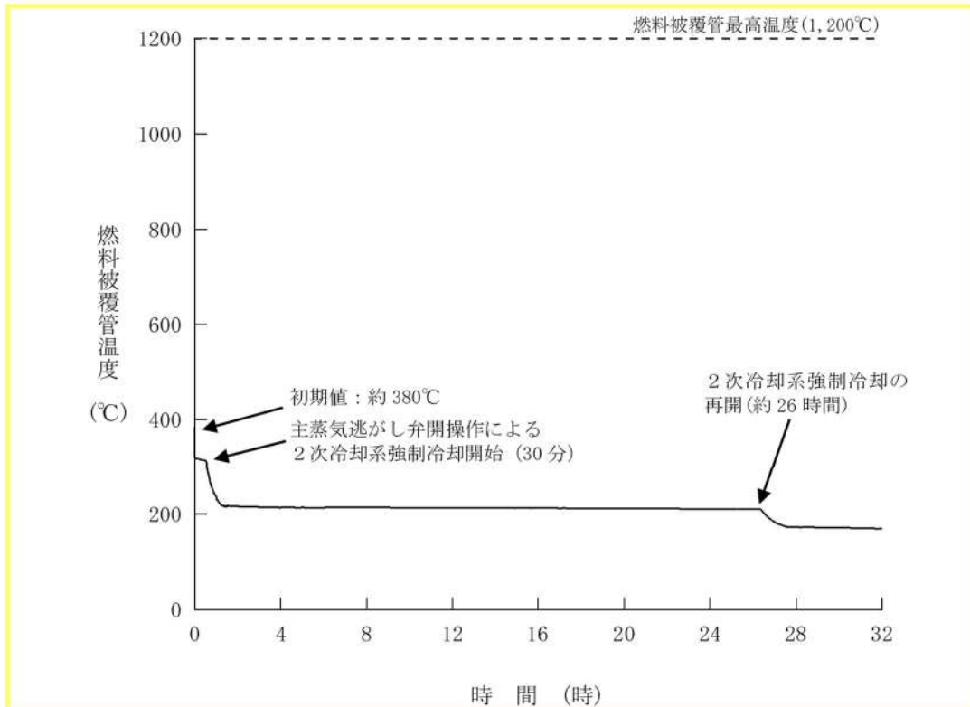
第 7. 1. 2. 35 図 燃料被覆管温度の推移 (RCP シール LOCA が発生しない場合)
