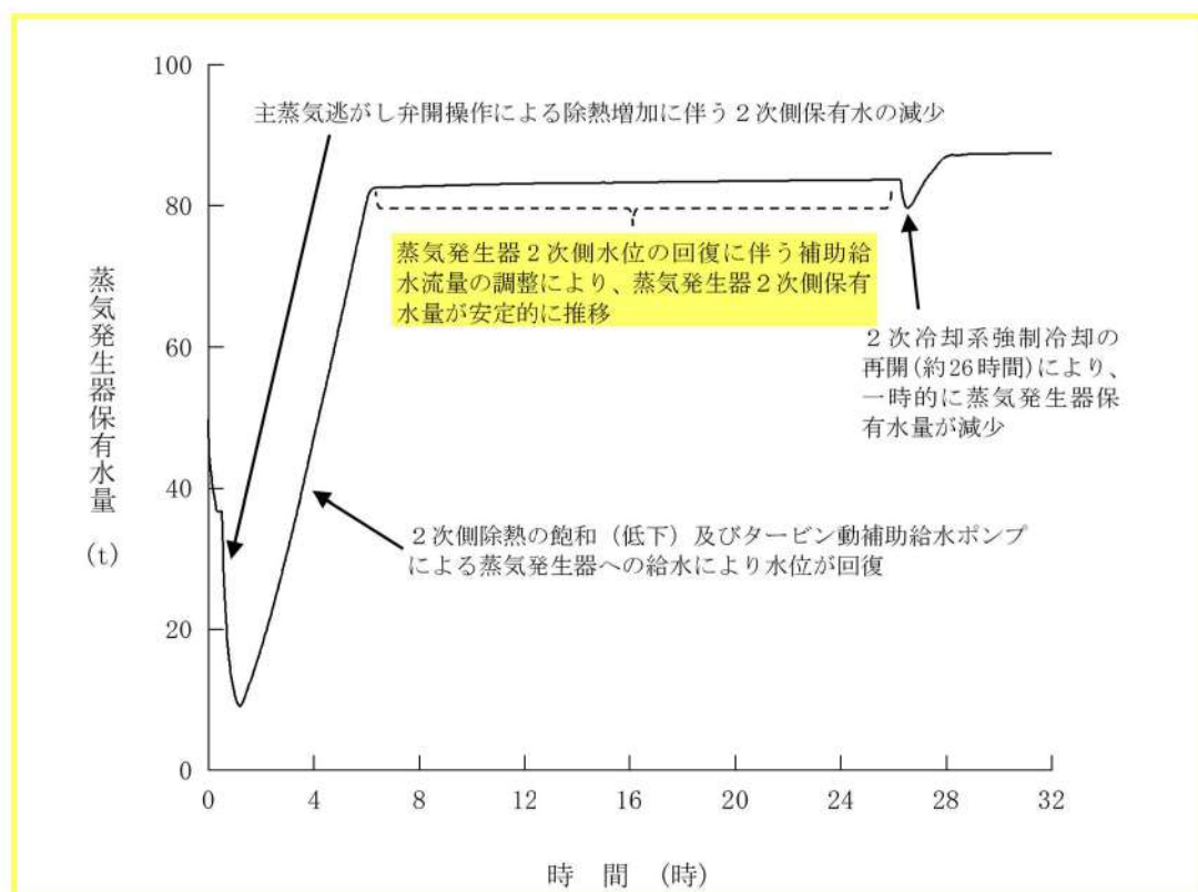
第 7. 1. 2. 38 図 蒸気発生器保有水量の推移 (RCP シール LOCA が発生しない場合)
