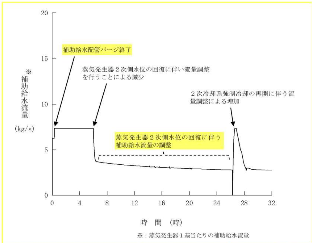
第 7.1.2.40 図 補助給水流量の推移 (RCP シール LOCA が発生しない場合)
