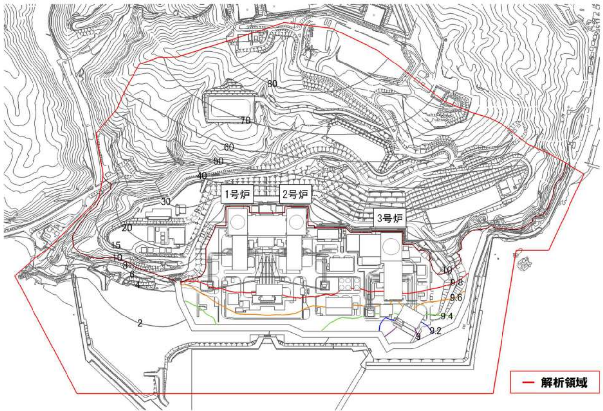
第 3.1-3 図 三次元浸透流解析結果(定常状態・防潮堤設置後モデル(例))
