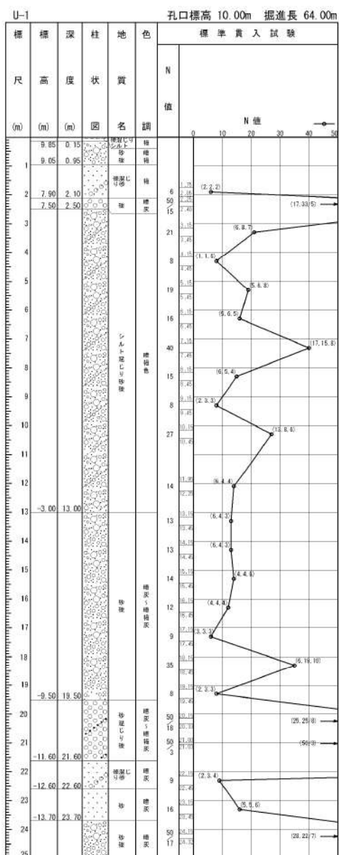
参考 1-41 図(1/3) ボーリング柱状図・コア写真 (U-1)
