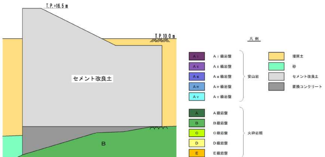
第 3.2-13 図 防潮堤断面図
