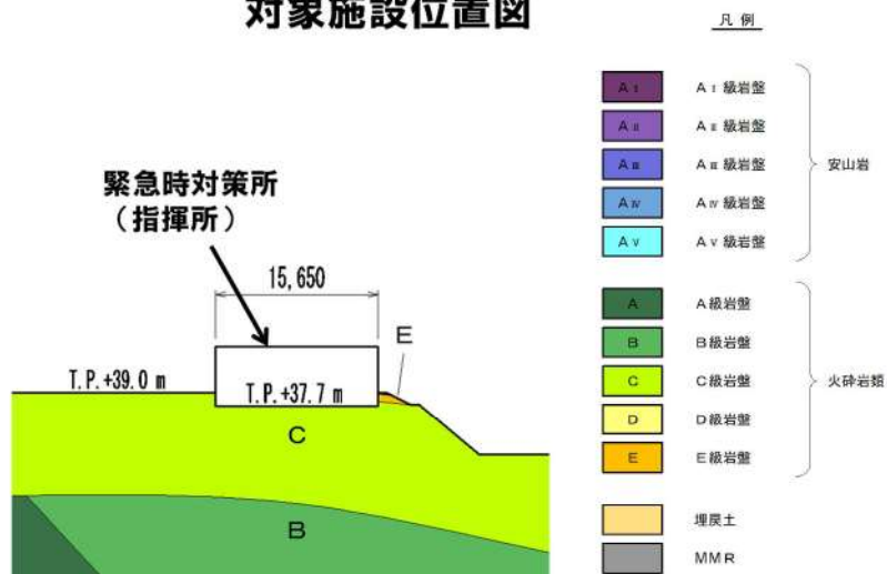
④緊急時対策所(指揮所)断面図(南北)
