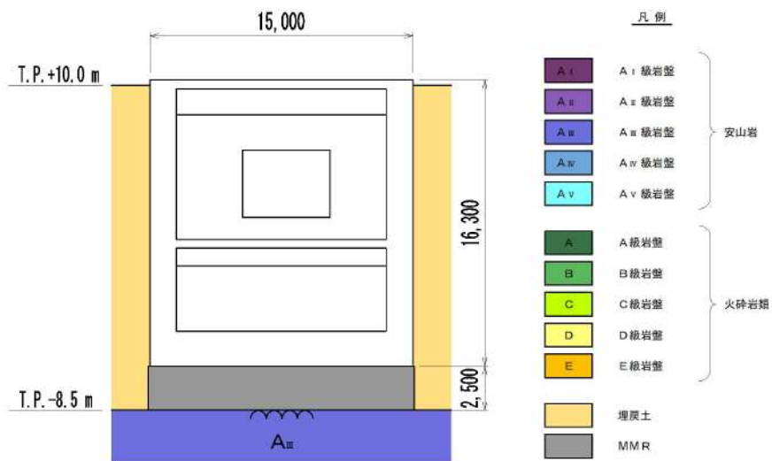
第 3.2-8 図 原子炉補機冷却海水ポンプ出口ストレーナ室断面図
