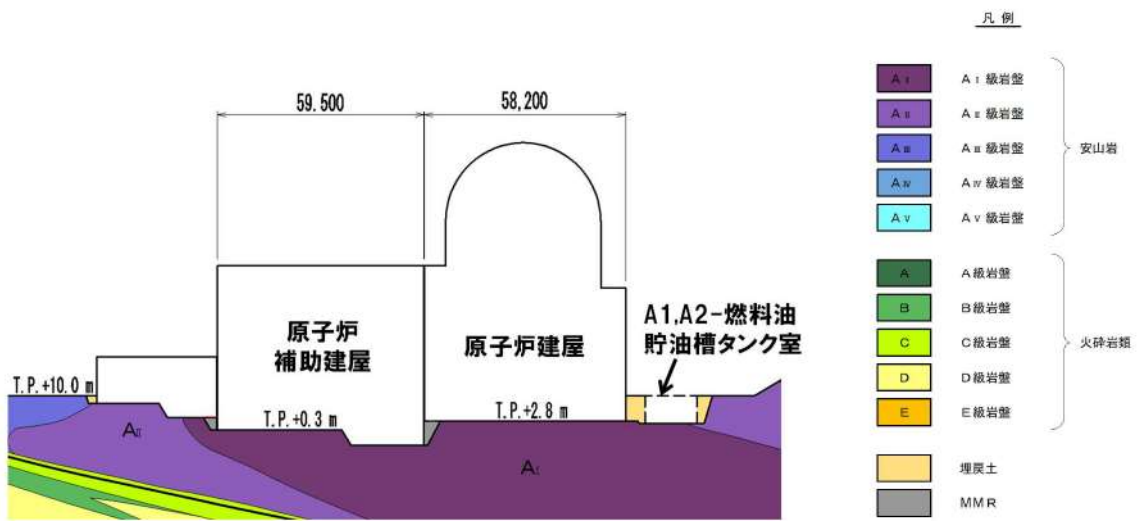
第 3.2-1 図 原子炉建屋，原子炉補助建屋，A1, A2-燃料油貯油槽タンク室断面図(東西)
