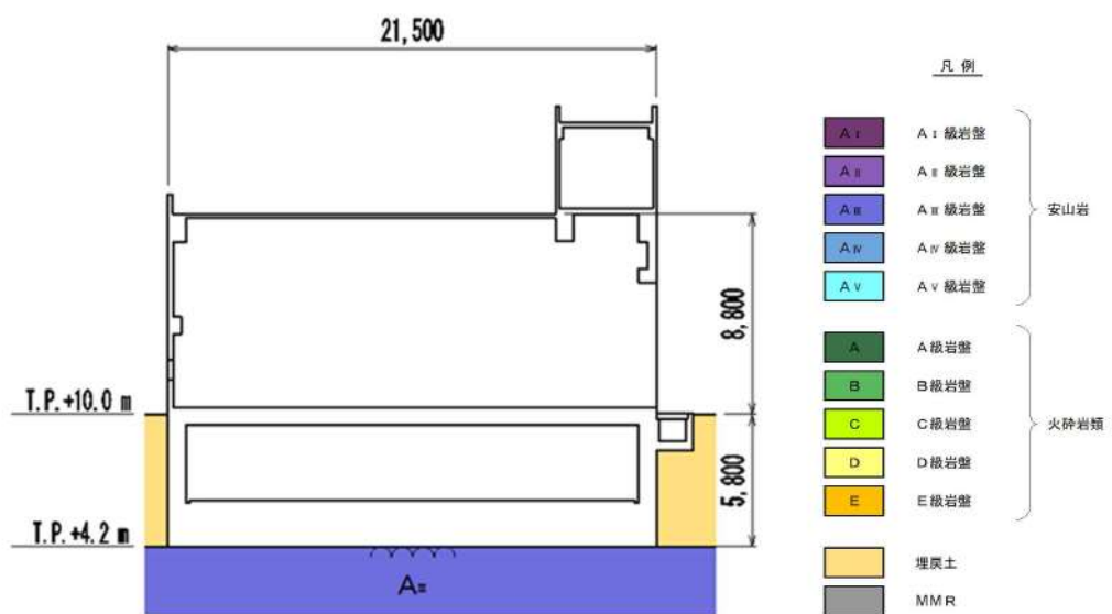
第 3.2-3 図 ディーゼル発電機建屋断面図
