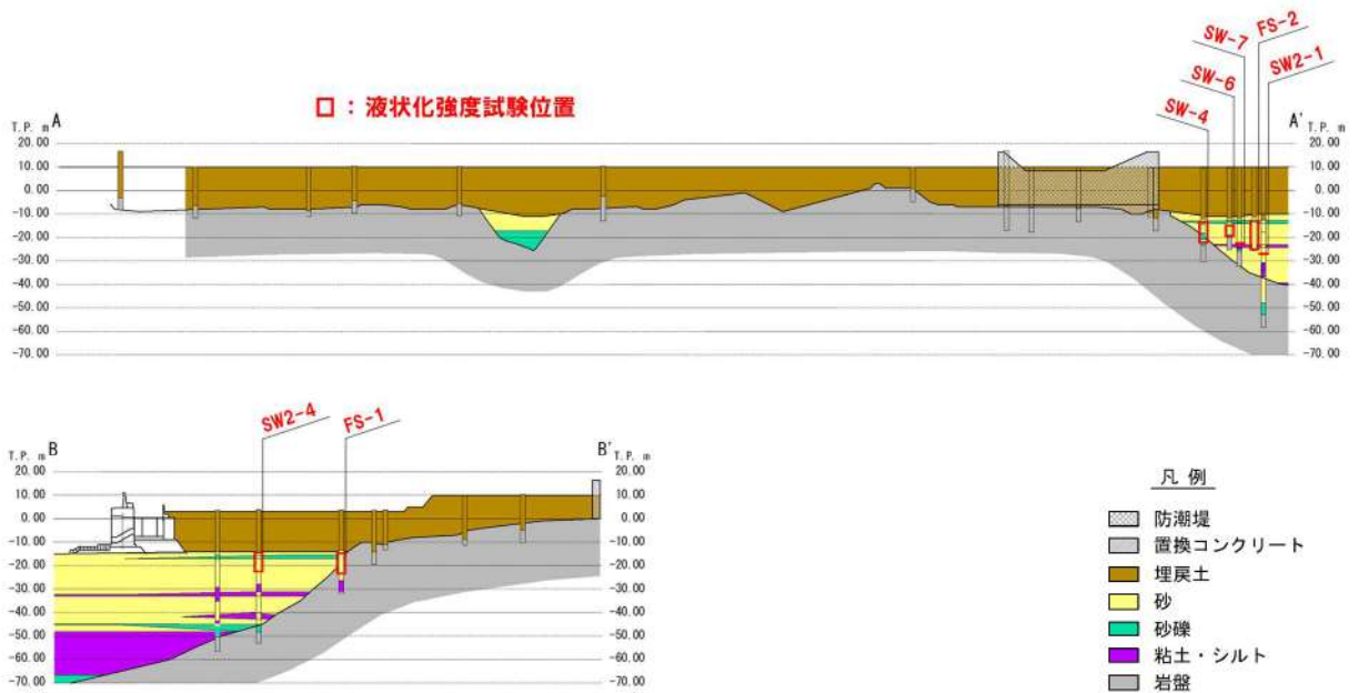
第 4.1-5 図 液状化強度試験に用いる試料採取位置断面図(砂層)
