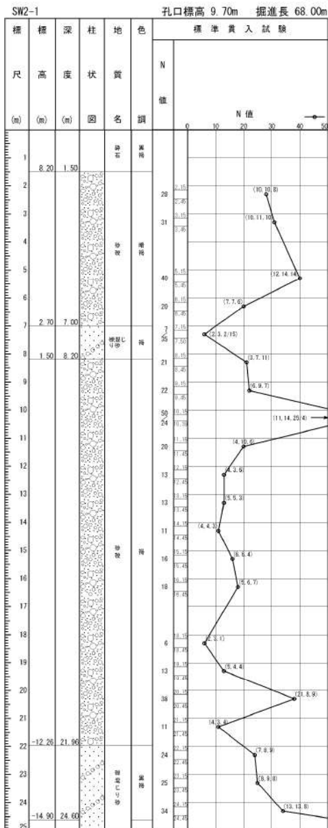
参考 1-45 図(1/3) ボーリング柱状図・コア写真 (SW2-1)
