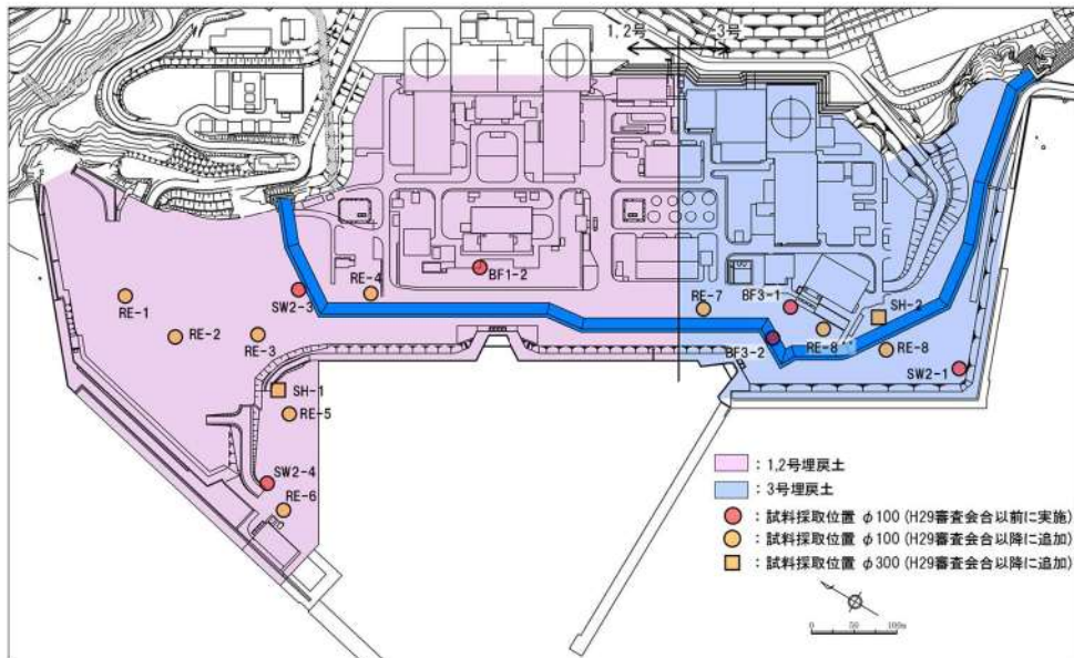
第 5.3-1 図 液状化強度試験箇所平面図(埋戻土)
