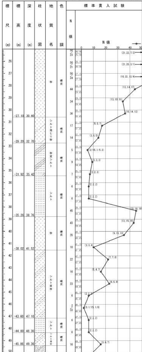
参考 1-9 図(2/3) ボーリング柱状図・コア写真 (RE-6)
