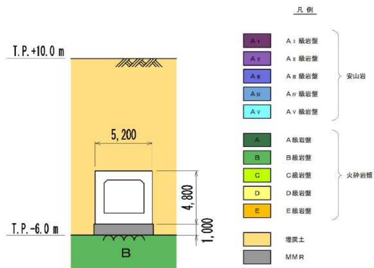
第 3.2-7 図 原子炉補機冷却海水管ダクト断面図
