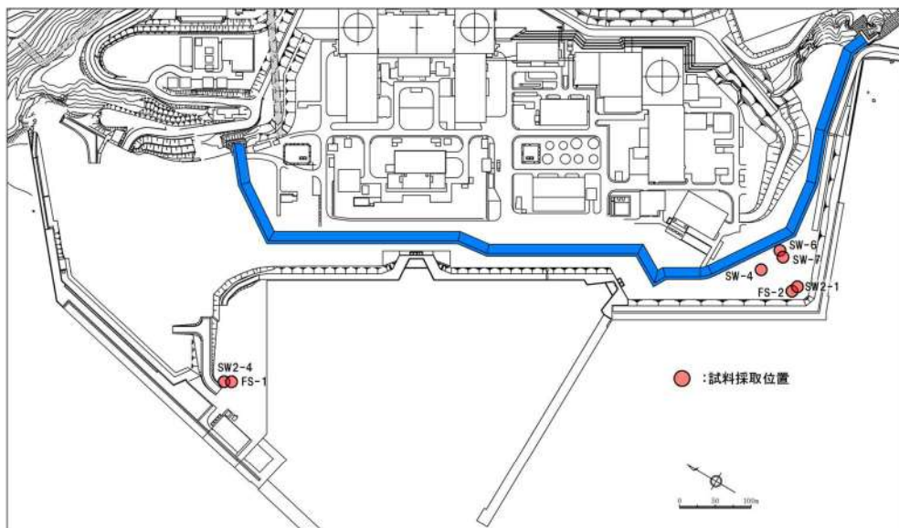
第 5.3-2 図 液状化強度試験箇所平面図(砂層)
