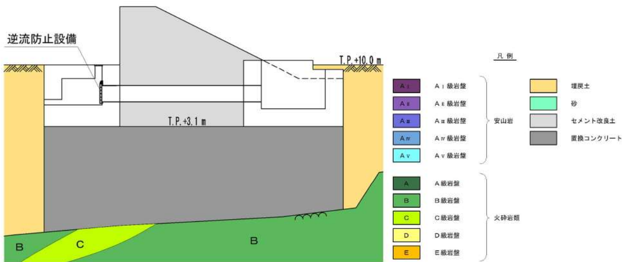
第 3.2-14 図 屋外排水路逆流防止設備断面図
