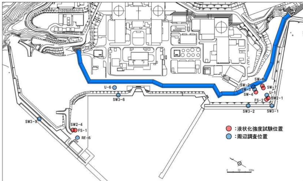
第 4.2-5 図 液状化強度試験位置並びに周辺調査位置(砂層)
