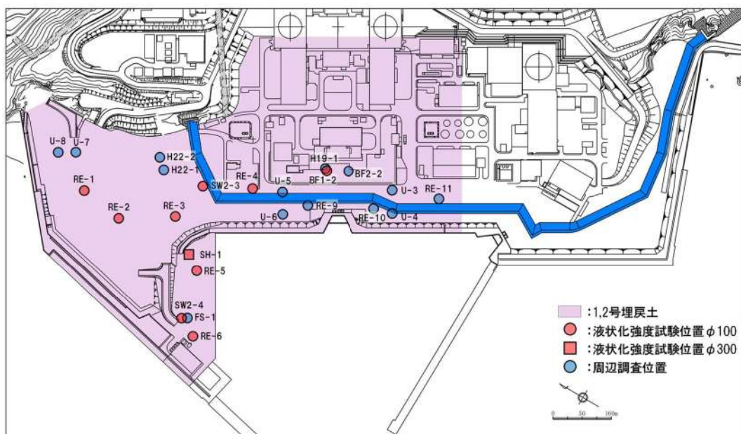
第4.2-1図 液状化強度試験位置並びに周辺調査位置(1, 2号埋戻土)
