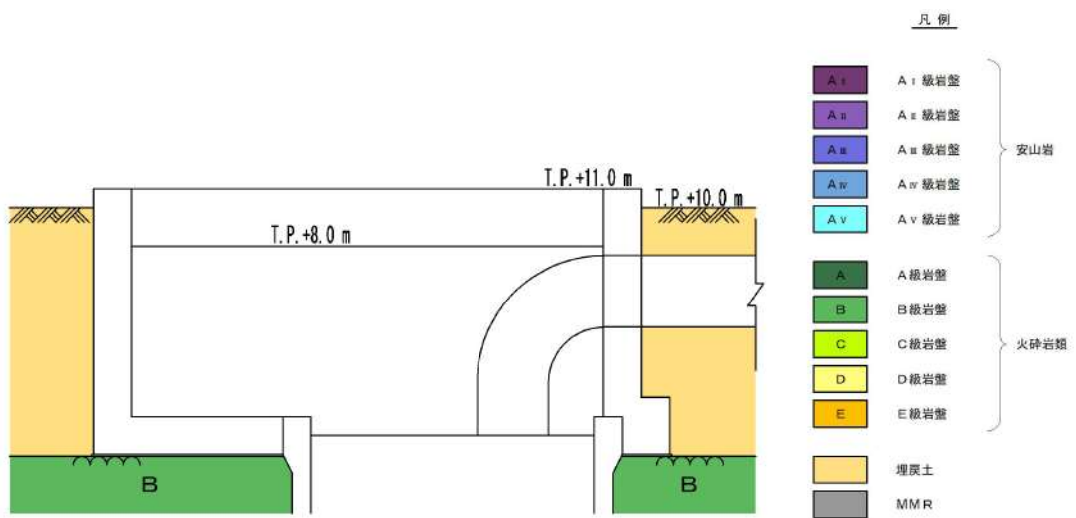
第 3.2-15 図 3 号炉放水ピット流路縮小工断面図
