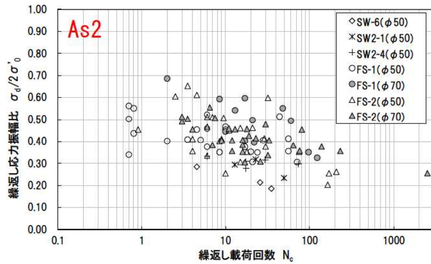
第 5.3-8 図 砂層の液状化強度試験結果
