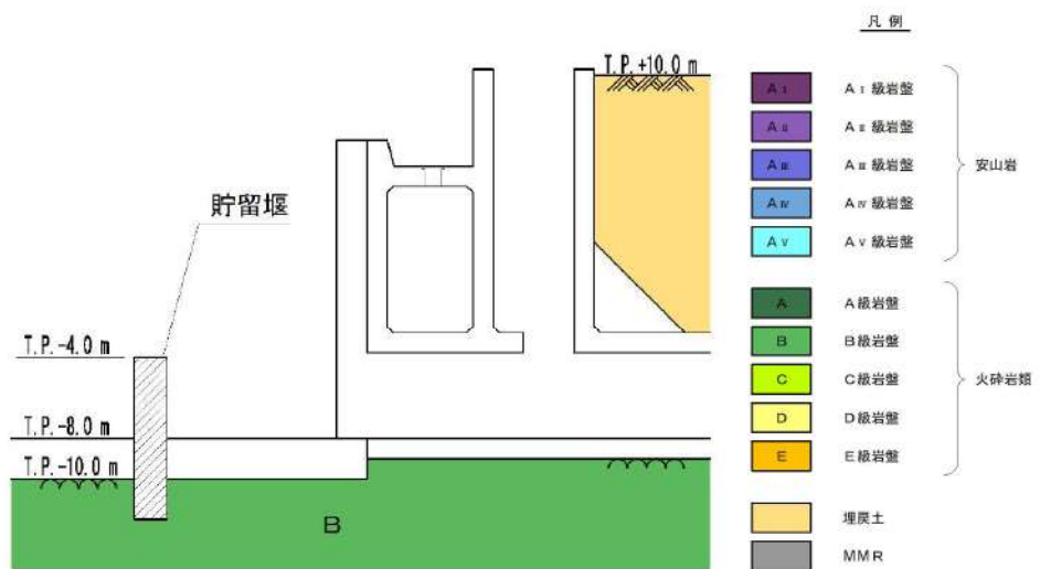
②貯留堰部断面図
