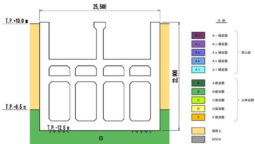
第 3.2-9 図 取水ピットポンプ室断面図
