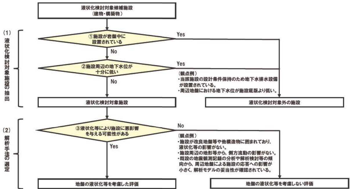
第 3.1-2 図(1) 液状化検討対象施設の選定及び解析手法選定フロー(建物・構築物)
