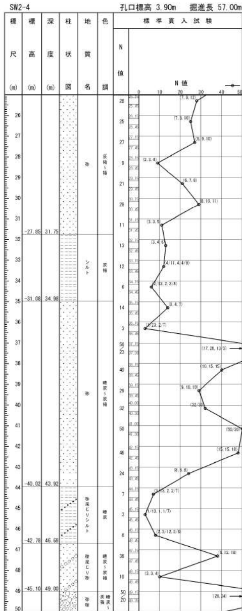
参考 1-2 図(2/3) ボーリング柱状図・コア写真 (SW2-4)
