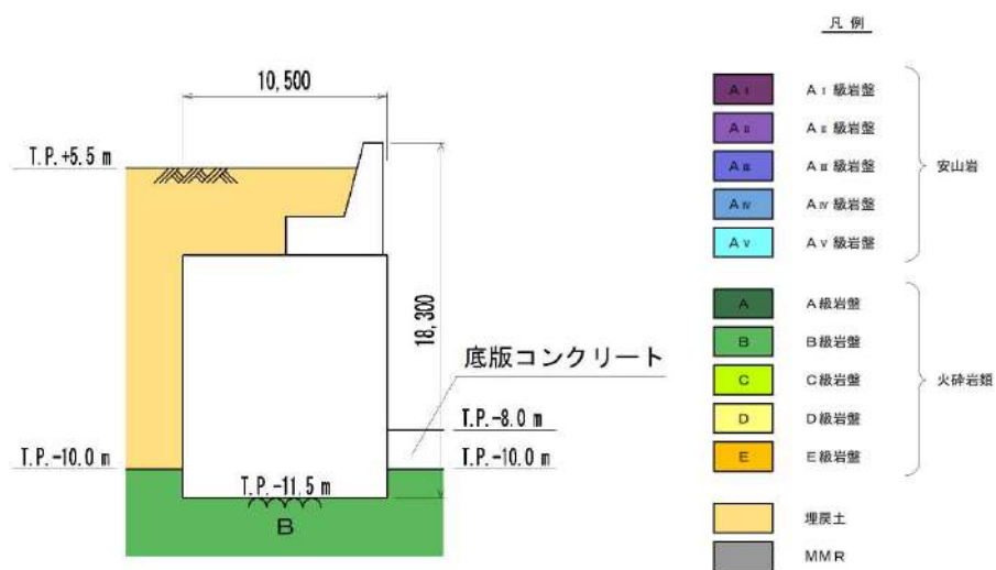
①護岸部断面図
