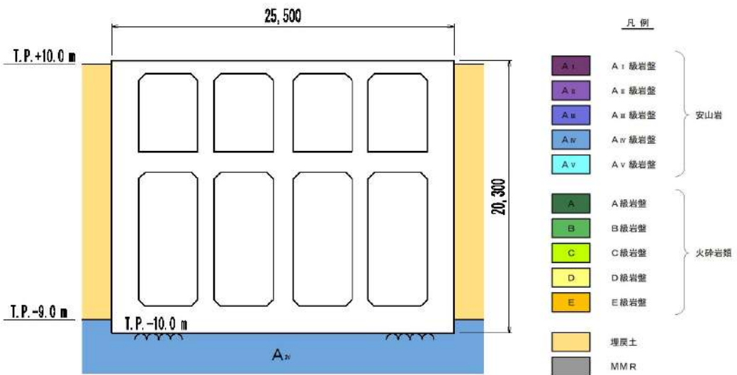
第 3.2-10 図 取水ピットスクリーン室断面図
