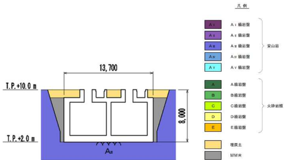
第 3.2-5 図 B1, B2-燃料油貯油槽タンク室断面図
