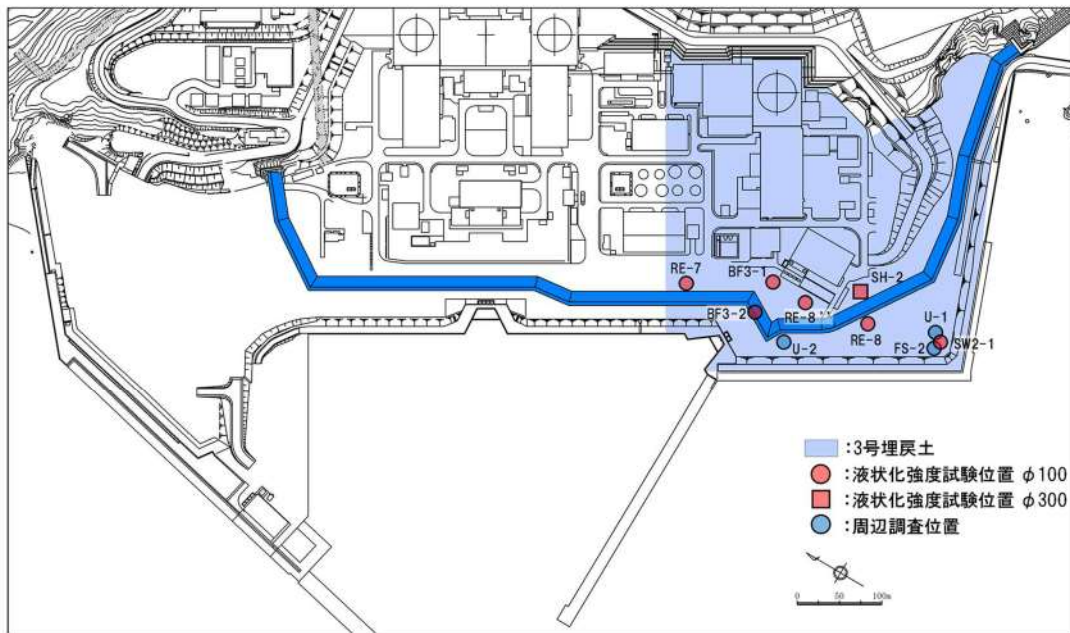
第4.2-3図 液状化強度試験位置並びに周辺調査位置(3号埋戻土)
