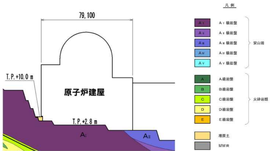
第 3.2-2 図 原子炉建屋断面図(南北)
