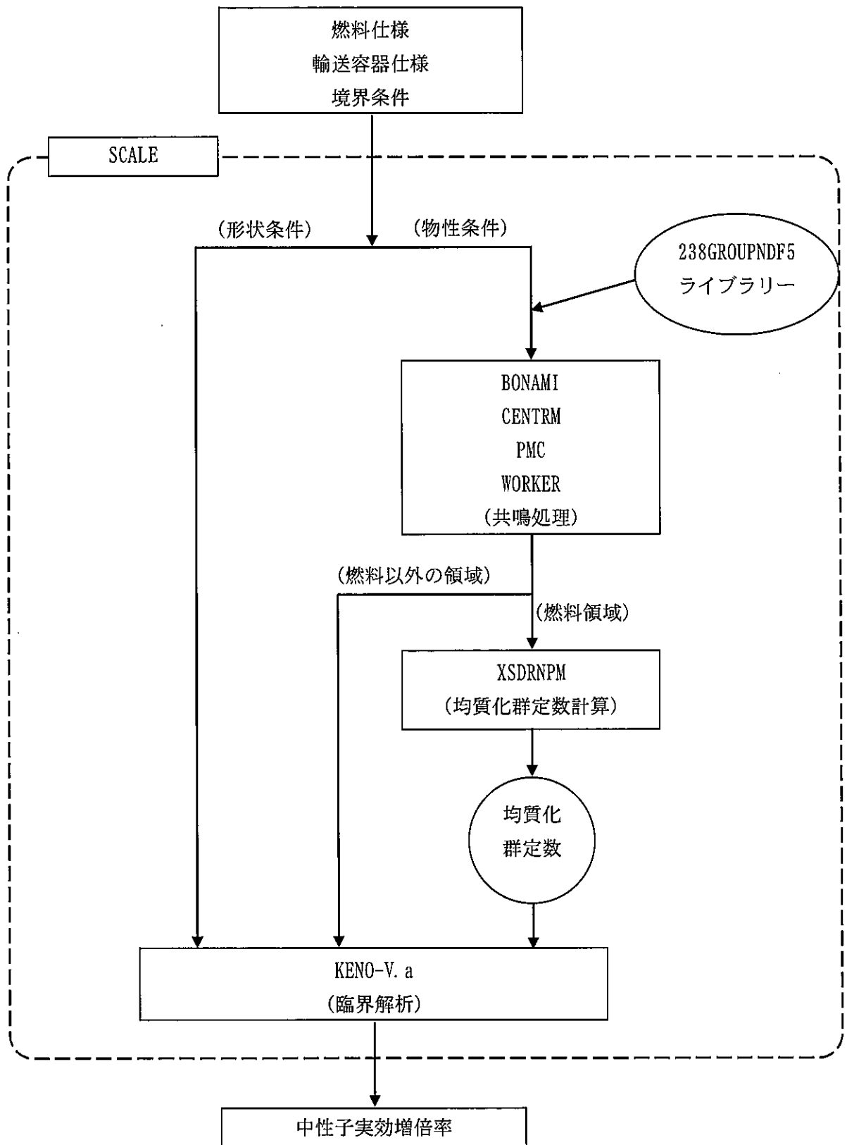
(口) - 第E. 4 図 臨界計算の流れ
