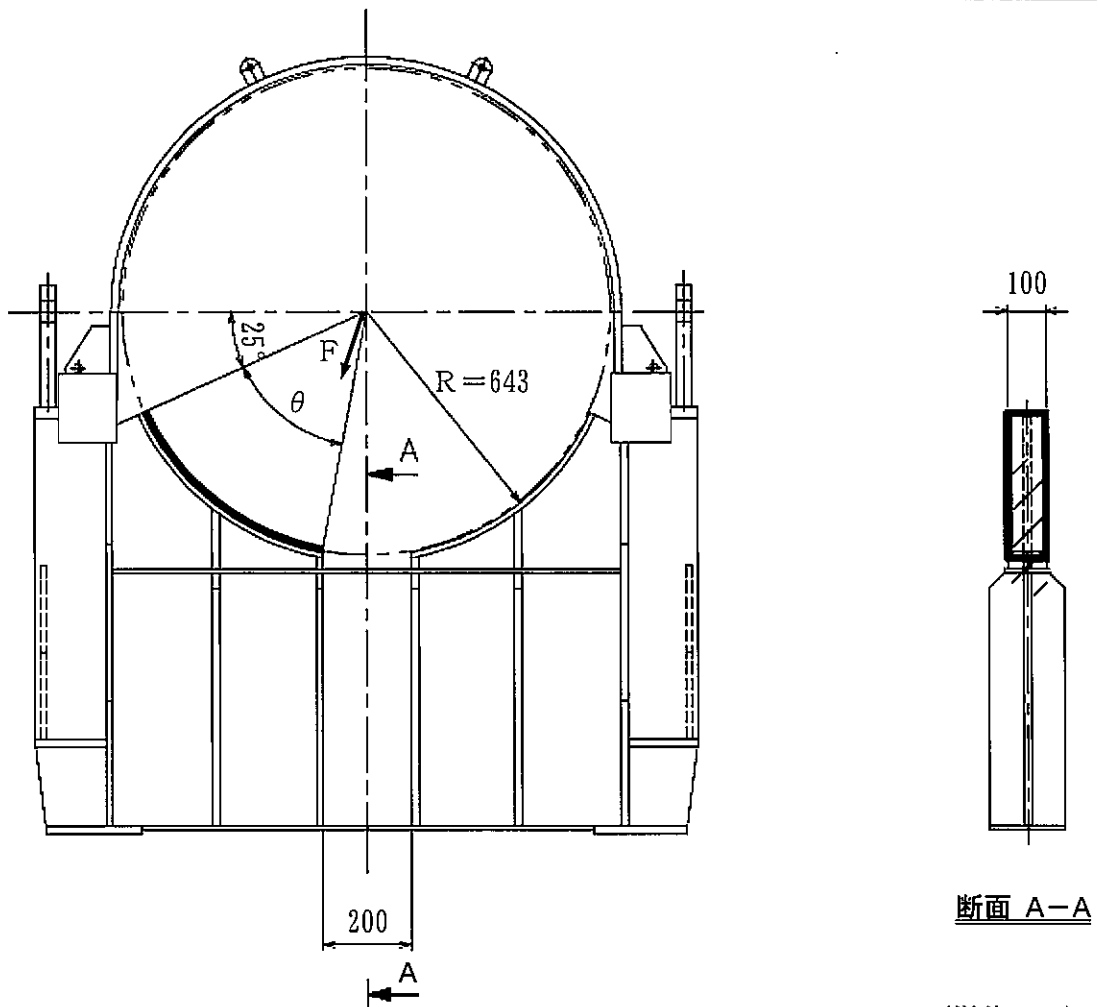
(口) - 第A. 6 図 外筒支圧面積範囲
