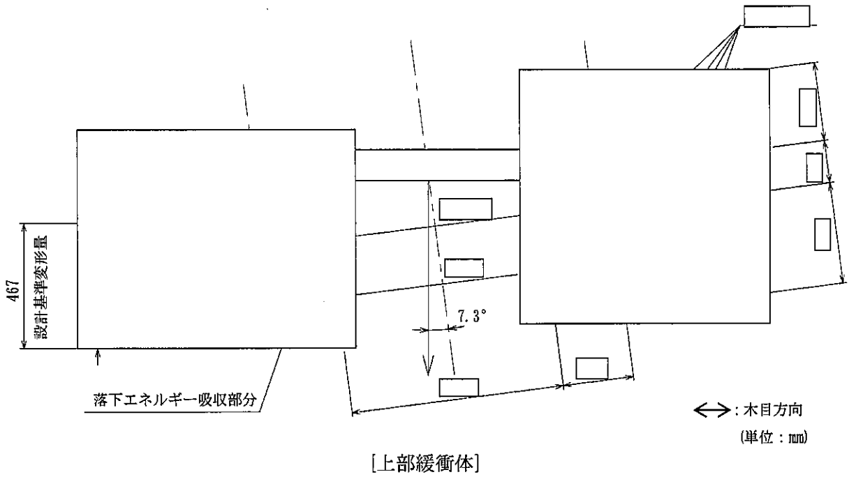
(口) - 第A. 16 図 頭部コーナー落下解析モデル
