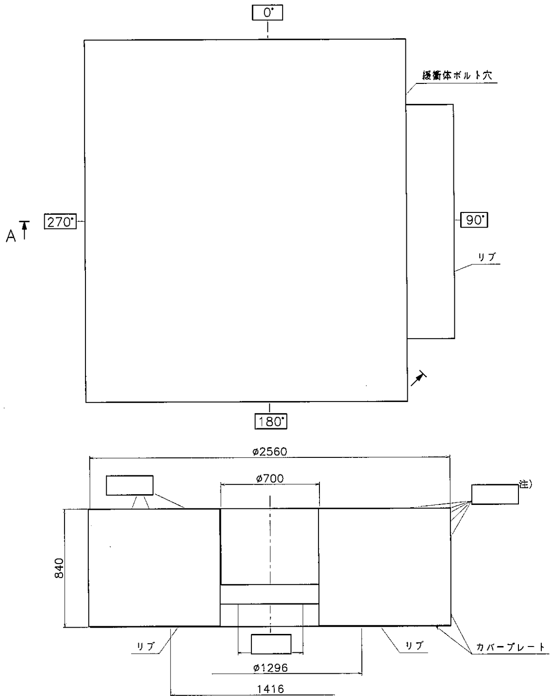
断面 A-A
