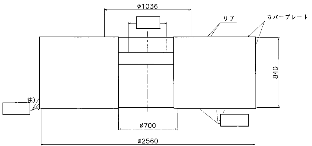
断面 A-A
