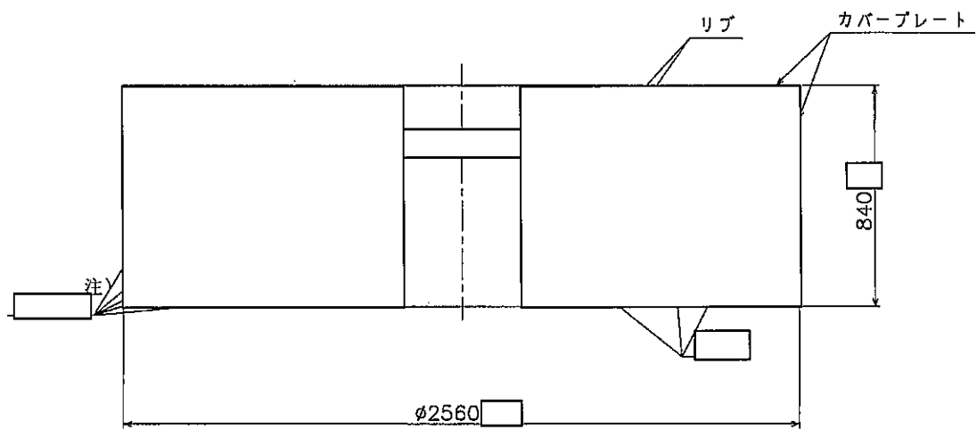
断面 A-A
