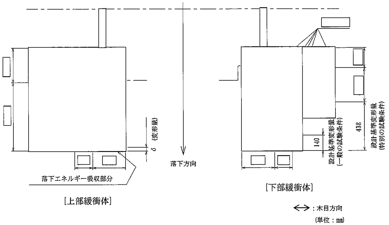
(口) - 第A. 15 図 水平落下解析モデル
