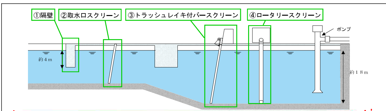
【取水設備の構成（断面図）】
