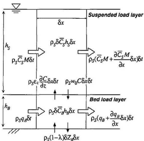
図-1 掃流砂層・浮遊砂層分離モデルの概念図
