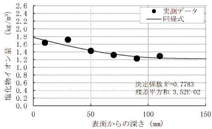
図1(2/9) 取水構造物気中帯 (SP-ci-2u-8-J-②) の回帰分析結果 (上：中性化考慮あり [○データを棄却]、下：中性化考慮なし)
