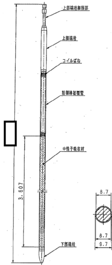
図11-2 17×17型制御棒構造図
