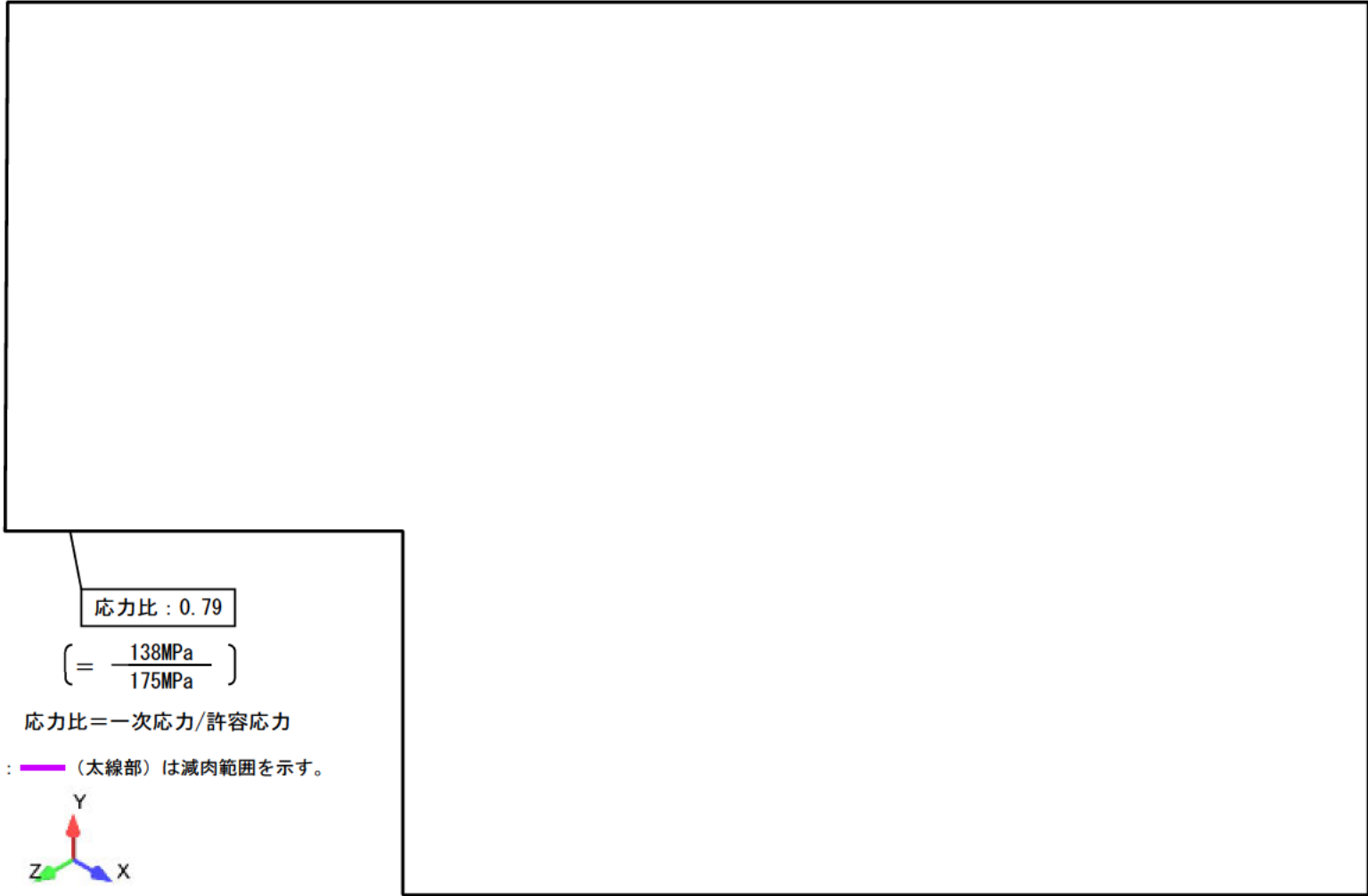
タービングランド蒸気系統配管 グランド蒸気管
