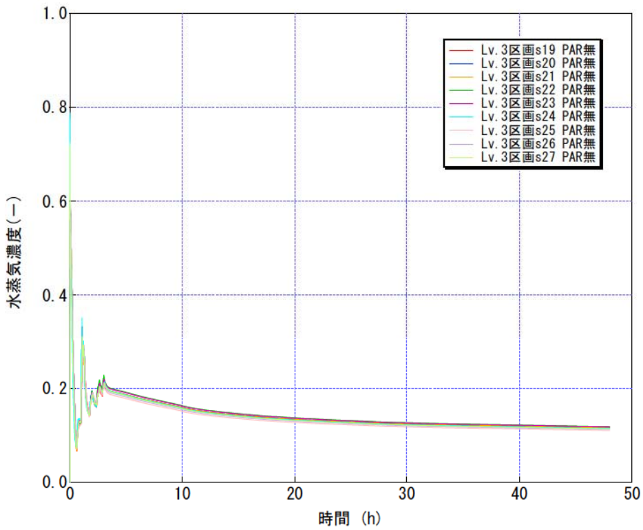
図8 上部区画Lv. 3水蒸気濃度
