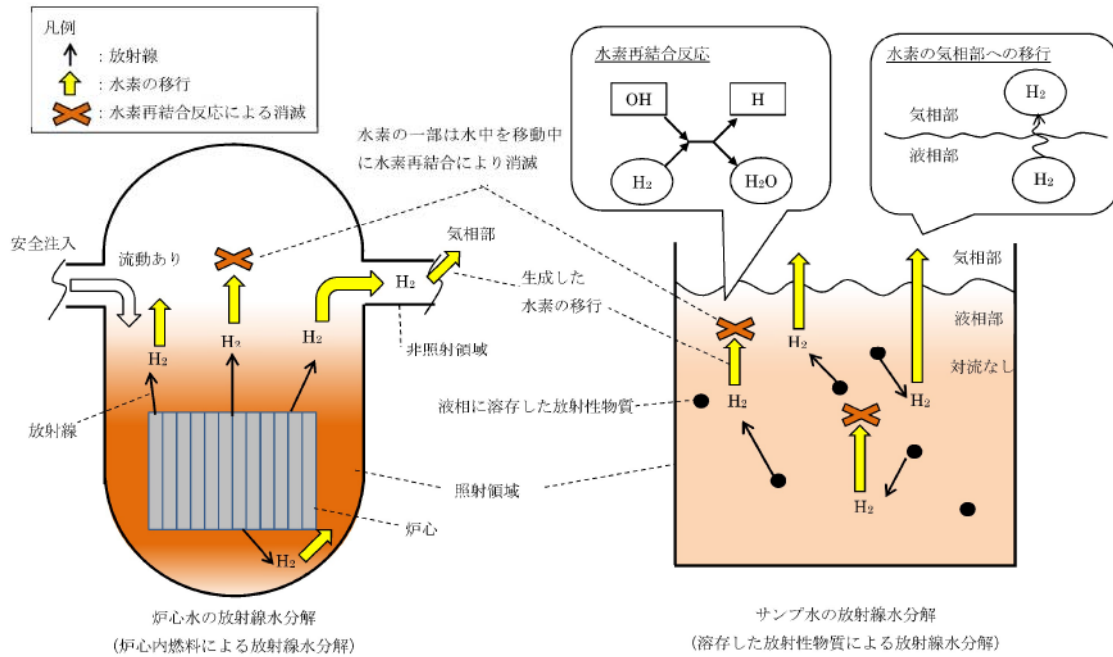
図 11 炉心水及びサンプル水における水の放射線分解による水素発生(イメージ)
