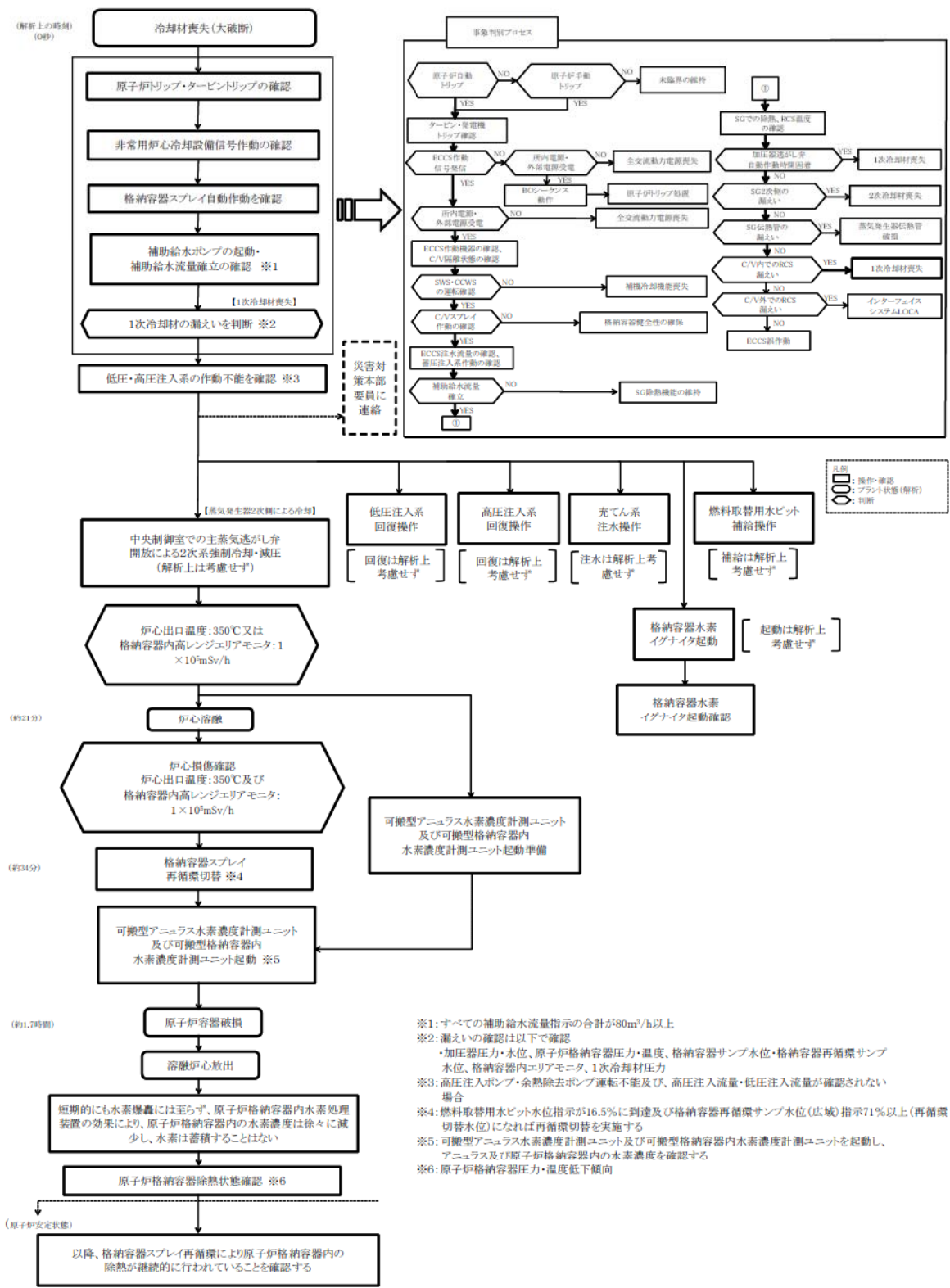
第 7.2.4.6 図 「水素燃焼」の事象進展 (対応手順の概要) (大破断 LOCA 時に低压注入機能及び高压注入機能が喪失する事故)
