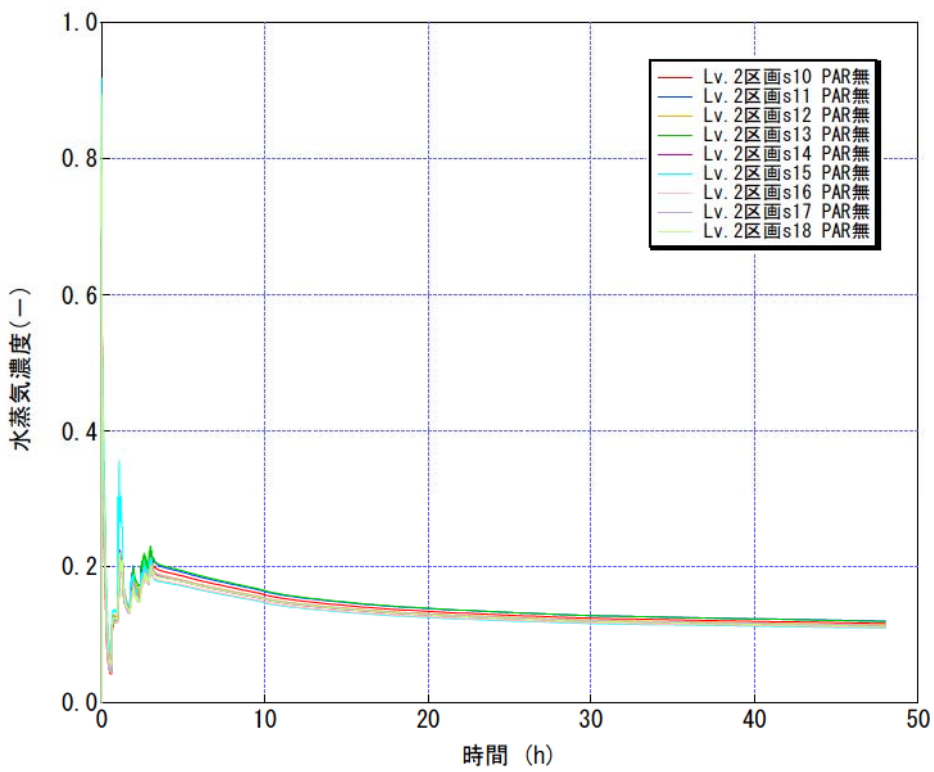
図6 上部区画Lv. 2水蒸気濃度
