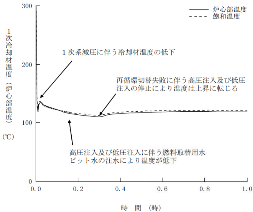
図2 1次冷却材温度の推移 (本資料 第7.1.7.5図の拡大図)
