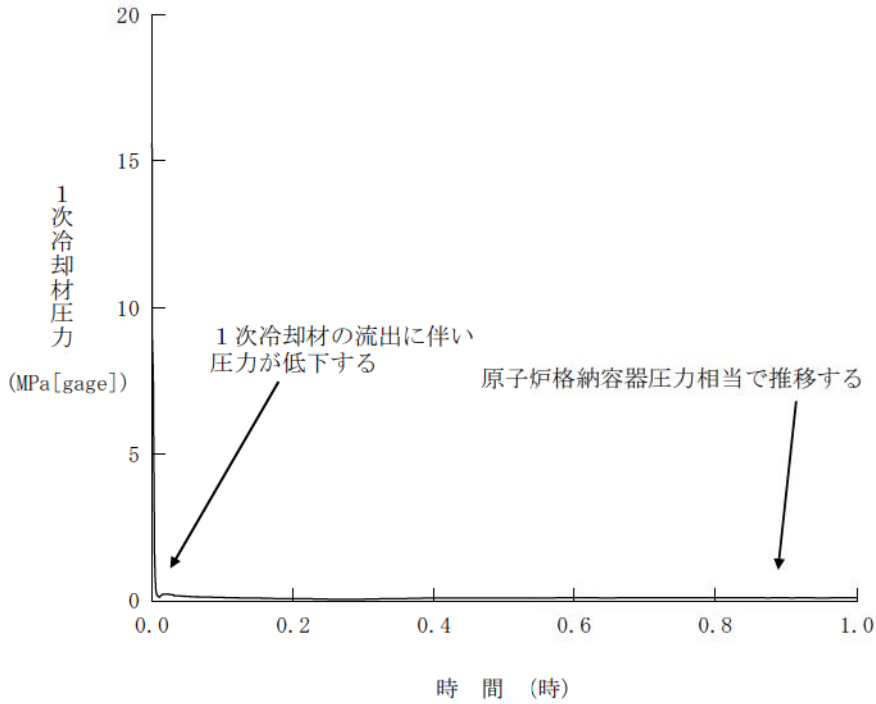
図1 1次冷却材圧力の推移 (本資料 第7.1.7.4図の拡大図)
