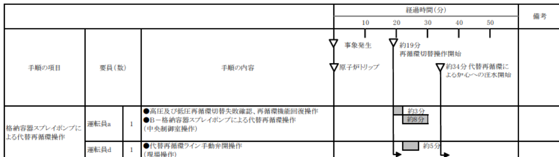
図-1 代替再循環運転タイムチャート
