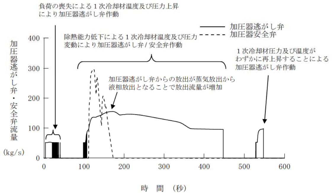
第 7. 1. 5. 21 図 加圧器逃がし弁・安全弁流量の推移（負荷の喪失）
