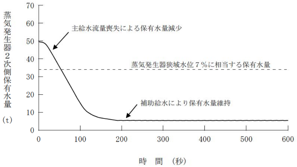
第 7. 1. 5. 28 図 蒸気発生器2次側保有水量の推移（負荷の喪失）
