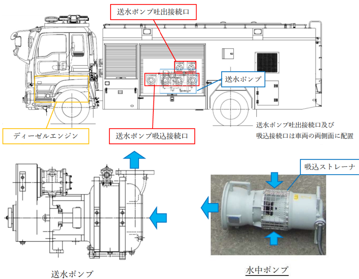
図 48-10-1 可搬型大型送水ポンプ車の構造概要図
