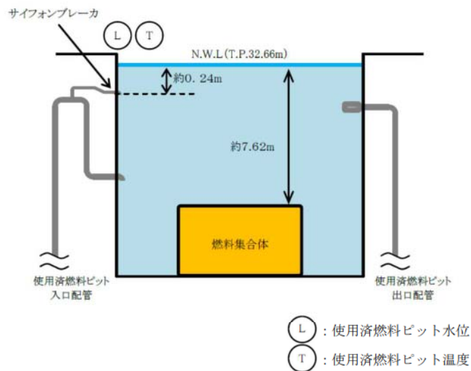
第 4. 1. 5 図 サイフォンブレーカの配置の概要図
