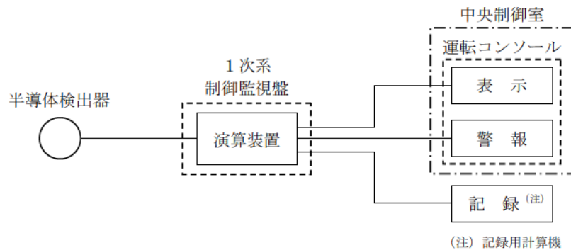
図 1.2.6 使用済燃料ピットエリアモニタのシステム構成ブロック図
