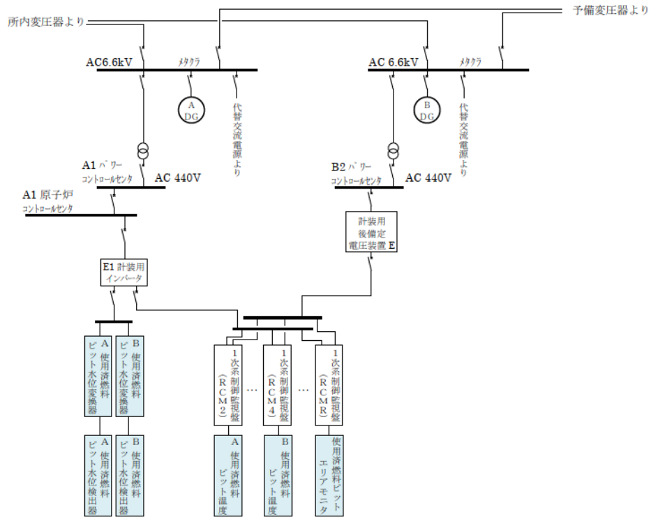
図 1.4.1 使用済燃料ピット監視設備（設計基準対象設備）の電源構成
