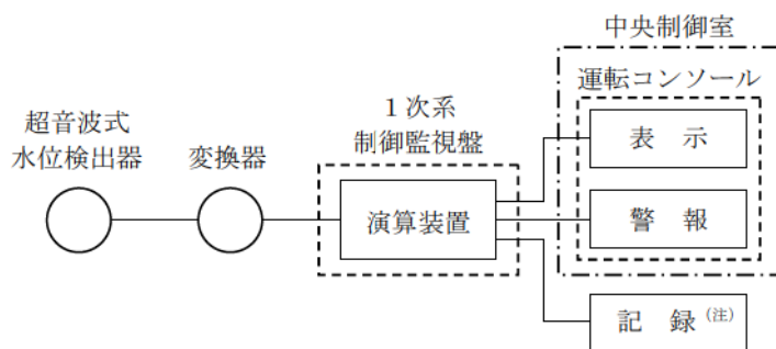
図 1.2.2 使用済燃料ピット水位計のシステム構成ブロック図
