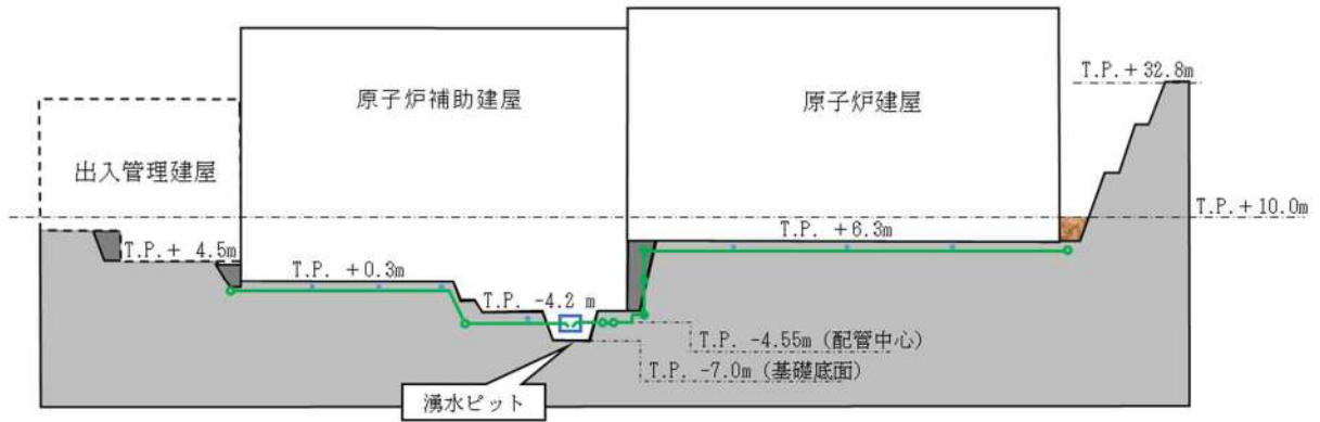
添付 1-4(1)図 集水管及びサブドレンの配置と建屋基礎底面のレベル (添付 1-3 図の A-A)
