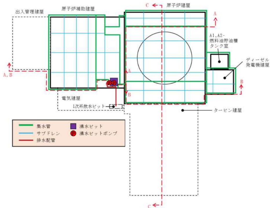
添付 1-3 図 地下水排水設備の配置
