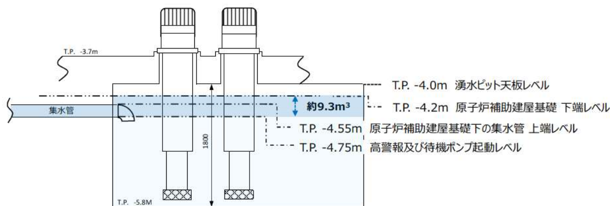
添付 3-1 図 湧水ピットと集水管による貯留可能量
