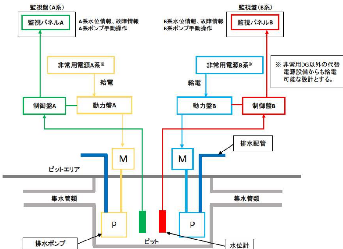
別紙 11-3 図 設計上の配慮事項を反映した電源系，監視・制御系の系統構成概要
