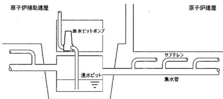
別紙 11-1 図 地下水排水設備(既設)の概念図
