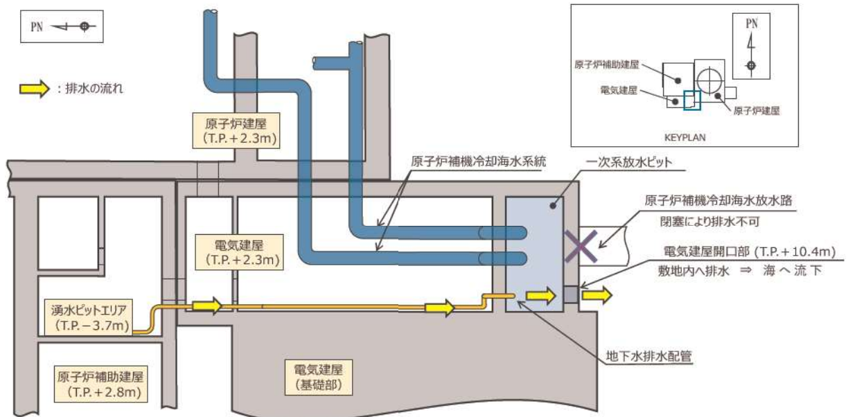
添付 4-3 図 建屋内の排水経路（地震時）
