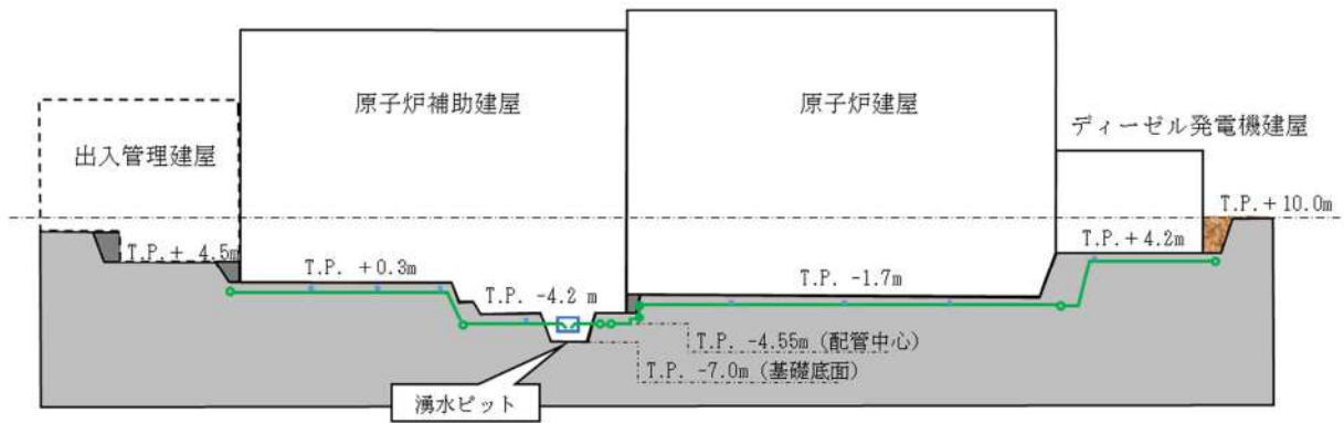
添付 1-4(2)図 集水管及びサブドレンの配置と建屋基礎底面のレベル (添付 1-3 図の B-B)
