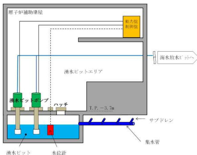
添付 1-1 図 設備構成イメージ
