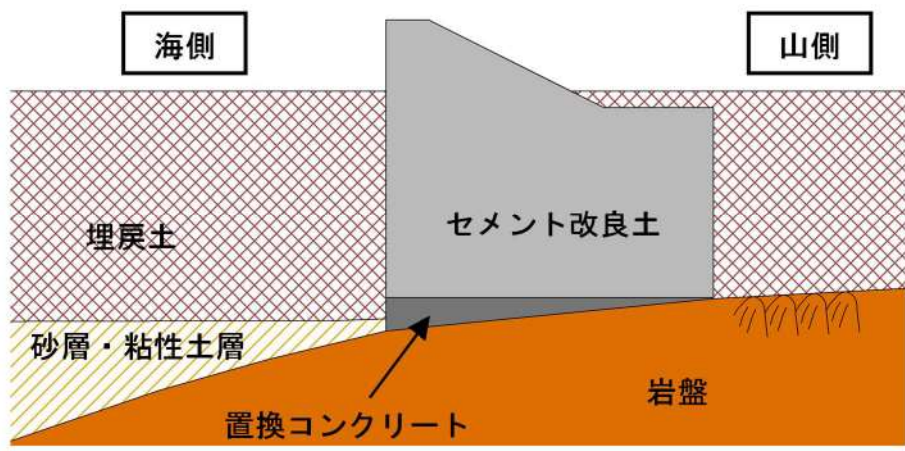
別紙 11-2 図 岩着構造の防潮堤概要図
