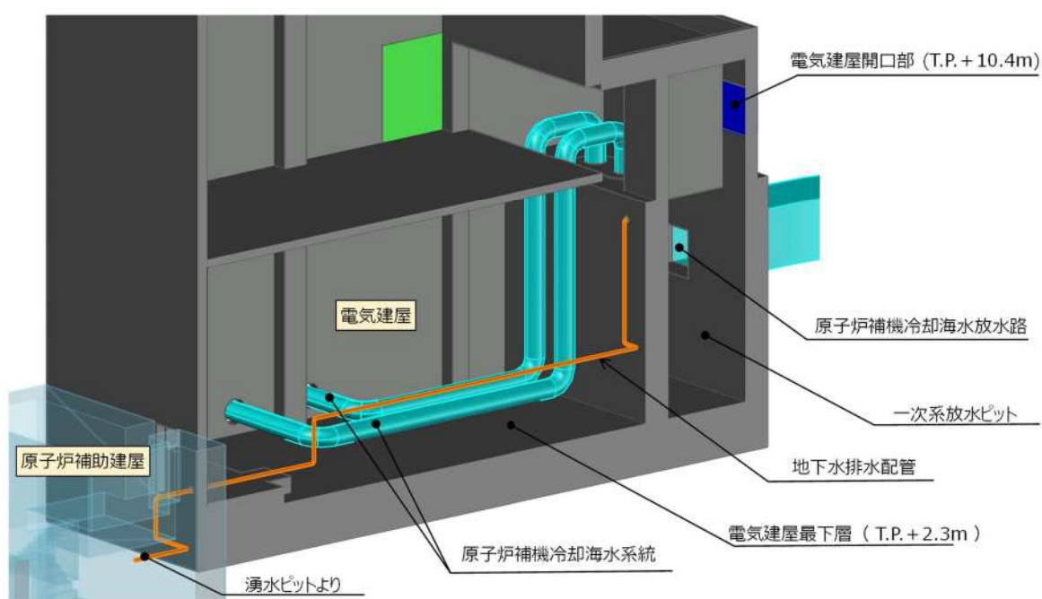
添付 4-1 図 電気建屋内イメージ図（現状）
