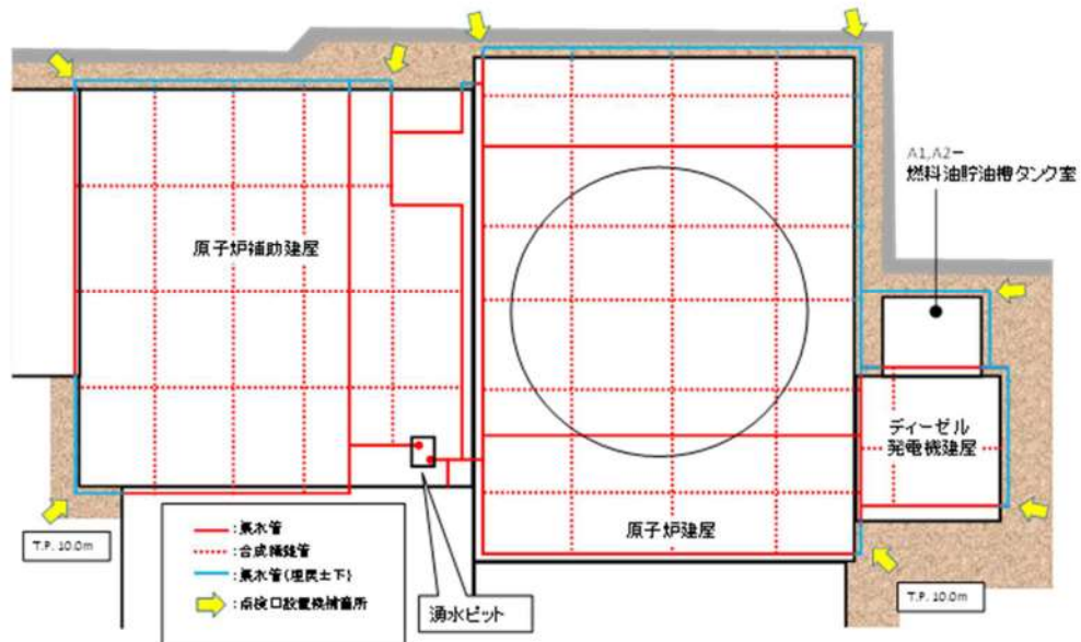
添付 6-4 図 点検口の設置候補箇所
