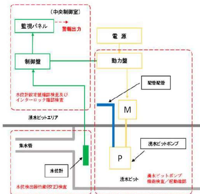
別紙 11-4 図 地下水排水設備の試験又は検査項目と範囲
