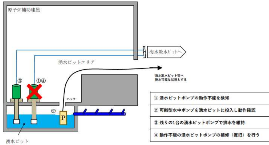
別紙 11-6 図 可搬型水中ポンプの運用例 (湧水ピットポンプが動作不能な場合)
