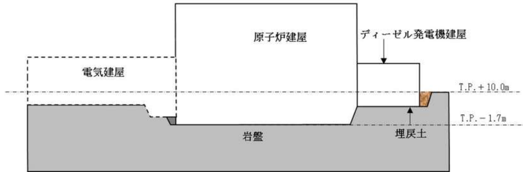
添付 2-3 図 A2-A2 断面図
