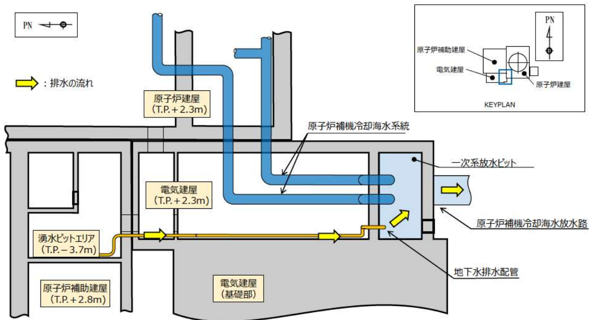
添付 4-2(1) 図 屋内の排水経路（通常時）
