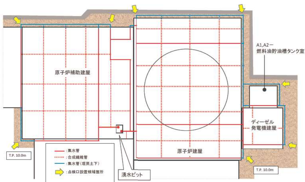
別紙 11-5 図 点検口の設置候補箇所
