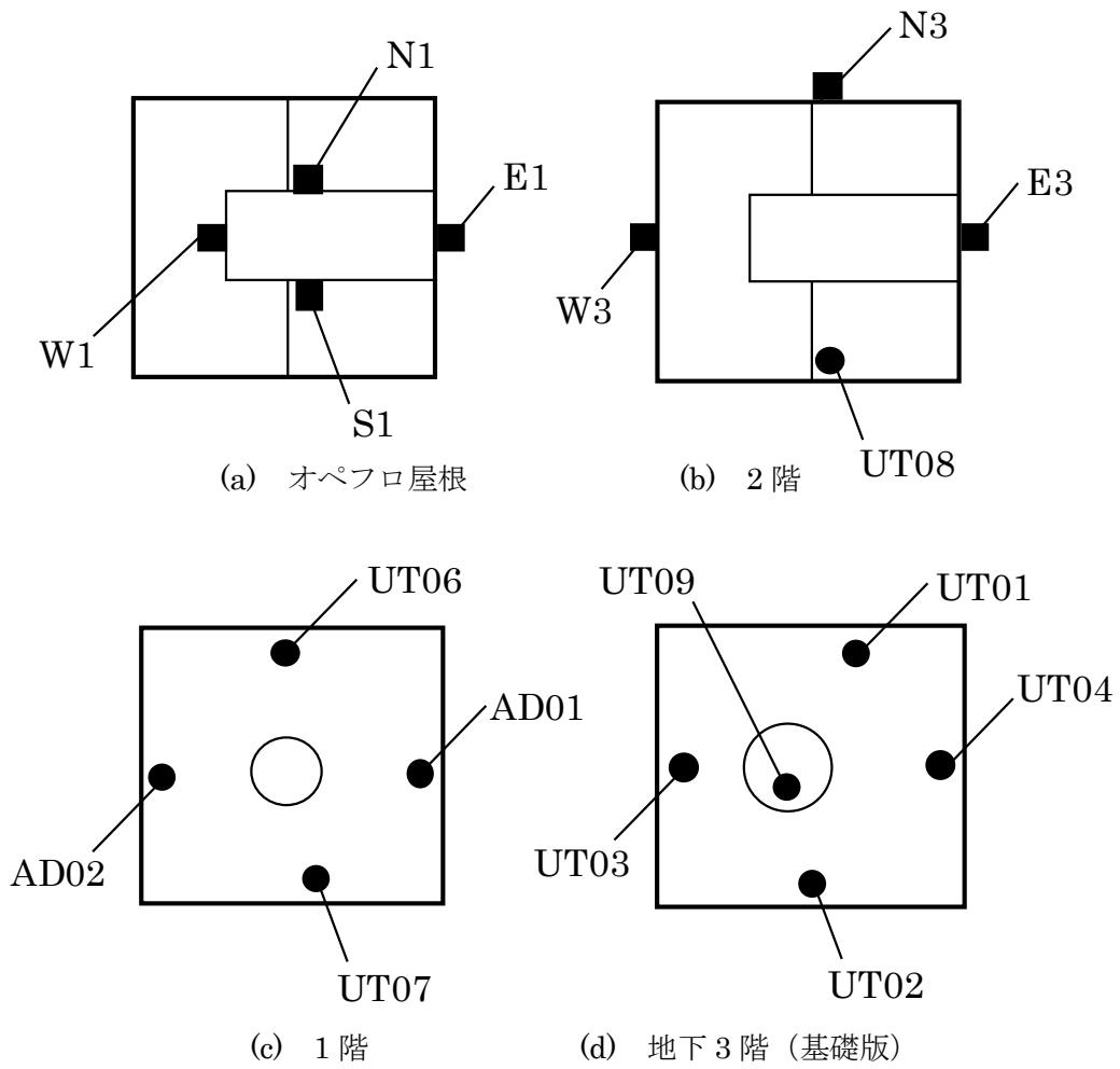
図3 対象とする各フロア加速度計位置（平面図）
