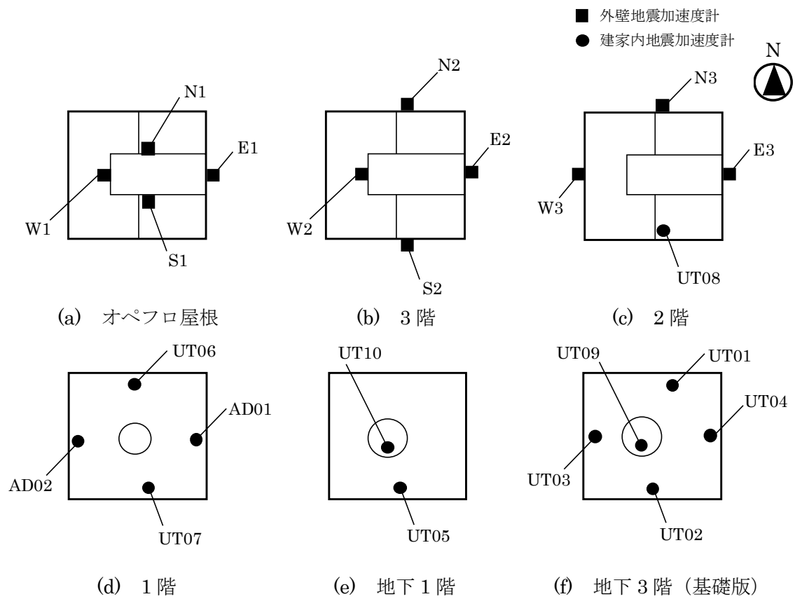
図6 建家内加速度計位置 (平面図)
