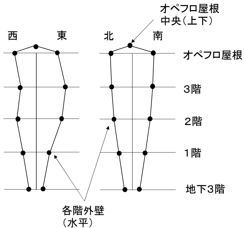
図5 外壁の水平変位・オペフロ屋根の上下変位の図化イメージ
