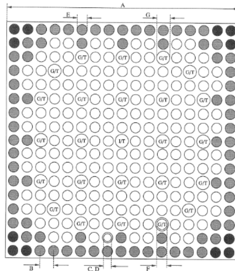
図 4. PWR17×17 型 UO_2 燃料集合体の幾何形状の仕様
