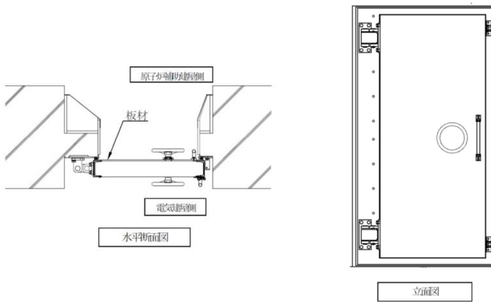
図 4.2-7 水密扉構造例 (扉 No. 68)
