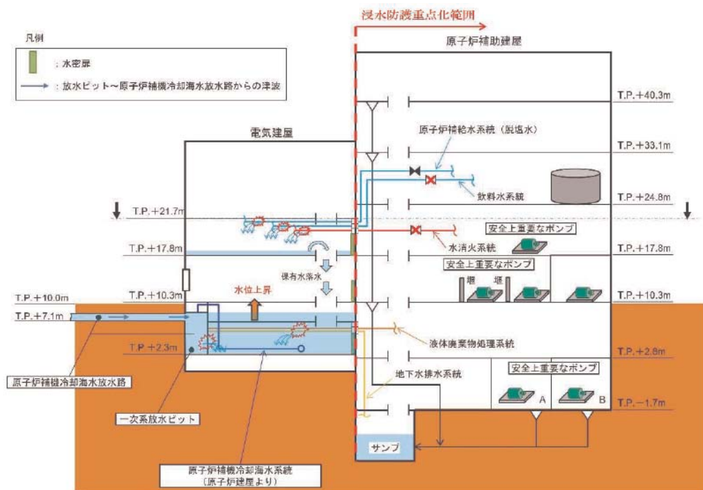
図 3.4-2(3) 地震による溢水の概念図
