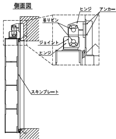
図 4.2-3 逆流防止設備構造例（断面図）
