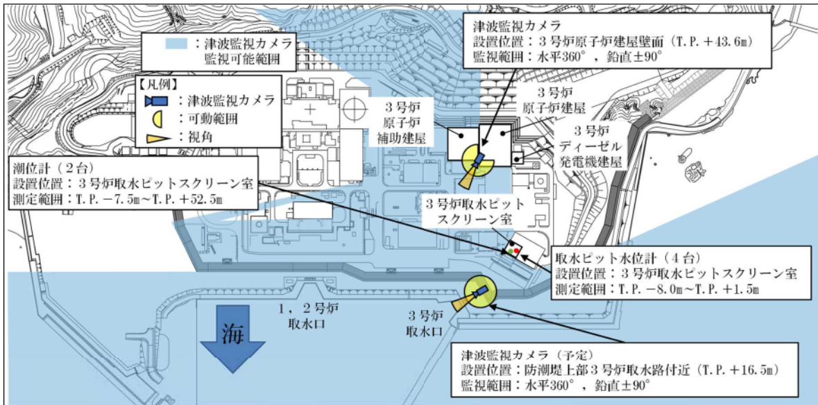
図 2.6-1 津波監視設備配置図
