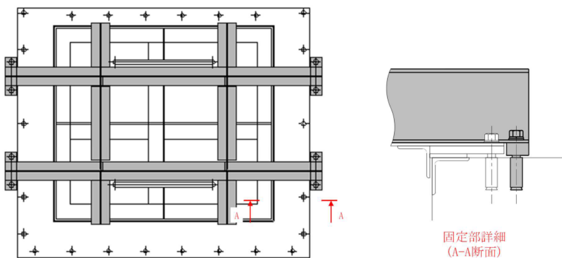
図 4.2-12 浸水防止蓋構造例
