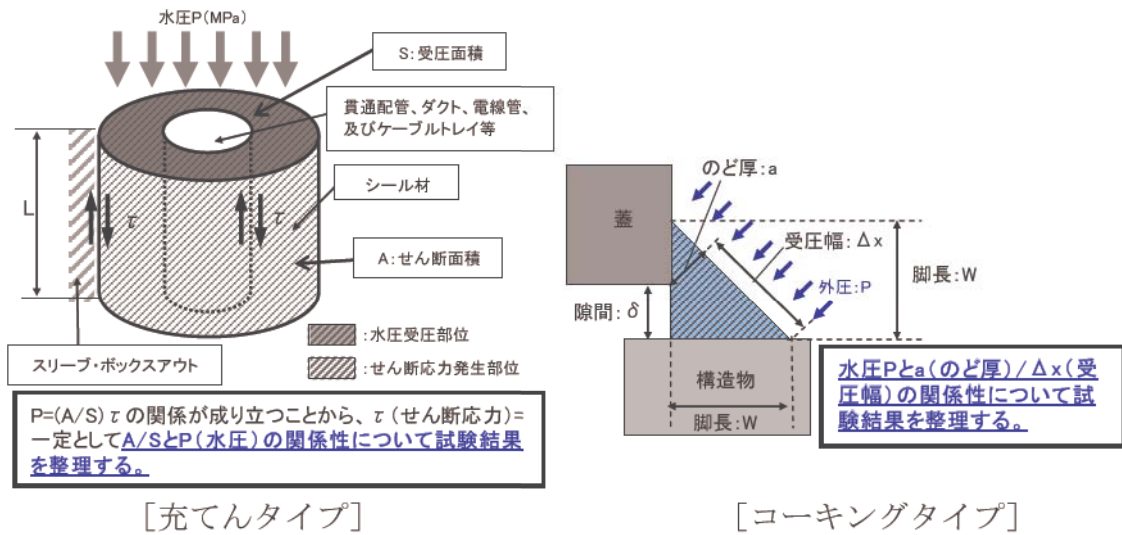
図 4.2-18 試験モデル図
