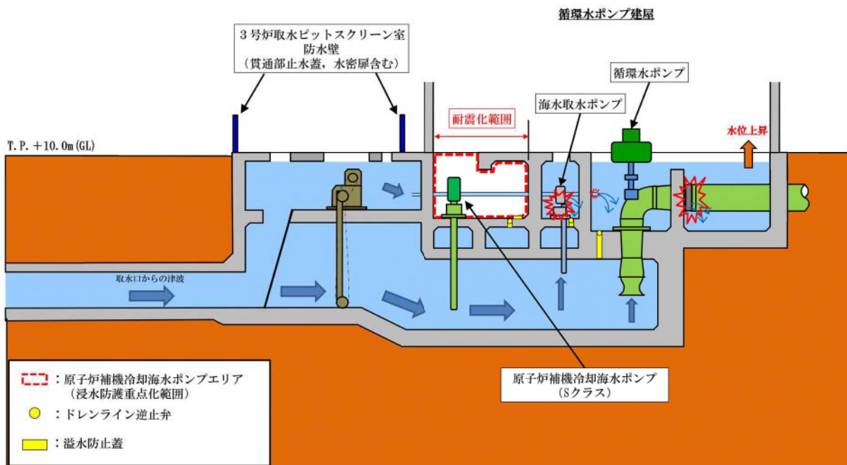
図 3.4-2(1) 地震による溢水の概念図
