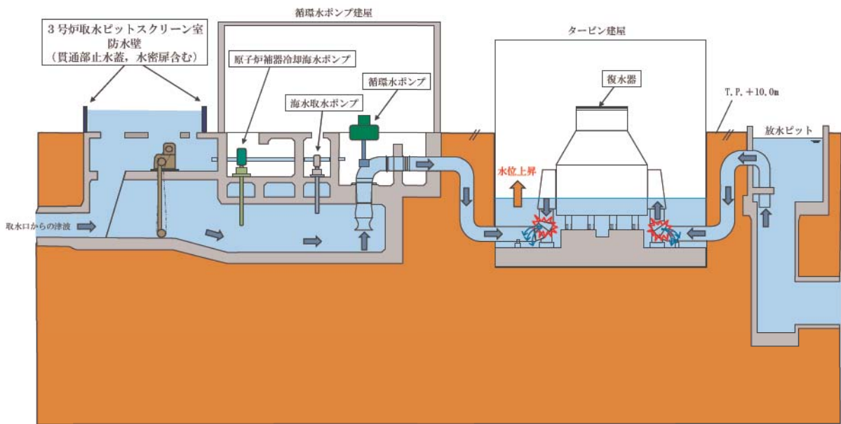
図 3.4-2(2) 地震による溢水の概念図
