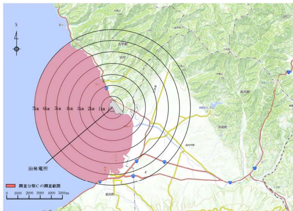
図 2.5-30 海洋設置物（調査分類C）の調査範囲
