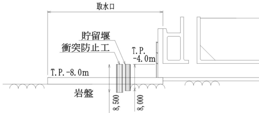
図 4.1-10 貯留堰 構造図
