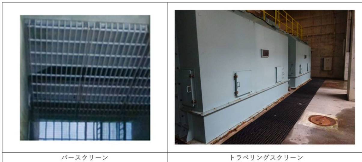
図 2.5-44 除塵設備写真
