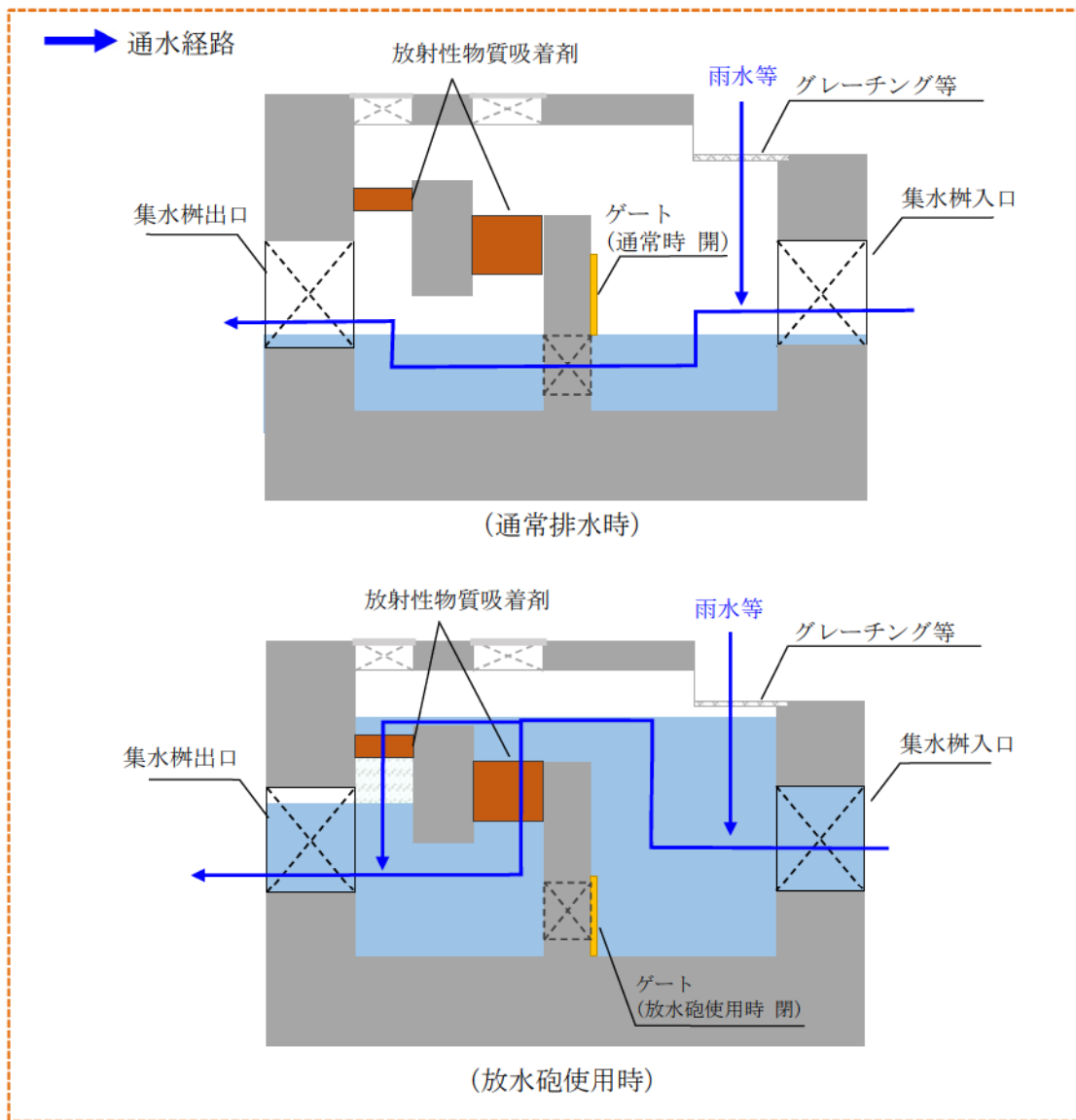
図 3. 4-3 T.P. 10. 0m 盤集水柵内の放射性物質吸着剤の設置位置と通水経路
