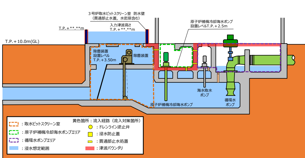
【取水系統断面図（3号炉）】
