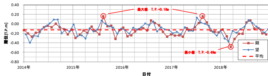
【観測地点岩内港における潮位の推移 (上：満潮位, 下：干潮位)】
