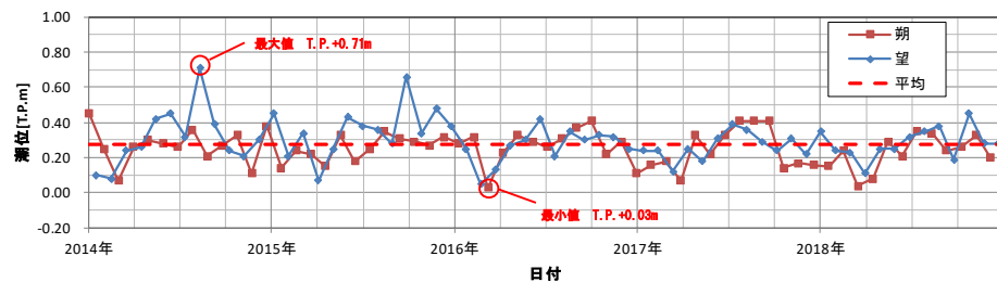
朔望満潮位
