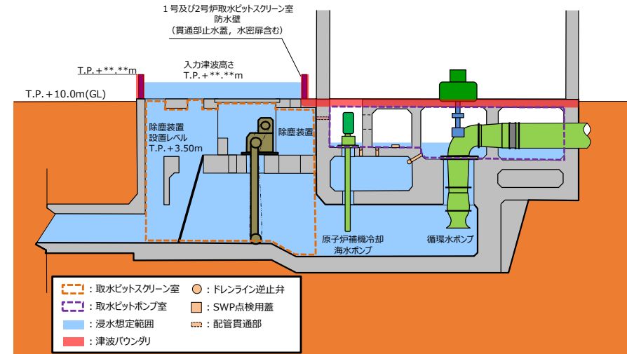
【取水系統断面図（1，2号炉）】
