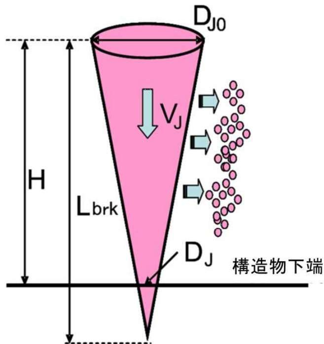
図1 溶融燃料ジェットブレイクアップモデル
