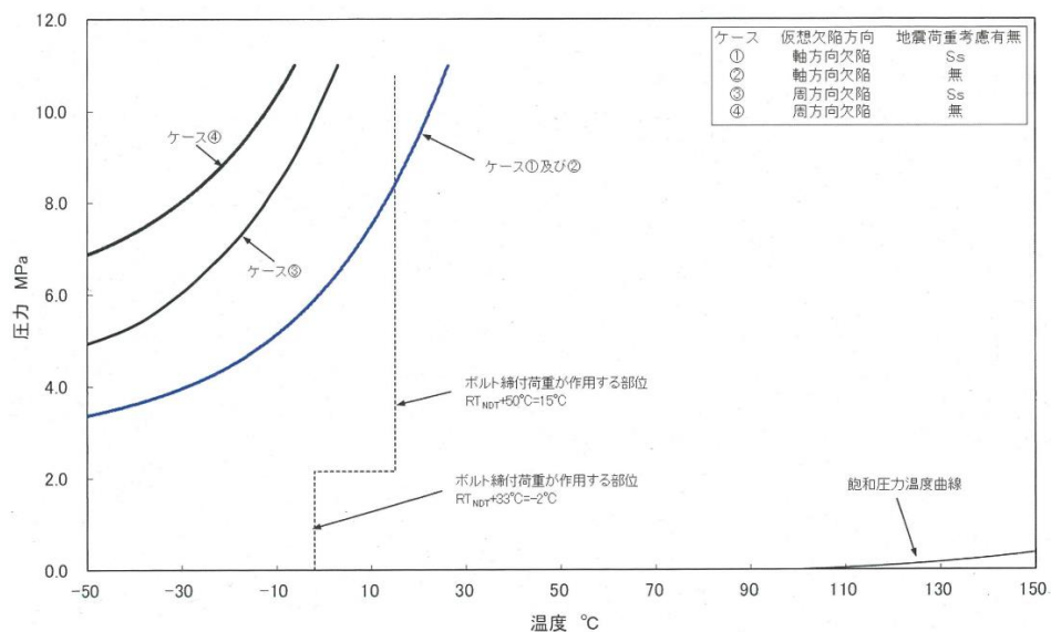
図 5-1 原子炉压力容器の圧力-温度制限図(耐圧試験時)
