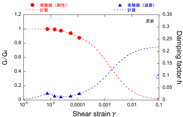
泥岩2
