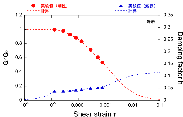
礫岩
