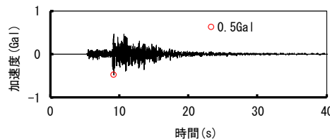
NS方向
