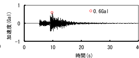
UD方向
