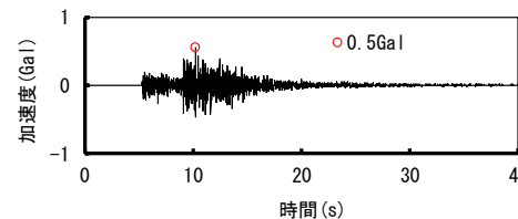
EW方向
