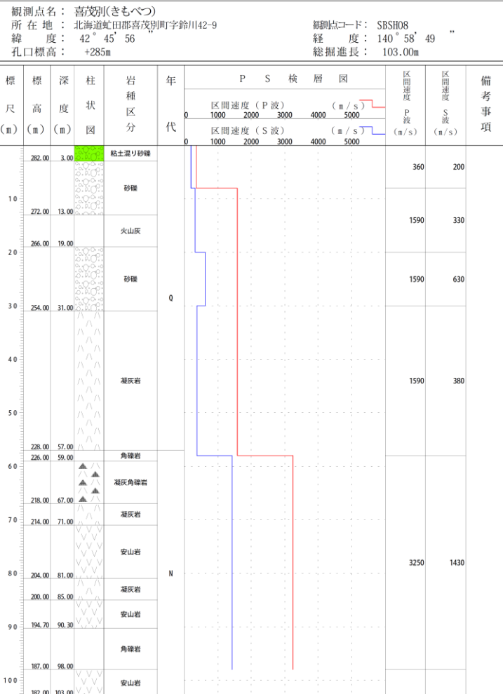
ボーリング柱状図(暫定版)
