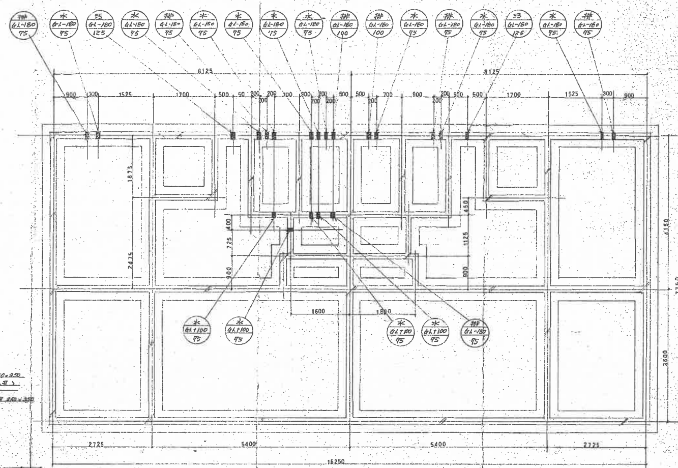
基礎スリーブ参考図 S=1/50
