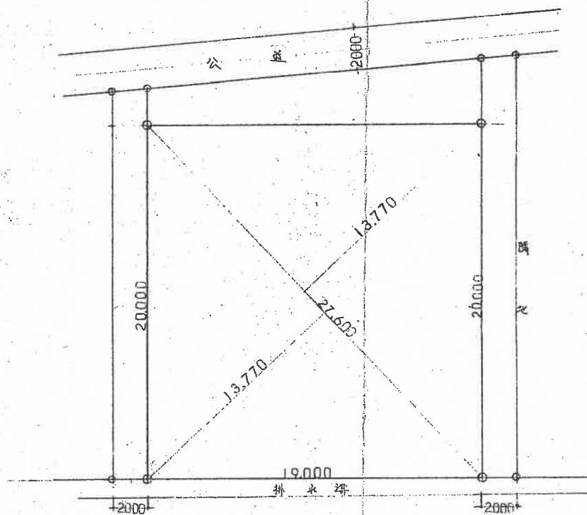
実測図 S: 1/200
