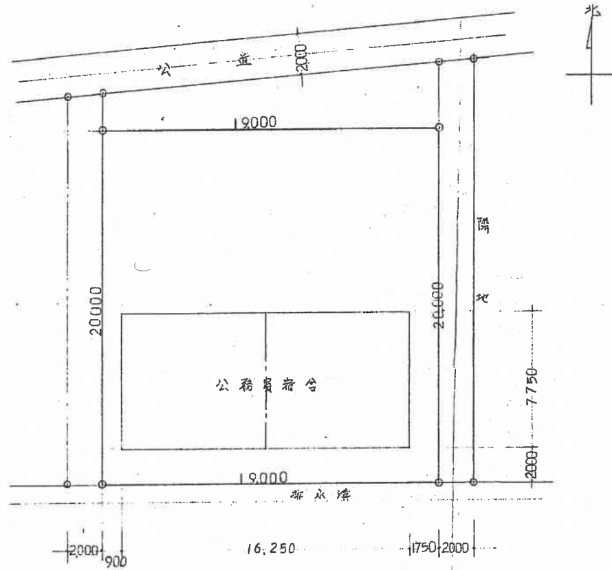
配置図 S: 1/200
