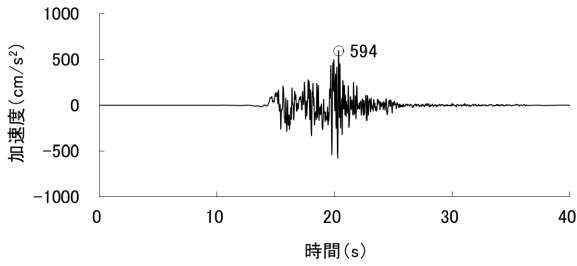
< S s - 1 8 (水平(EW)方向) >
