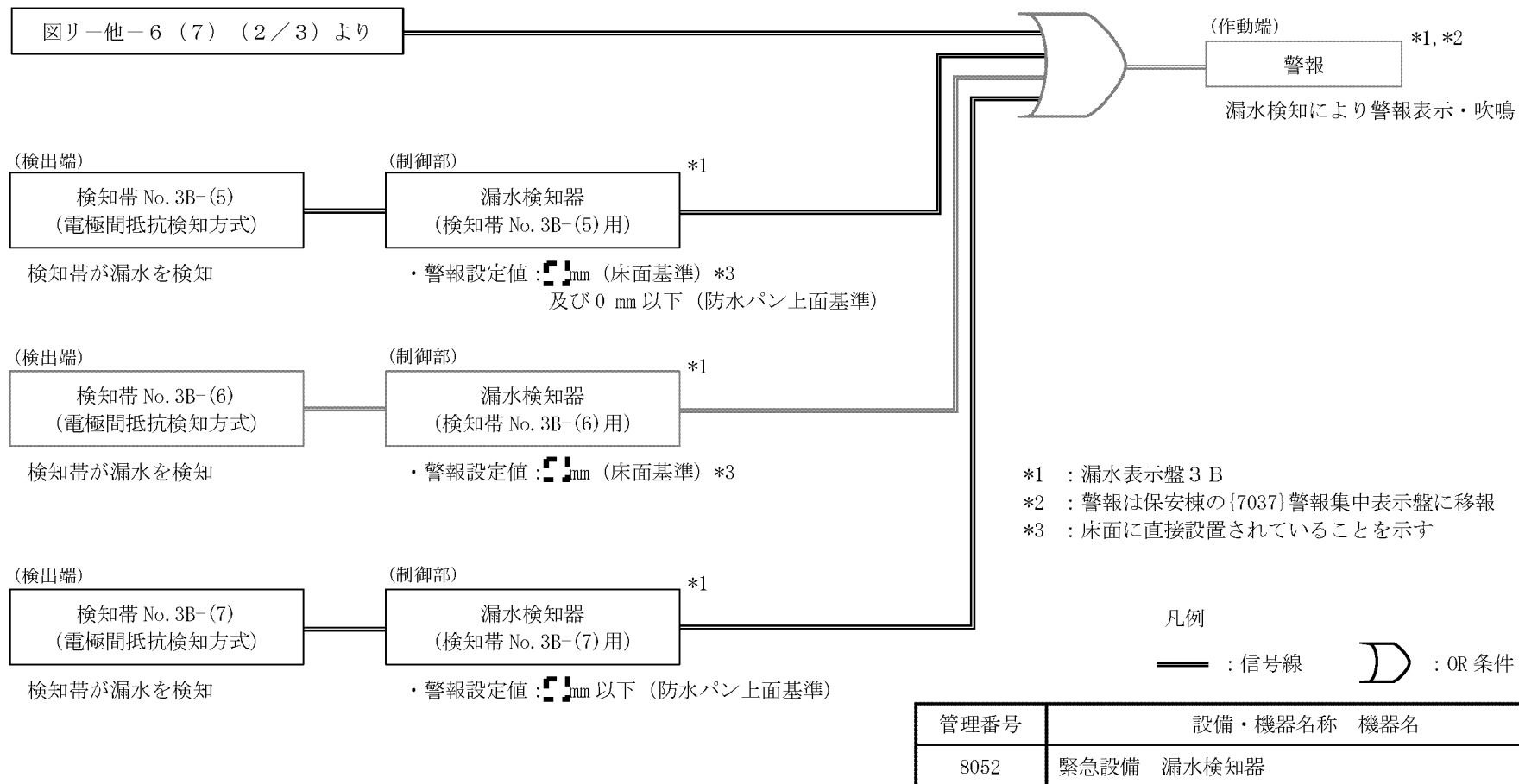
図リ一他ー6 (7) 緊急設備 漏水検知器 第2加工棟 3階 (警報信号系統図) (3/3)
