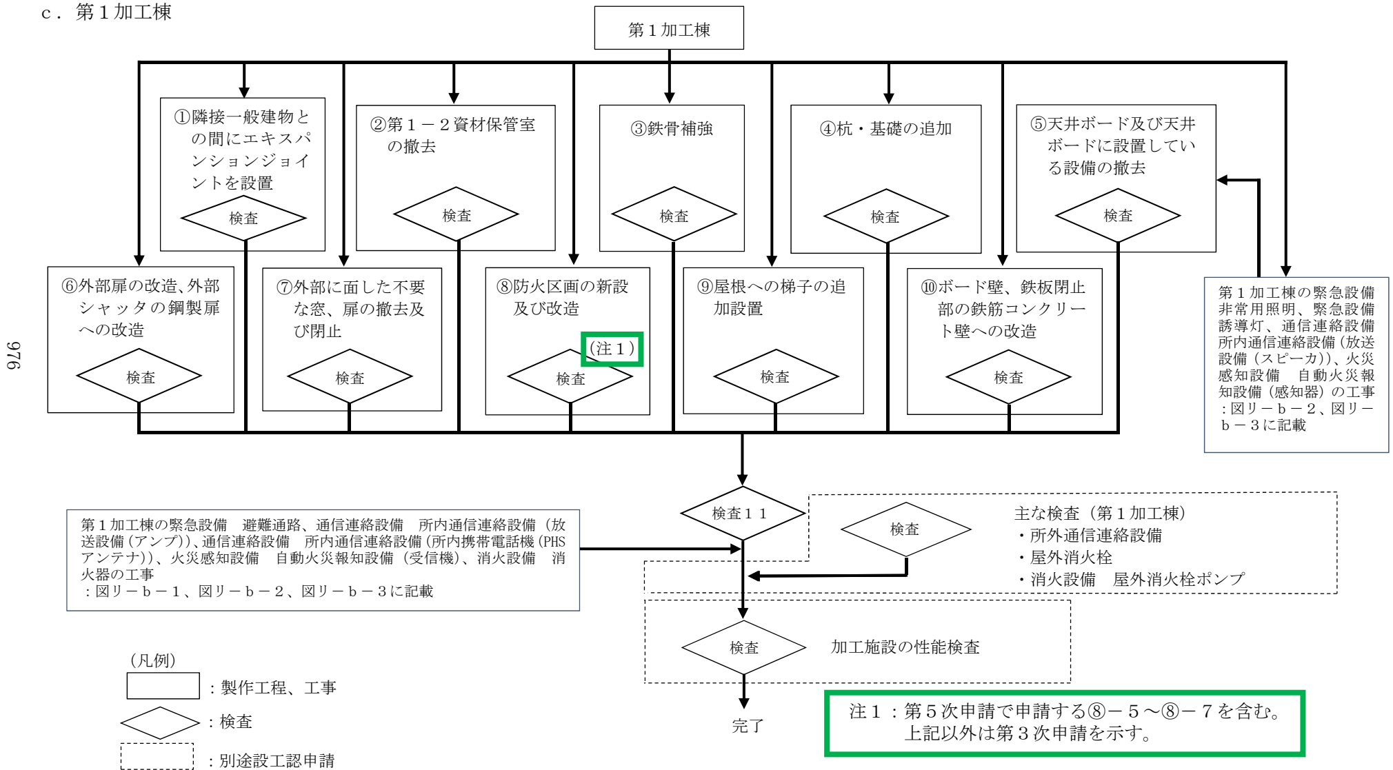
図へ-c-1 第1加工棟 全体工事フロー
