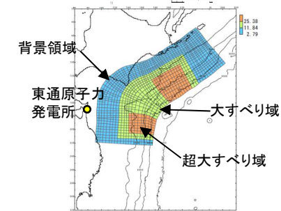
すべり量分布
