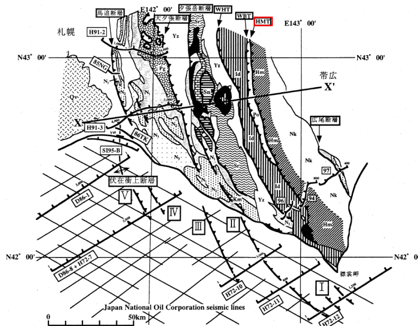
図1 日高衝突帯ならびに前縁褶曲・衝上断層帯の地質概略と主な反射法地震探査測線図。X-X'は図2の断面位置を示す。伊藤ら(1999)を改変。 【地質】主として、地質調査所(1982, 1996)による。Nk:中の川層群, Hm:日高変成岩類(主帯), Po:ボロシリ・オフィオライト(西帯), Id:イドンナップ帯, Yz:蝦夷層群, Sr:空知層群, Km:神威古潭変成岩類, Sn:沙流川層一ニセウ層, Pg:古第三系, N1~N3:地質調査所(1982)と同じ。Qv:第四紀火山岩類。HMT:日高主衝上断層, WBT:西縁衝上断層, WHT:日高西部断層群 【測線】94・96・97:日高深部構造反射法探査, 85NG・86TK:浅野ら(1990), Y97:佐藤ら(1998), その他の測線は石油公団(1973, 1987, 1993, 1996)。
