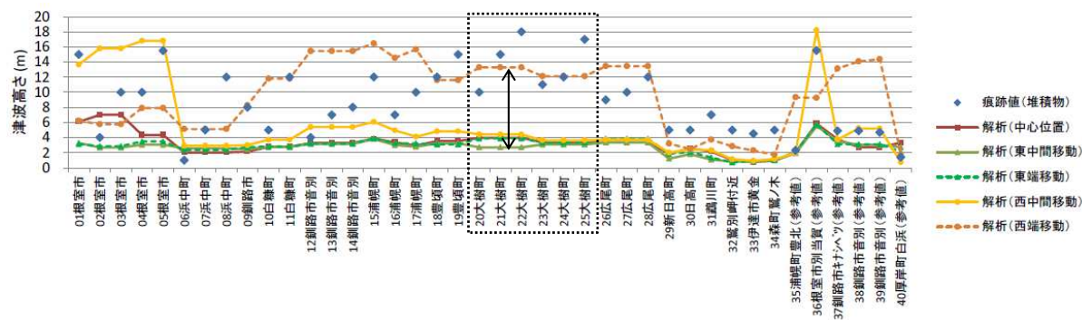
概略パラメータスタディ(大すべり域の位置)による北海道太平洋沿岸での最大津波高さ(土木学会(2016)に一部加筆)
