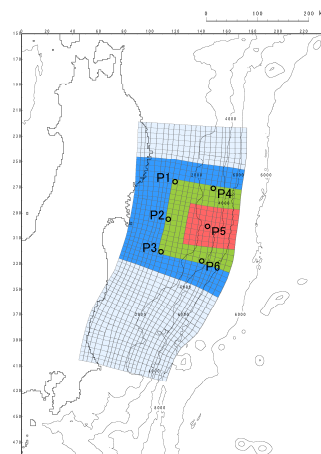
東北地方太平洋沖型の地震 (宮城県沖の大すべり域の破壊 特性を考慮した特性化モデル)
