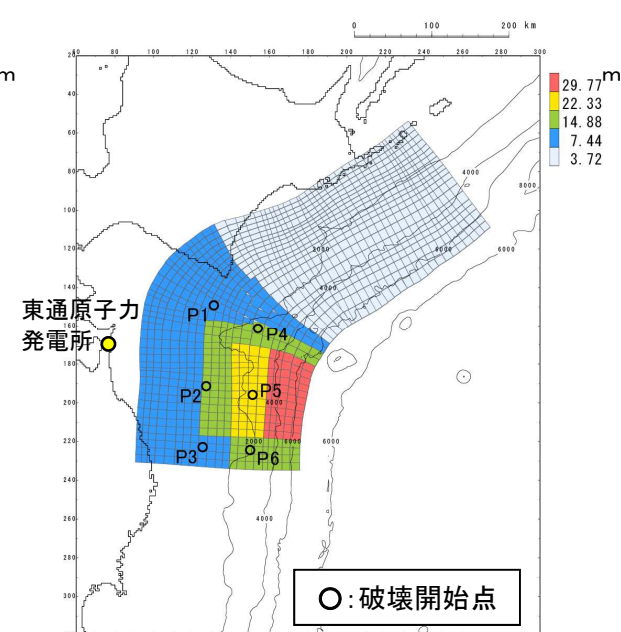
基準断層モデル③
