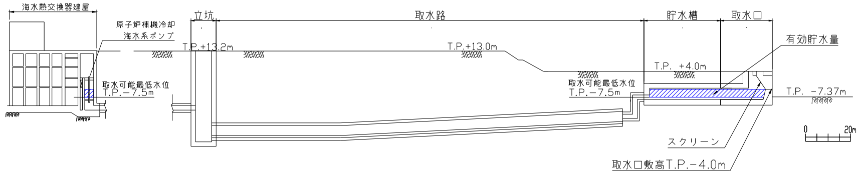
【補機冷却海水系取水設備(断面図)(概要)】
