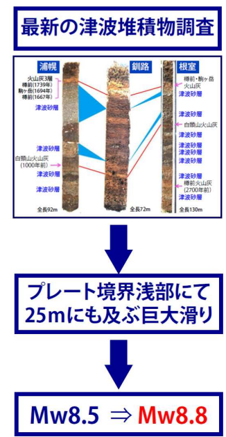
最新の津波堆積物調査から明らかにされた17世紀の地震の断層モデル(文部科学省測地学分科会(2013b))
