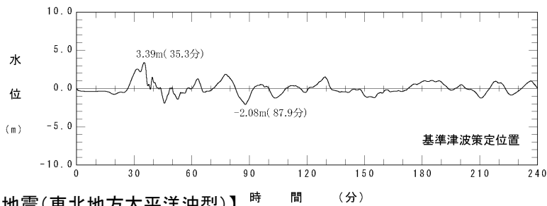
【超巨大地震(東北地方太平洋沖型)】
