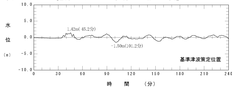
【十勝沖・根室沖から千島前弧スリパー北東端の連動型地震】
