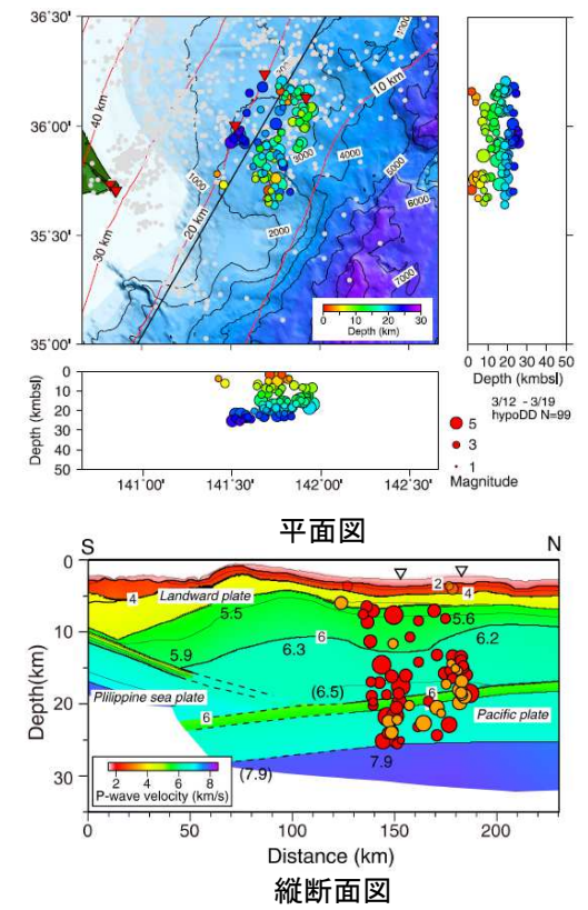
3.11地震の余震分布(3月12日-19日)とプレート境界面の位置関係 (Shinohara et al.(2011))
