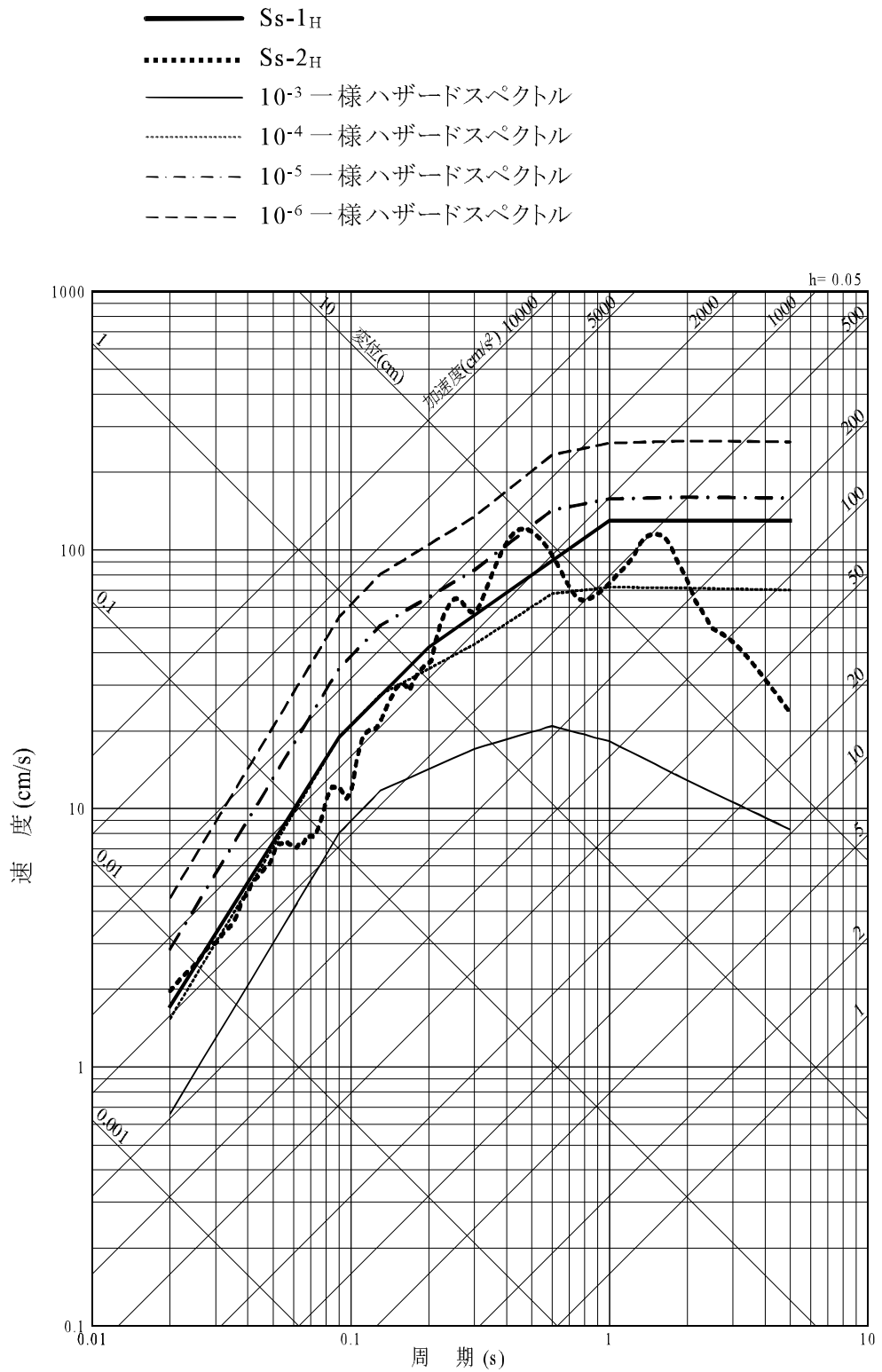
第1.2-316図 基準地震動の応答スペクトル及び解放基盤表面における地震動の一樣ハザードスペクトル(水平方向)
