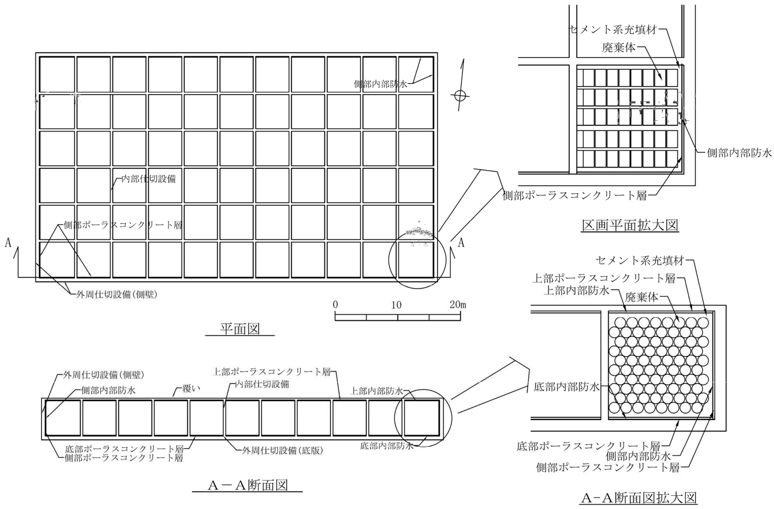
図 1-イ(ロ)-3 内部防水の設置位置図(3号廃棄物埋設地)
