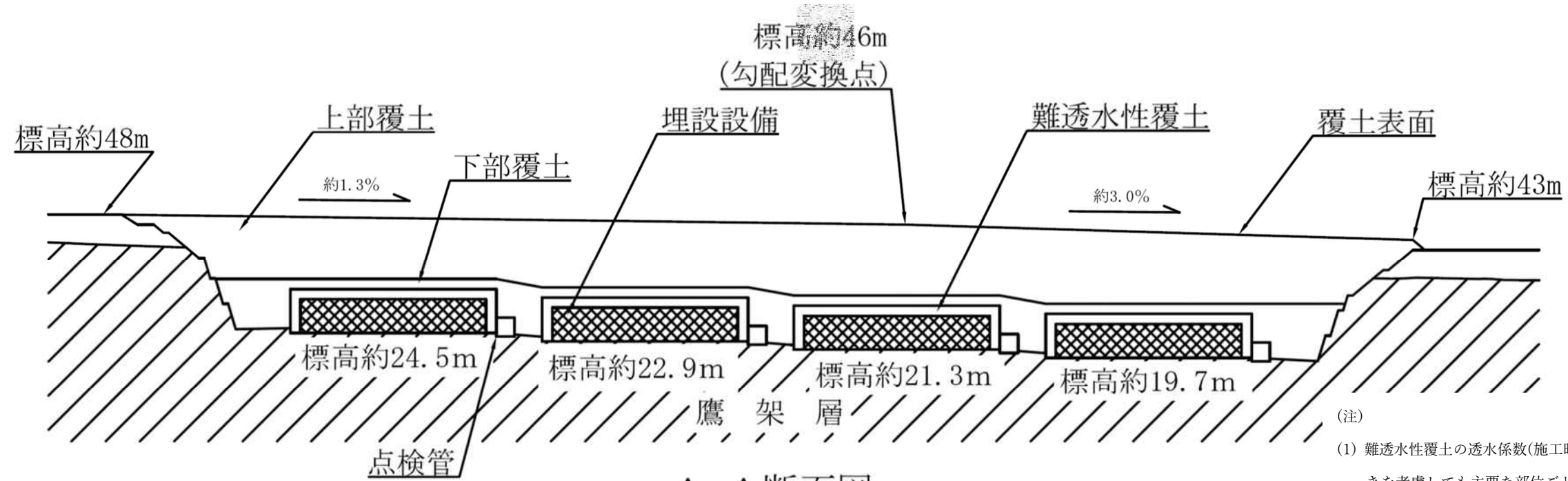
A-A断面図
