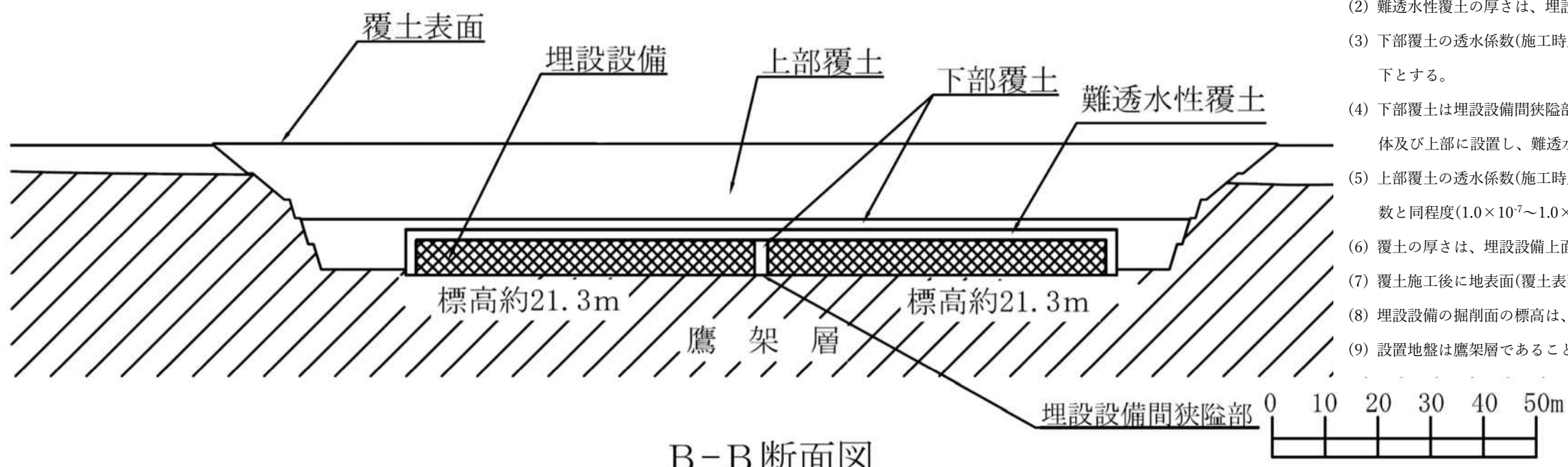
図 1-イ(イ)-2 廃棄物埋設地の設計図(2)
