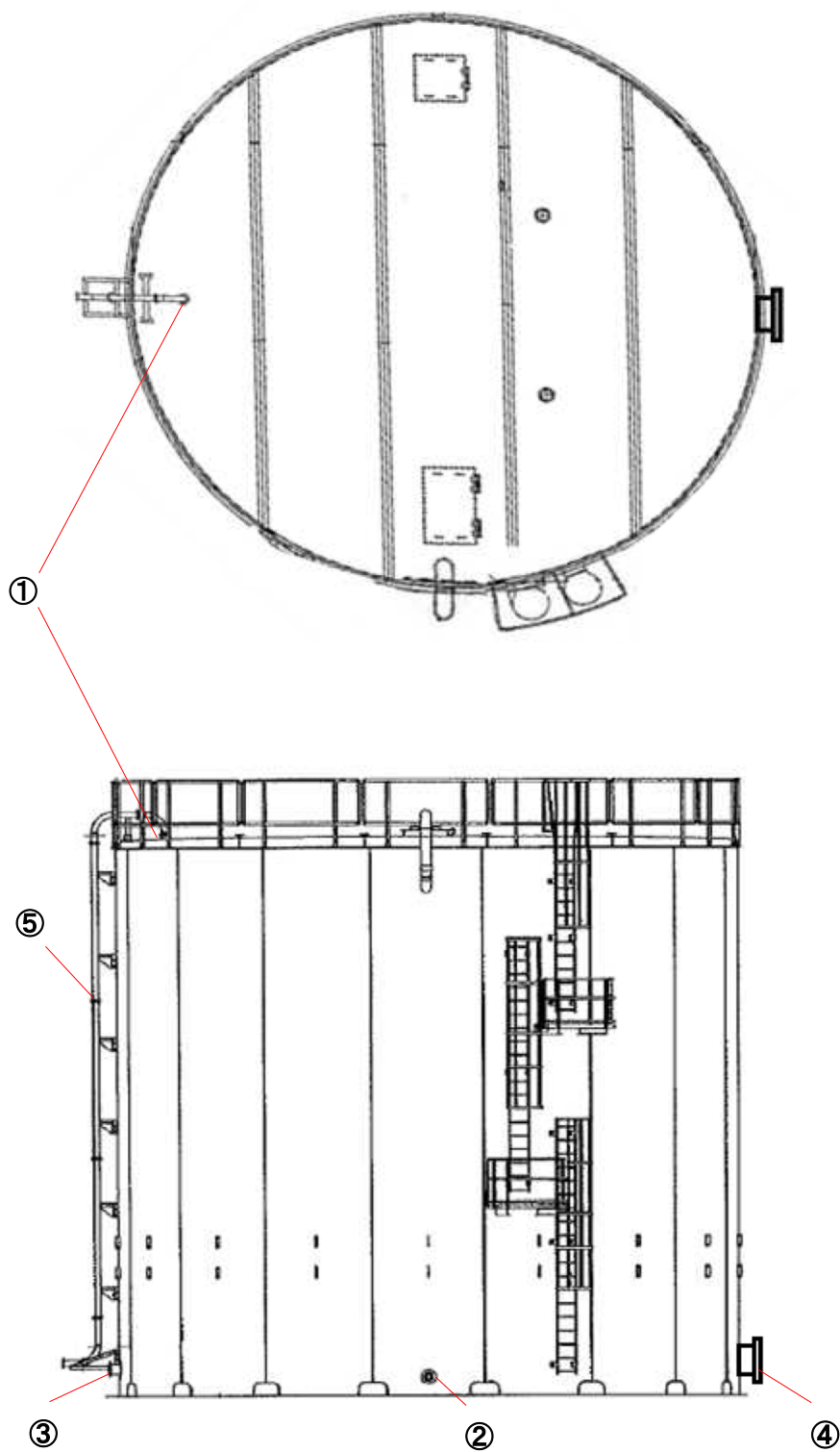
溶接型タンク概略図 (G 4 北) (1, 356m 3 )
